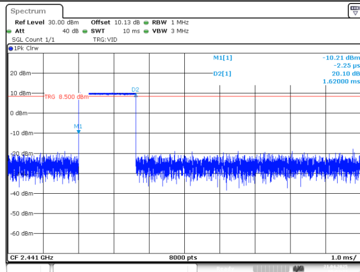
DH3_Ant1_Hop
