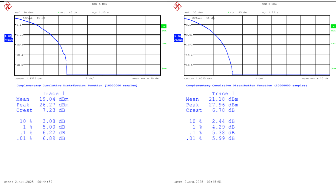
Band2-5MHz-QPSK-18625-1RB#0-PASS
