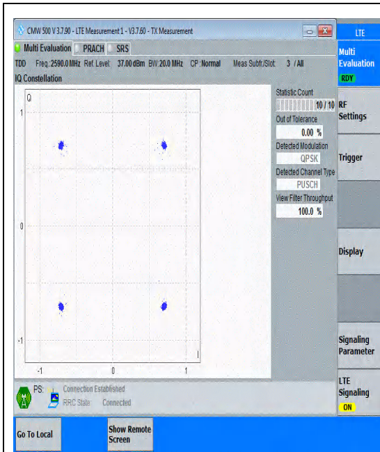
Band41(2535-2655)-20MHz-QPSK-40590-100RB #0-PASS
