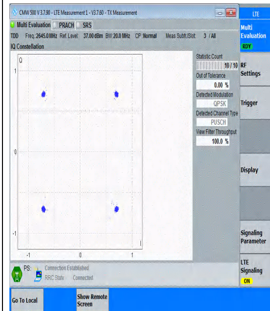
Band41(2535-2655)-20MHz-QPSK-41140-100RB #0-PASS
