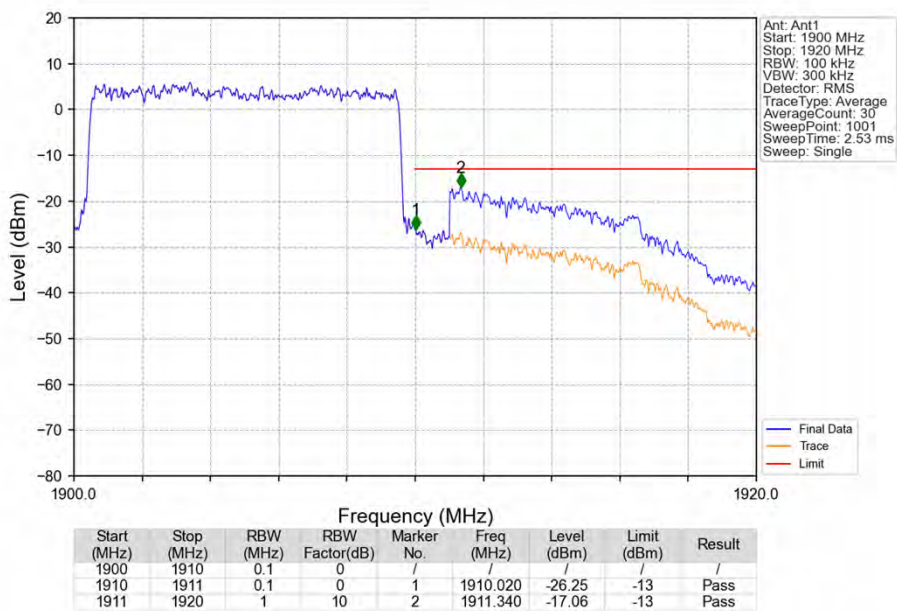
Band2_10MHz_QPSK_HCH_1905MHz_RB_50_0_NTNV
