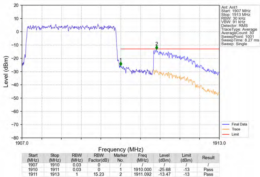
Band2_3MHz_QPSK_HCH_1908.5MHz_RB_15_0_NTNV
