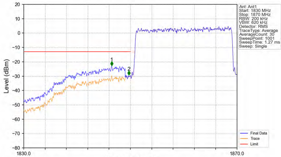
Band2_20MHz_16QAM_LCH_1860MHz_RB_100_0_NTNV
