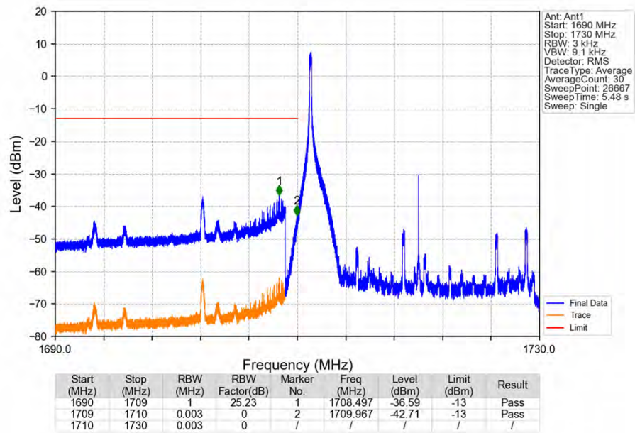
Band4_20MHz_16QAM_LCH_1720MHz_RB_1_0_NTNV
