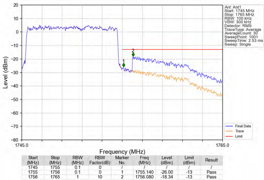
Band4_10MHz_QPSK_HCH_1750MHz_RB_50_0_NTNV
