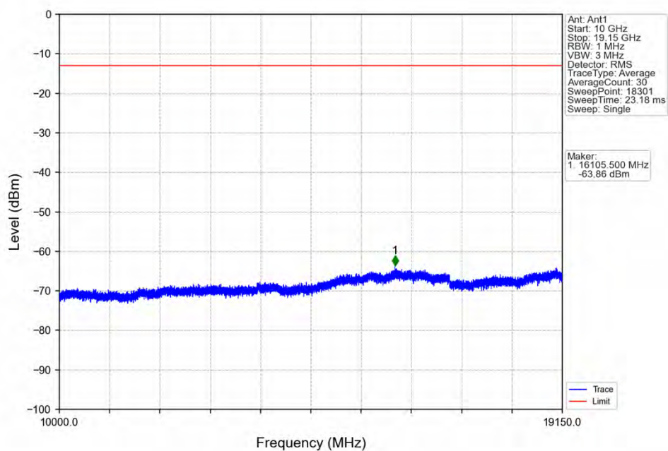
Band25_10MHz_QPSK_LCH_1855MHz_RB_50_0_NTNV
