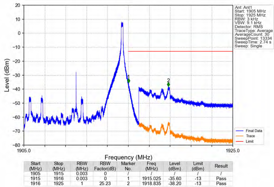
Band25_10MHz_QPSK_HCH_1910MHz_RB_1_49_NTNV
