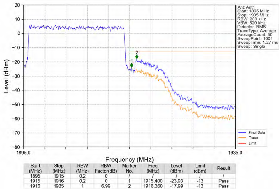
Band25_20MHz_QPSK_HCH_1905MHz_RB_100_0_NTNV
