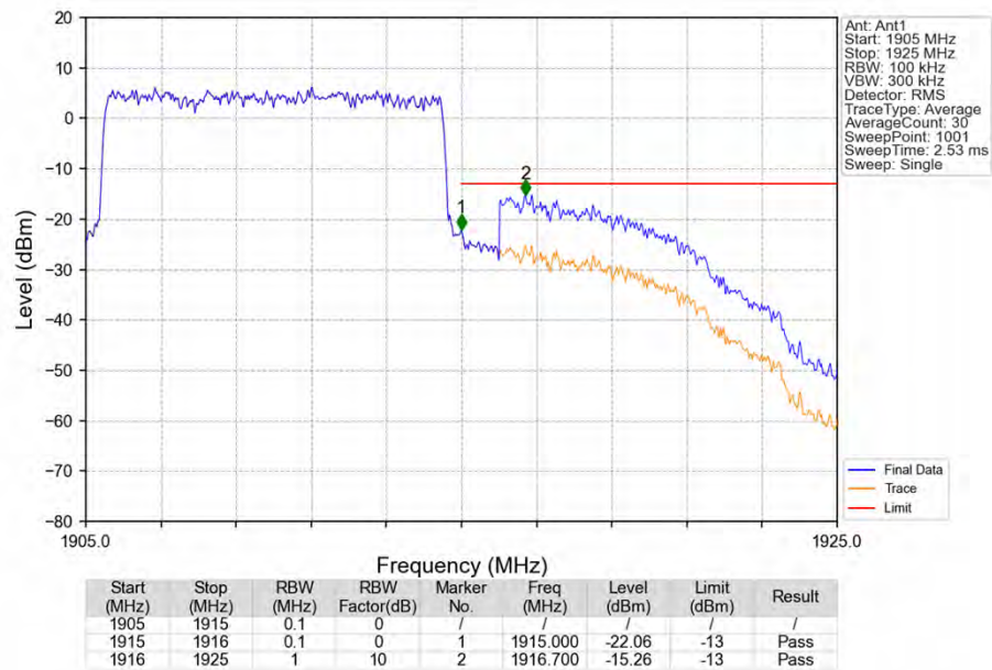
Band25_10MHz_QPSK_HCH_1910MHz_RB_50_0_NTNV
