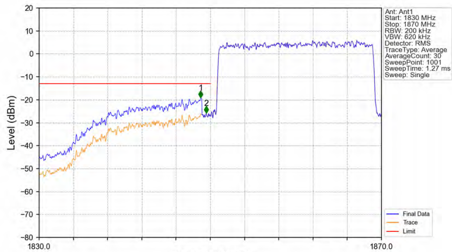
Band25_20MHz_QPSK_LCH_1860MHz_RB_100_0_NTNV
