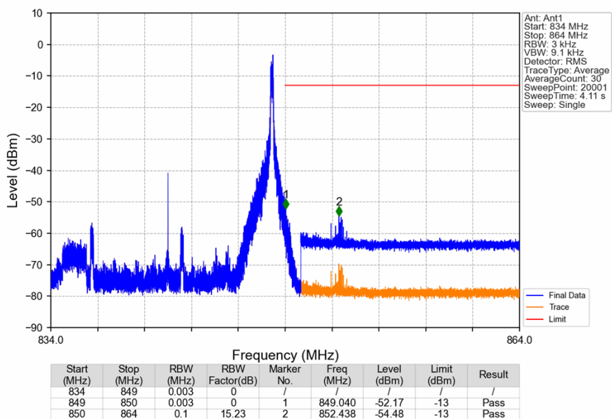
Band26c_15MHz_16QAM_HCH_841.5MHz_RB_1_74_NTNV
