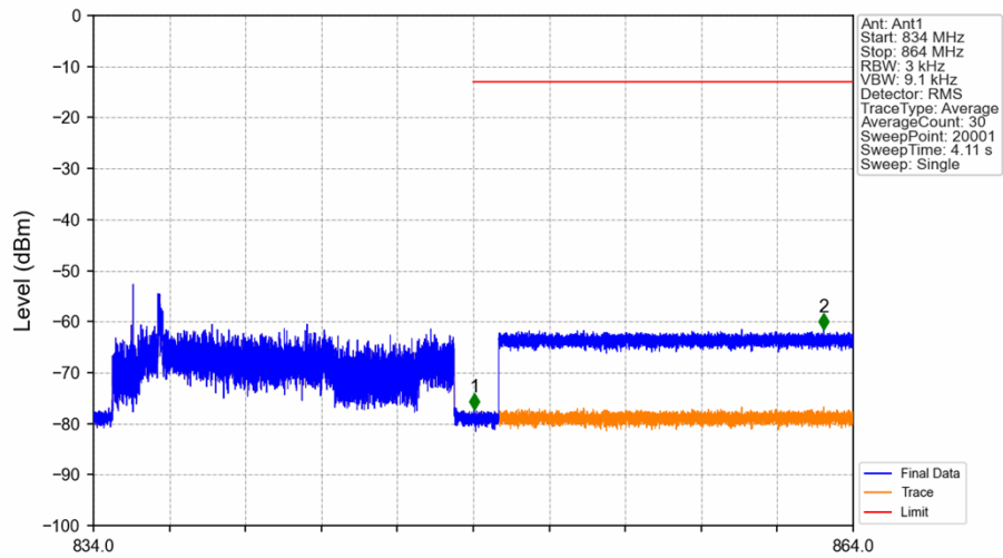
Band26c_15MHz_QPSK_HCH_841.5MHz_RB_1_74_NTNV
