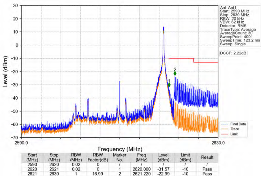
Band38_20MHz_16QAM_HCH_2610MHz_RB_1_99_NTNV
