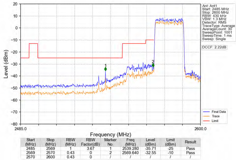
Band38_20MHz_QPSK_LCH_2580MHz_RB_100_0_NTNV
