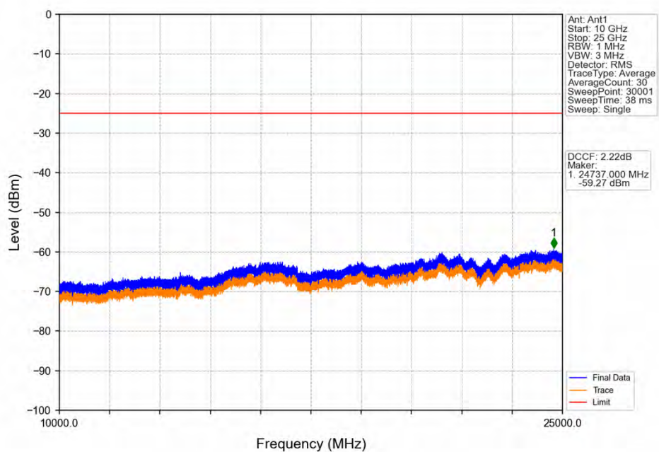
Band38_20MHz_16QAM_HCH_2610MHz_RB_1_0_NTNV
