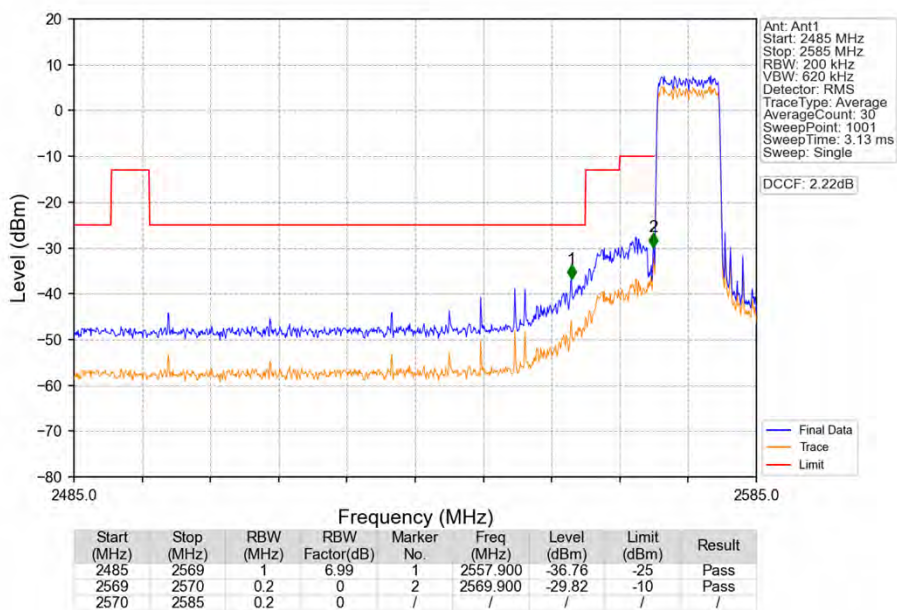
Band38_10MHz_QPSK_LCH_2575MHz_RB_50_0_NTNV
