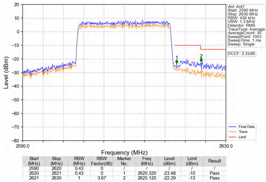
Band38_20MHz_QPSK_HCH_2610MHz_RB_100_0_NTNV
