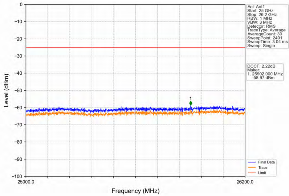
Band38_10MHz_QPSK_HCH_2615MHz_RB_1_49_NTNV
