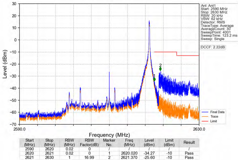
Band38_20MHz_QPSK_HCH_2610MHz_RB_1_99_NTNV
