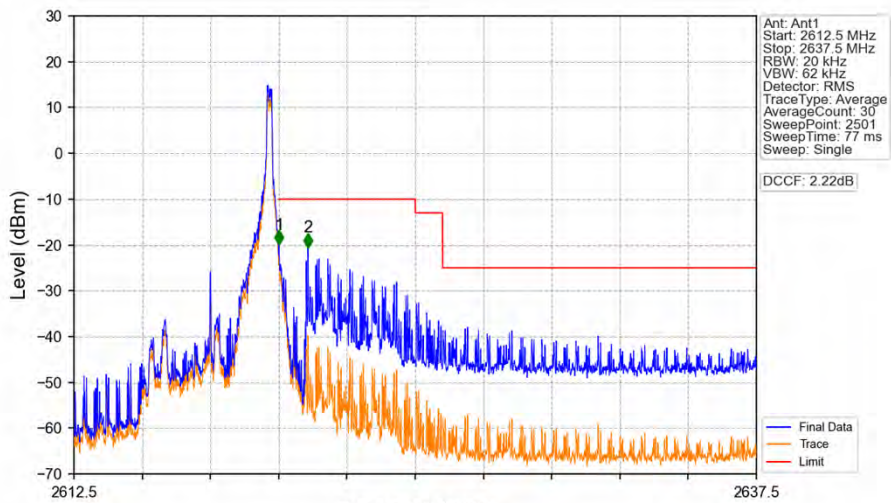
Band38_5MHz_QPSK_HCH_2617.5MHz_RB_1_24_NTNV
