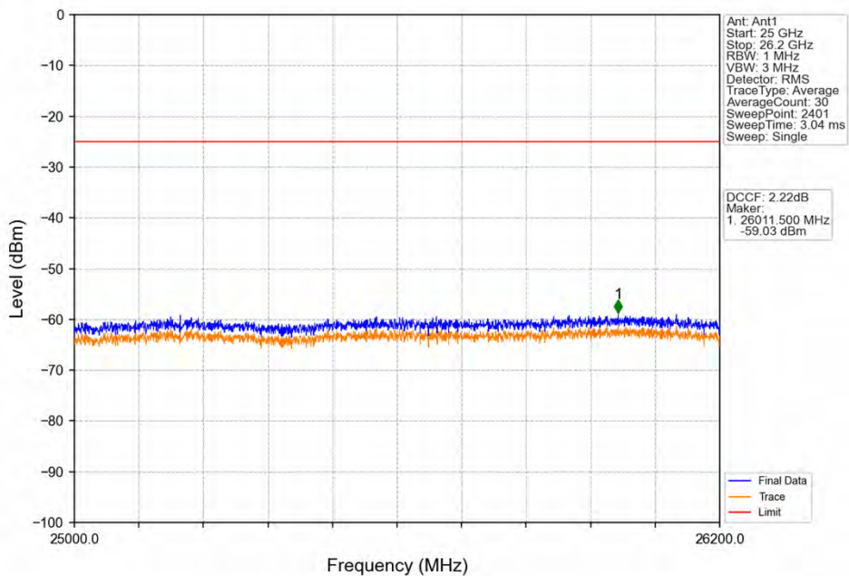
Band38_20MHz_QPSK_HCH_2610MHz_RB_1_99_NTNV
