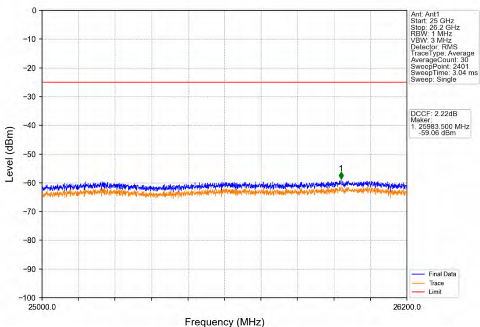
Band38_5MHz_QPSK_HCH_2617.5MHz_RB_1_24_NTNV
