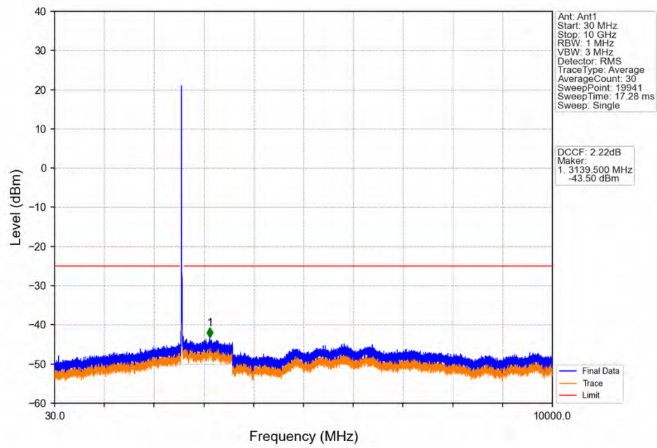
Band38_20MHz_16QAM_LCH_2580MHz_RB_1_0_NTNV
