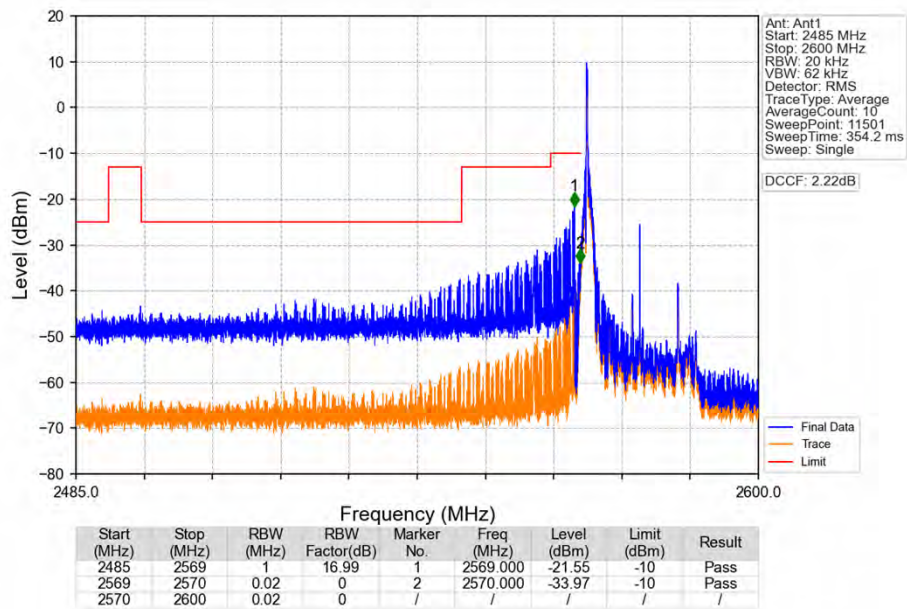
Band38_20MHz_16QAM_LCH_2580MHz_RB_1_0_NTNV
