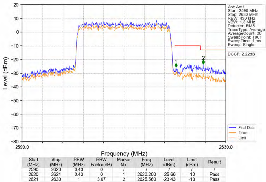
Band38_20MHz_16QAM_HCH_2610MHz_RB_100_0_NTNV
