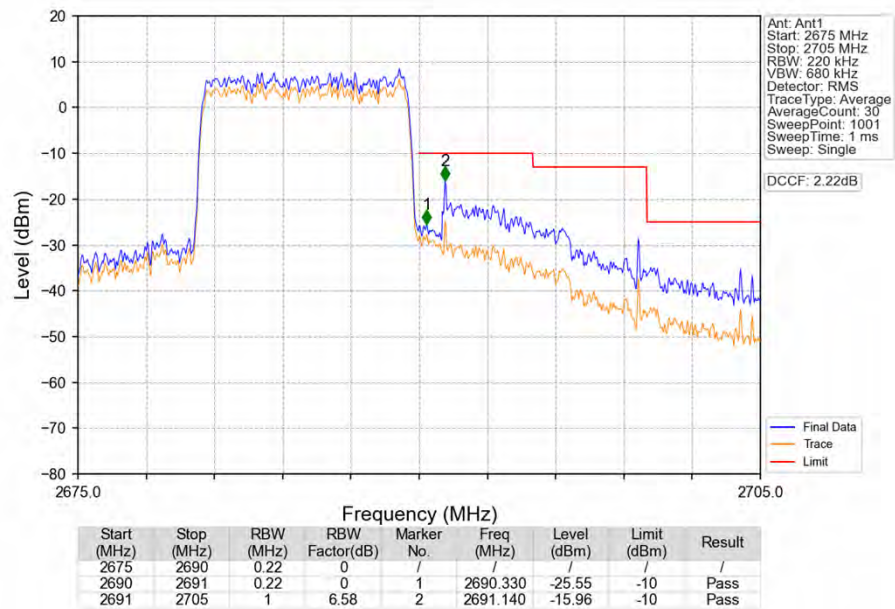
Band41_10MHz_16QAM_HCH_2685MHz_RB_50_0_NTNV
