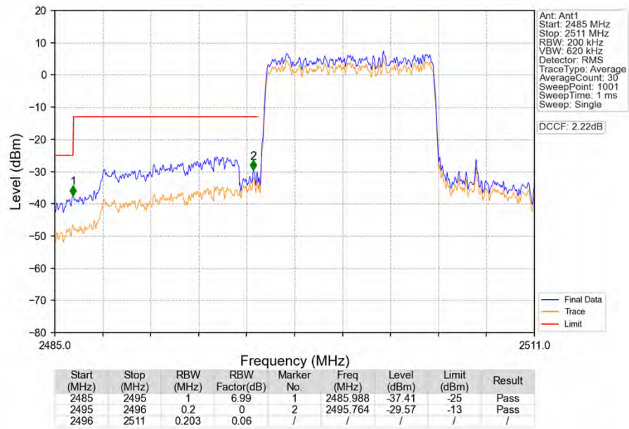
Band41_10MHz_QPSK_LCH_2501MHz_RB_50_0_NTNV
