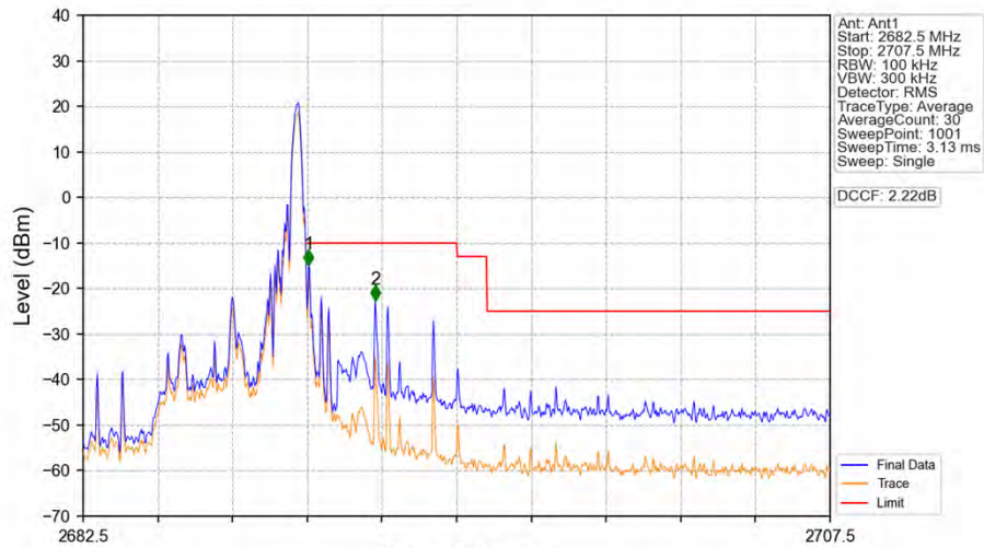
Band41_5MHz_QPSK_HCH_2687.5MHz_RB_1_24_NTNV
