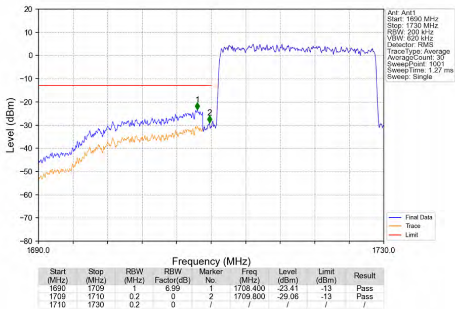
Band66_20MHz_QPSK_LCH_1720MHz_RB_100_0_NTNV
