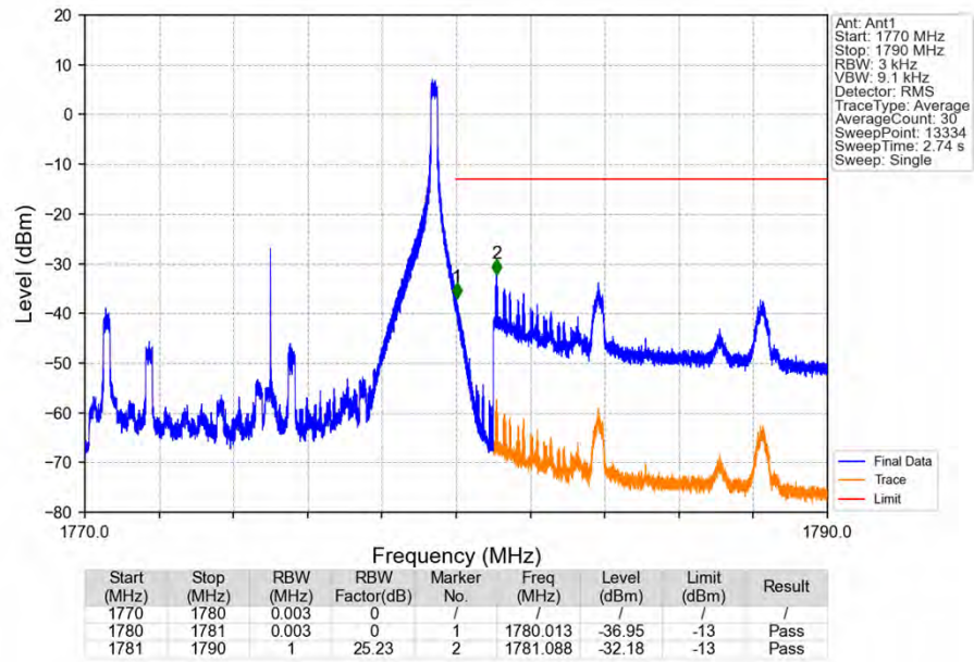
Band66_10MHz_QPSK_HCH_1775MHz_RB_1_49_NTNV
