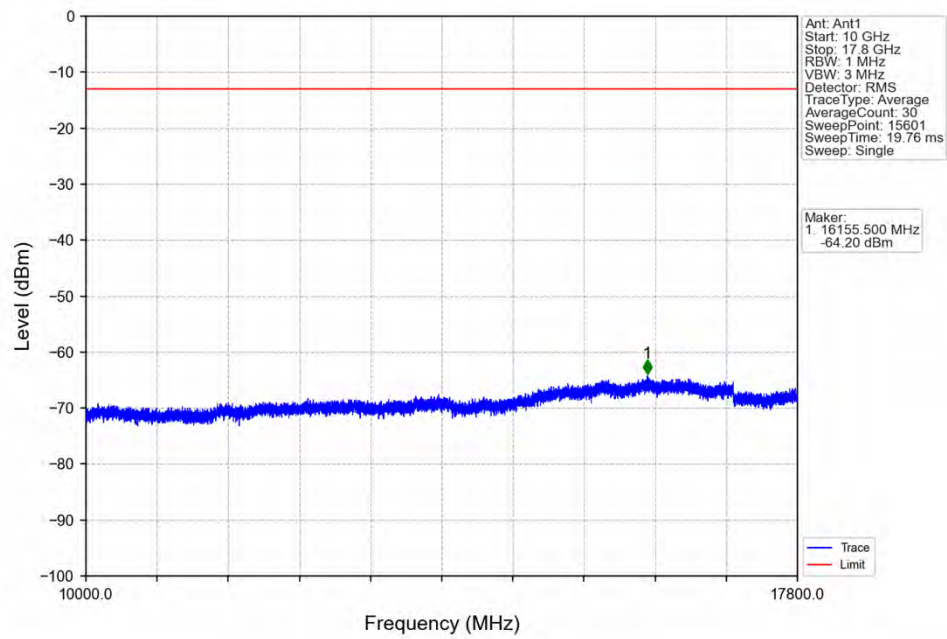
Band66_20MHz_QPSK_MCH_1745MHz_RB_1_0_NTNV
