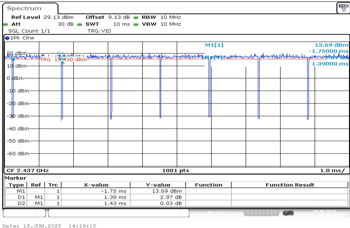
NTNV-11G-Ant1-2437
