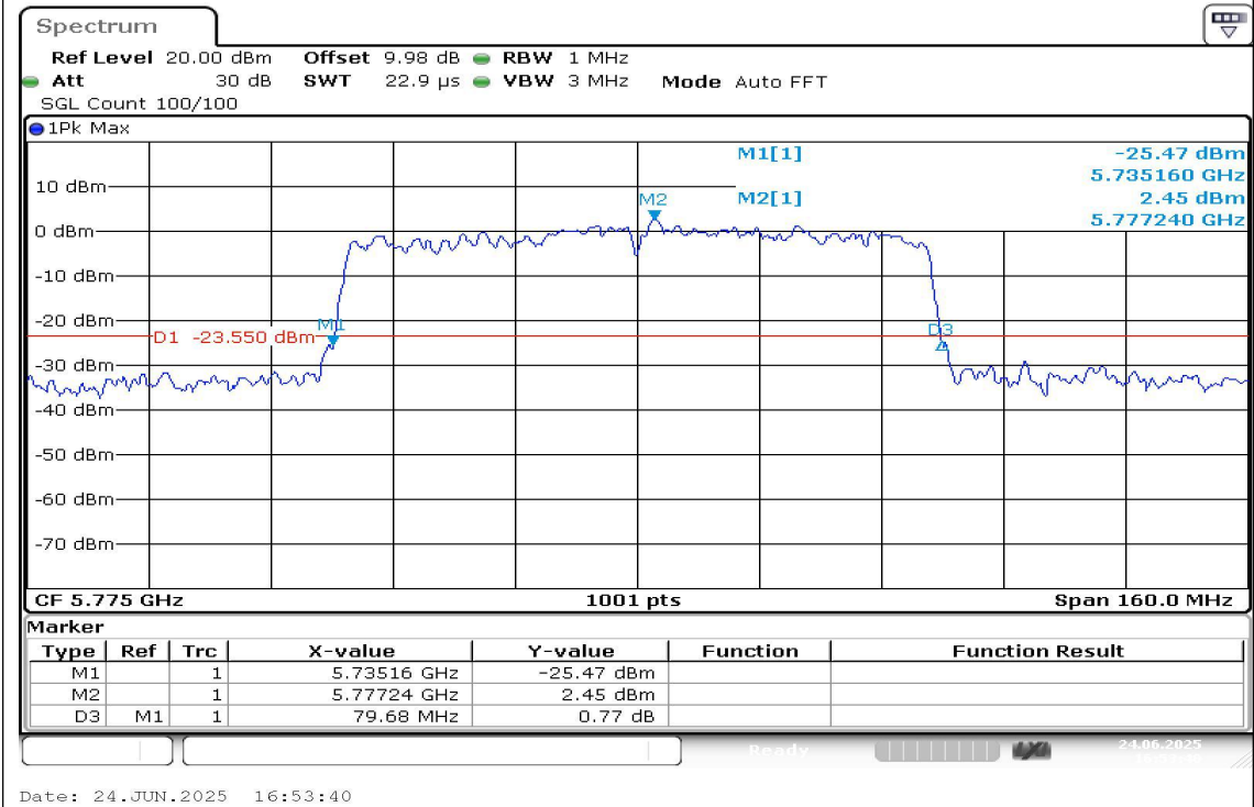
11AC80SISO-Ant1-5775
