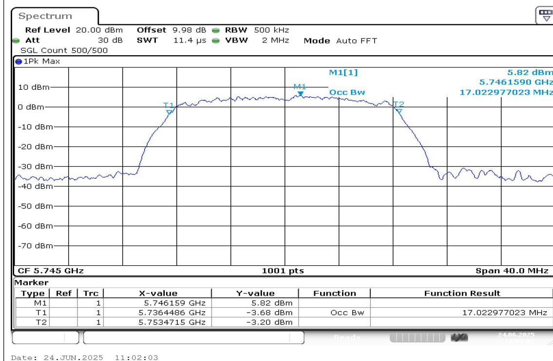
11A-Ant1-5745
