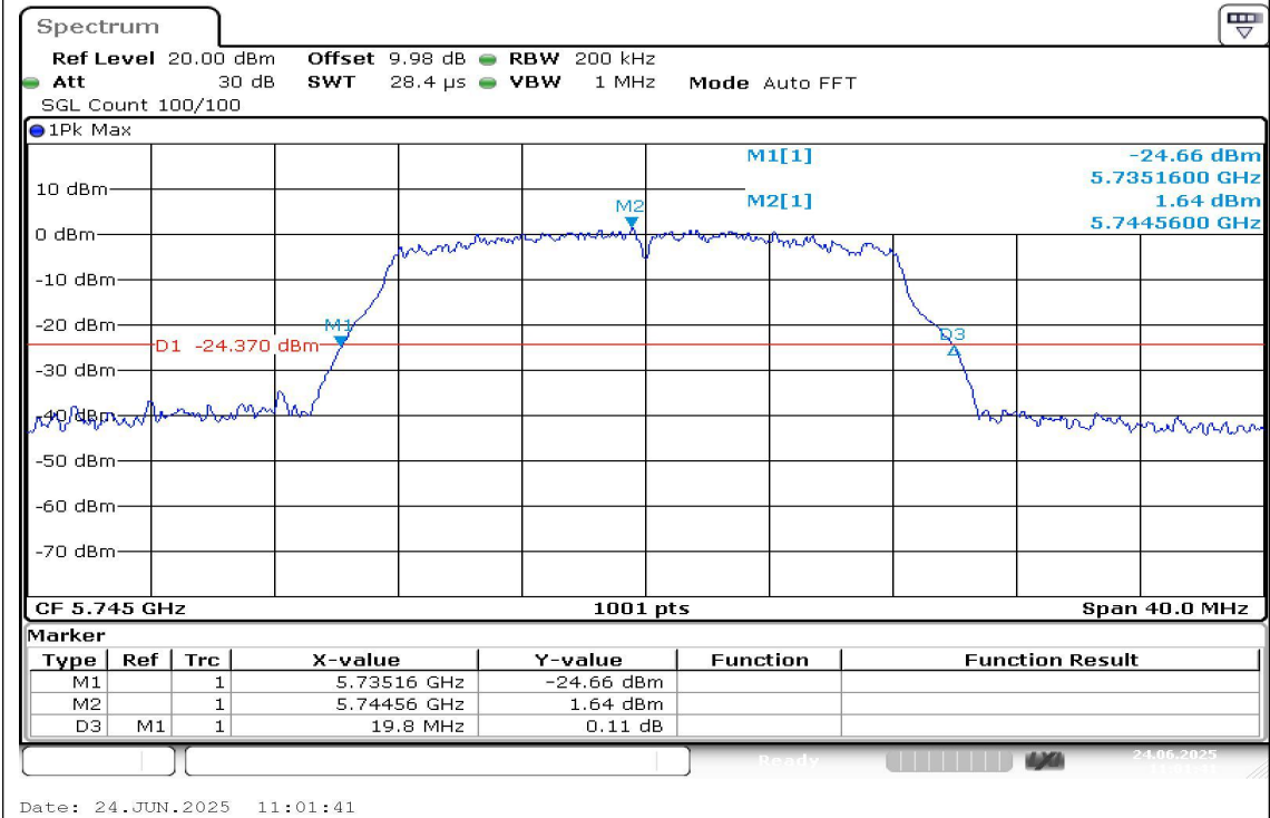
11A-Ant1-5745
