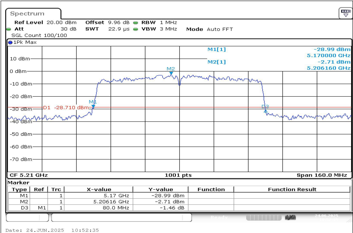
11AC80SISO-Ant1-5210
