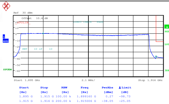
Band25-20MHz-QPSK-26590-1RB#0-PASS
