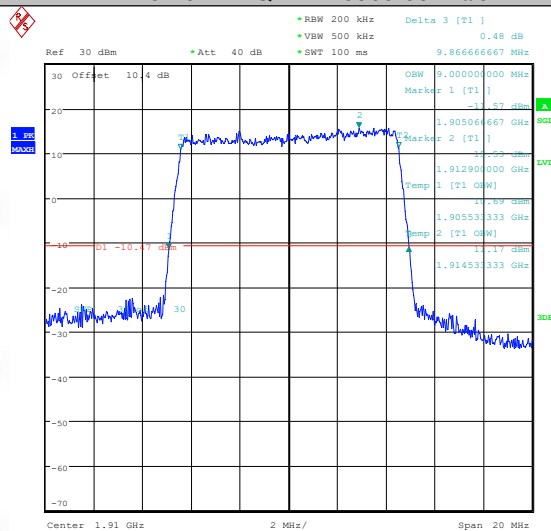
Band25-10MHz-QPSK-26365-50RB#0-PASS
