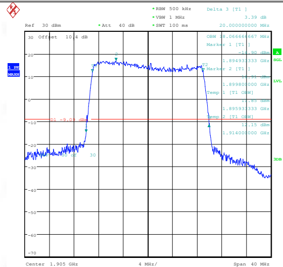
Band25-20MHz-16QAM-26365-100RB#0-PASS
