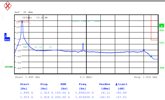
Band25-20MHz-QPSK-26590-1RB#99-PASS
