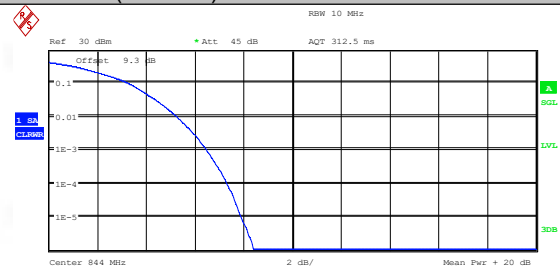
Band26(824-849)-10MHz-QPSK-26990-50RB#0-PASS
