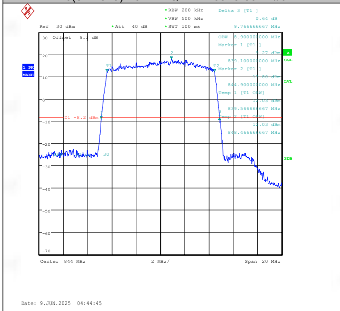
Band26(824-849)-10MHz-QPSK-26990-50RB#0-PASS
