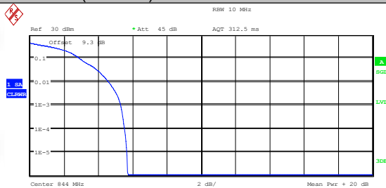
Band26(824-849)-10MHz-QPSK-26990-1RB#0-PASS
