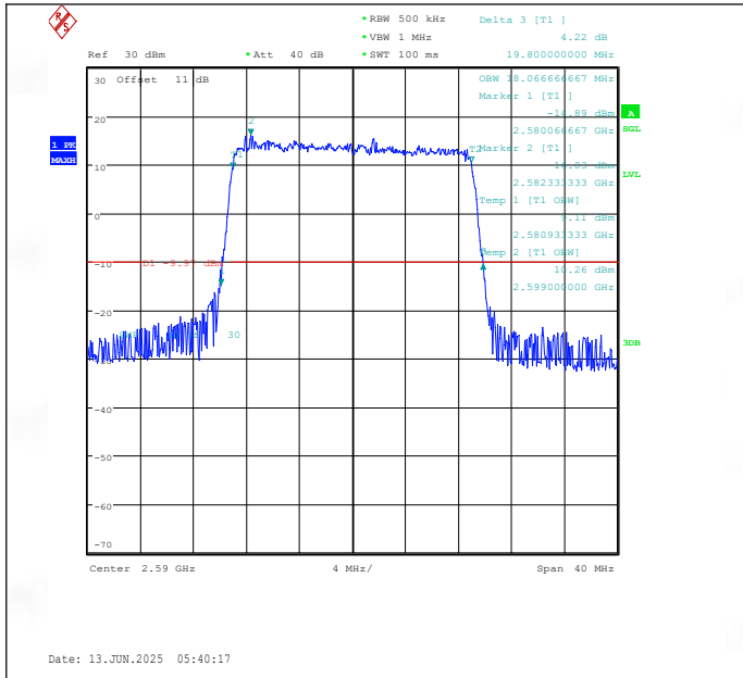
Band41(2535-2655)-20MHz-QPSK-40590-100RB#0-PASS
