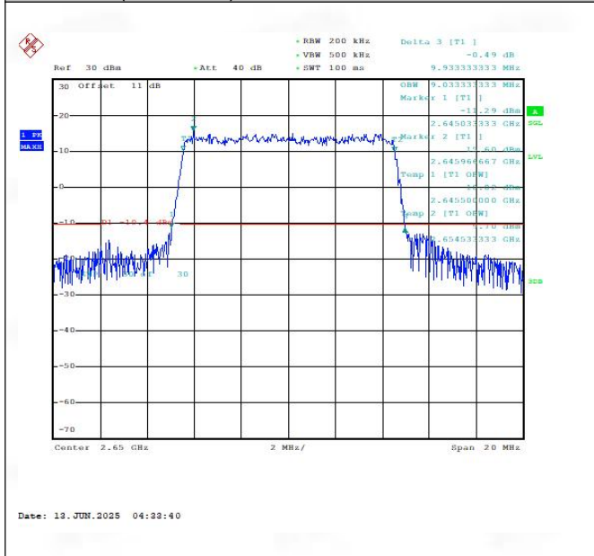
Band41(2535-2655)-10MHz-QPSK-41190-50RB#0-PASS
