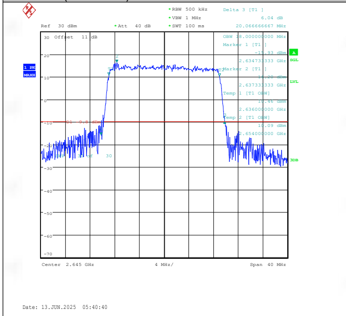
Band41(2535-2655)-20MHz-QPSK-41140-100RB#0-PASS
