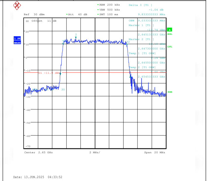
Band41(2535-2655)-10MHz-16QAM-41190-50RB#0-PASS
