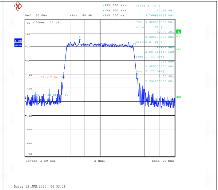
Band41(2535-2655)-10MHz-16QAM-40590-50RB#0-PASS
