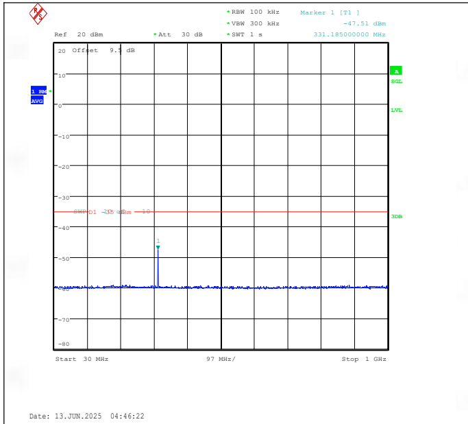
Band41(2535-2655)-10MHz-QPSK-41190-1RB#0-30~1000-PASS
