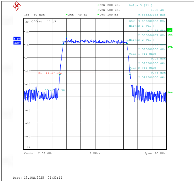
Band41(2535-2655)-10MHz-QPSK-40590-50RB#0-PASS
