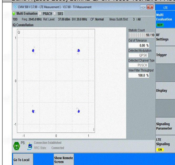
Band41(2535-2655)-20MHz-QPSK-41140-100RB#0-PASS
