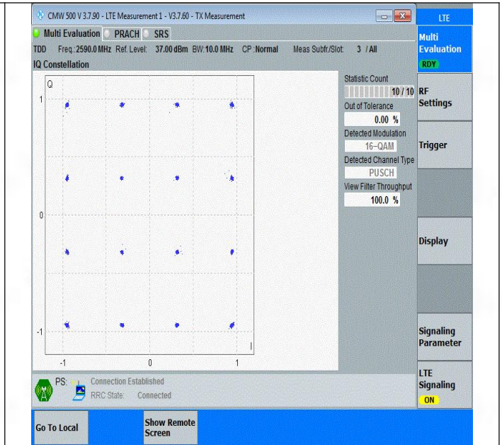
Band41(2535-2655)-10MHz-16QAM-40590-50RB#0-PASS
