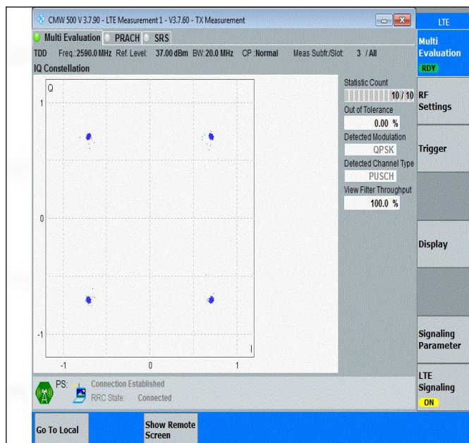
Band41(2535-2655)-20MHz-QPSK-40590-100RB#0-PASS
