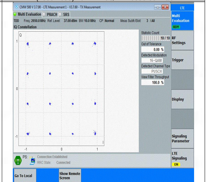
Band41(2535-2655)-10MHz-16QAM-41190-50RB#0-PASS
