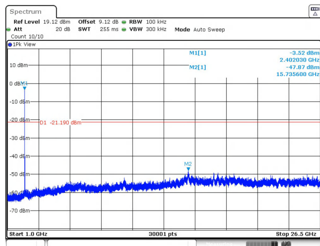
BLE_2M_Ant1_2402_1000~26500
