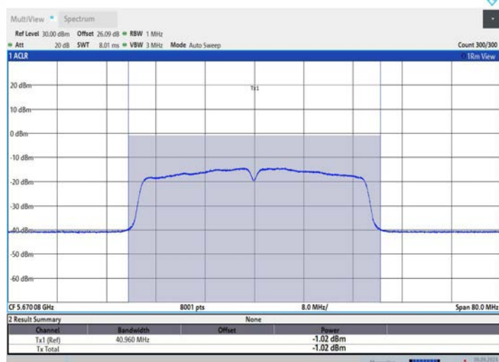
11AC40MIMO_Ant2_5670
