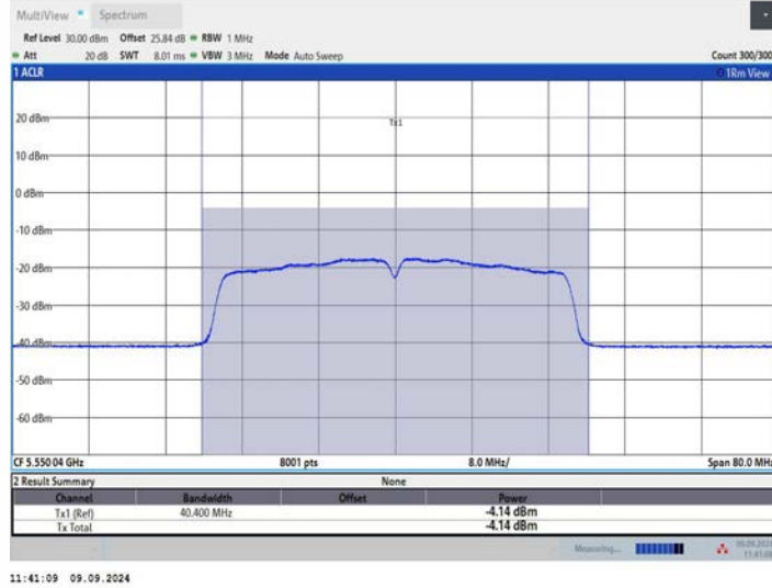
11AC40MIMO_Ant2_5550
