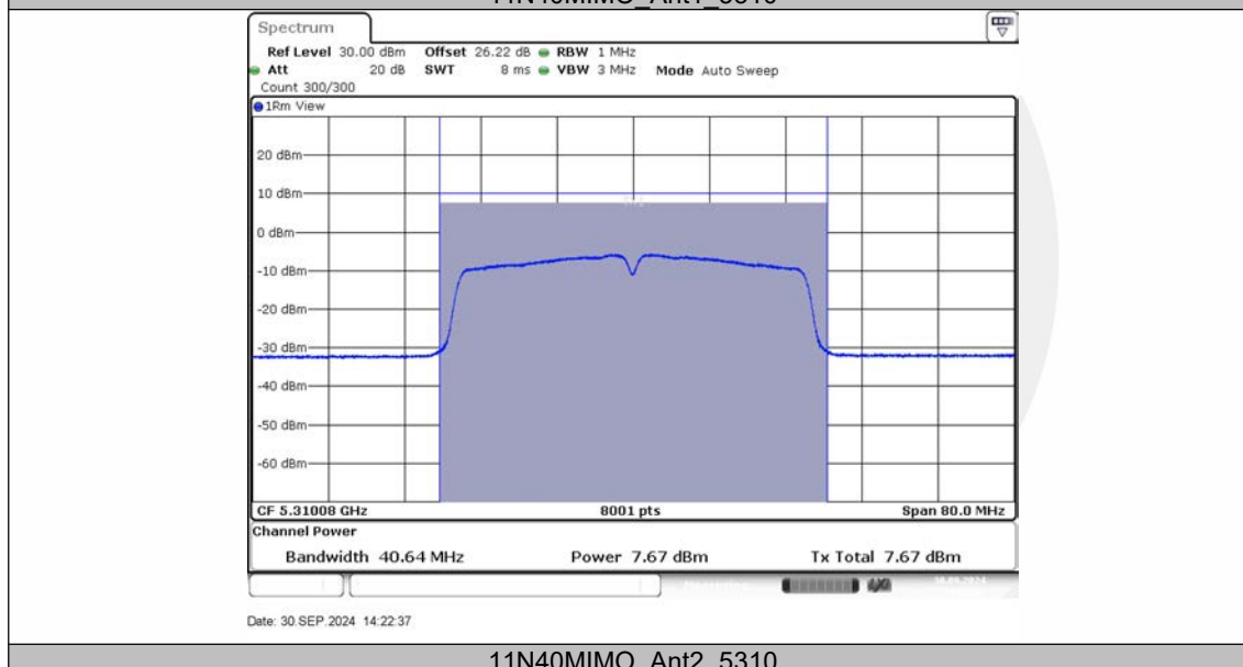
11N40MIMO_Ant2_5310
