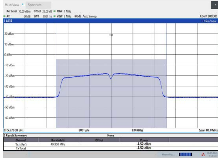
11AC40MIMO_Ant1_5670
