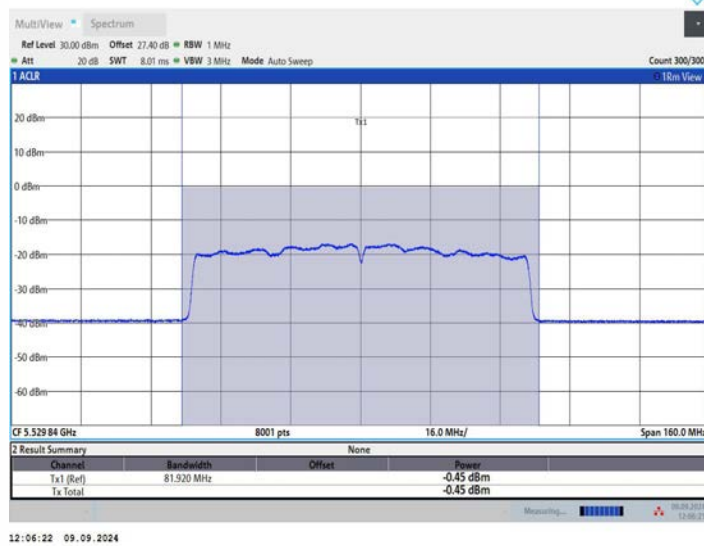
11AC80MIMO_Ant2_5530
