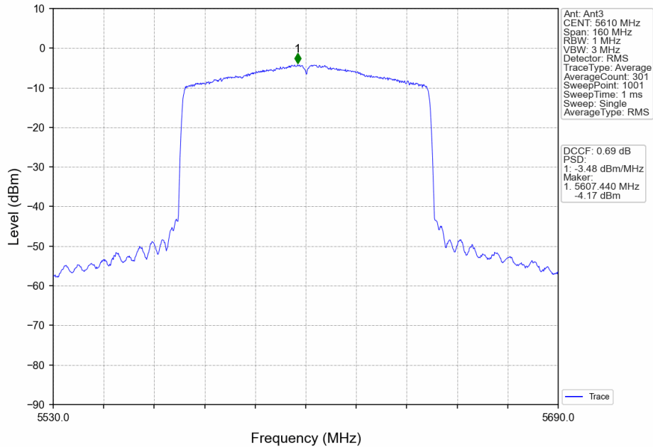
802.11ac(VHT80)_HCH_5610MHz_MIMO_NTNV
