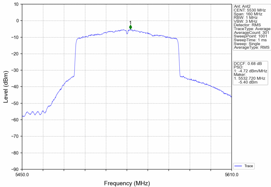
802.11ac(VHT80)_LCH_5530MHz_Ant2_NTNV
