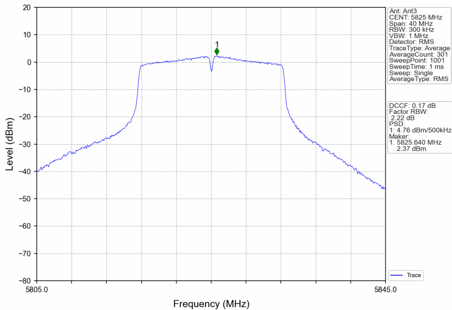
802.11a_HCH_5825MHz_MIMO_NTNV
