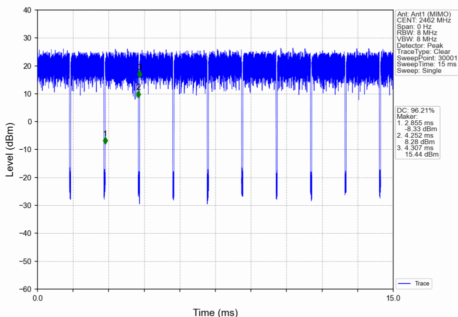
802.11g_HCH_2462MHz_Ant1 (MIMO)_NTNV
