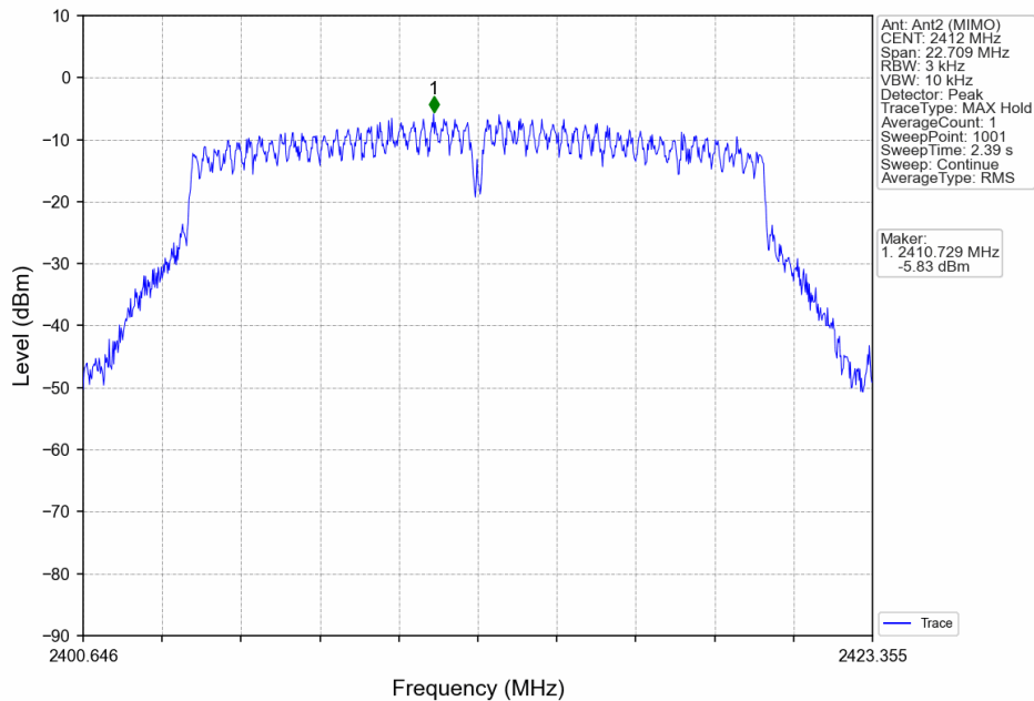
802.11g_LCH_2412MHz_MIMO_NTNV
