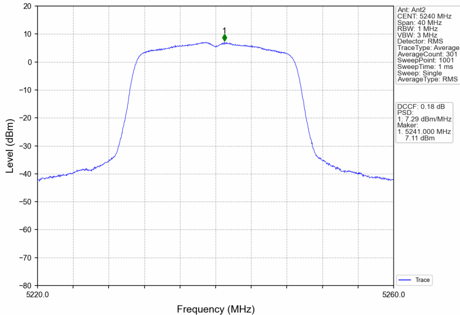
802.11n(HT20)_HCH_5240MHz_MIMO_NTNV
