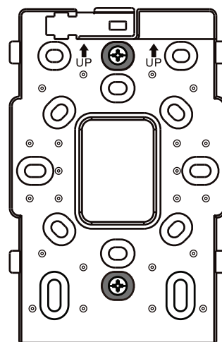
Halterung auf amerikanischem Standard 108 mm × 59 mm Anschlusskasten
