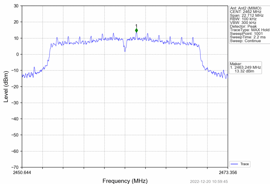
802.11g_HCH_2462MHz_Ant2 (MIMO)_NTNV
