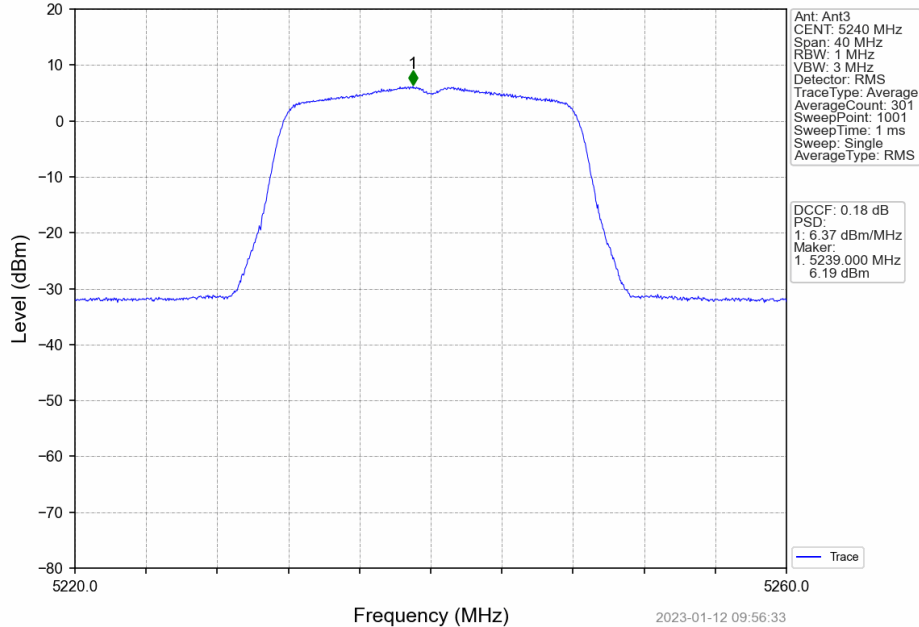
802.11a_HCH_5240MHz_MIMO_NTNV
