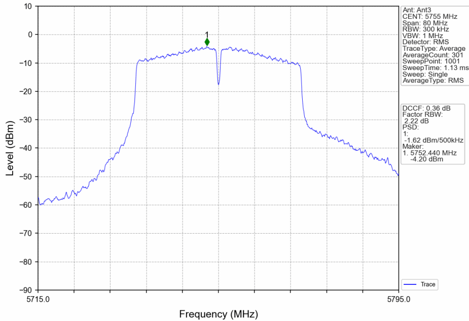
802.11ac(VHT40)_LCH_5755MHz_MIMO_NTNV
