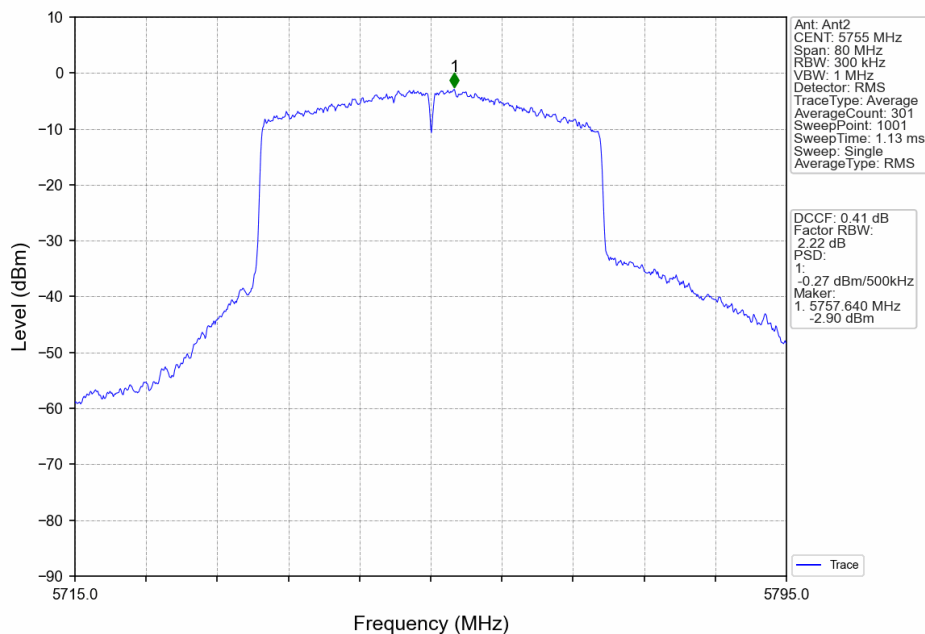
802.11ax(HEW40)_LCH_5755MHz_RU484_Left_Ant2_NTNV
