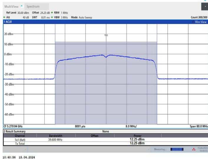
11AX40MIMO_Ant3_5270
