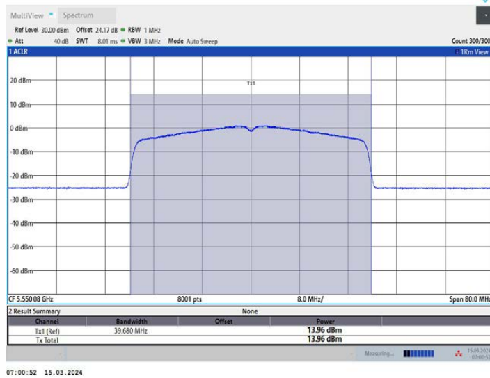
11AX40MIMO_Ant3_5550
