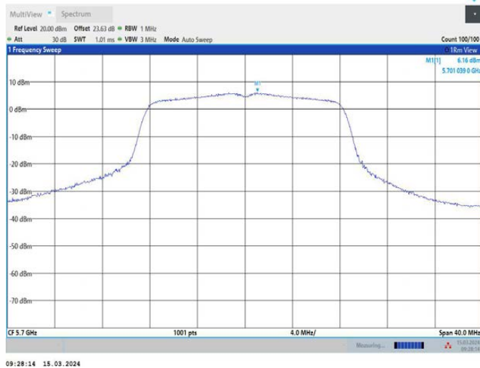
11A_Ant3_5700
