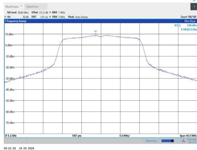
11A_Ant3_5200
