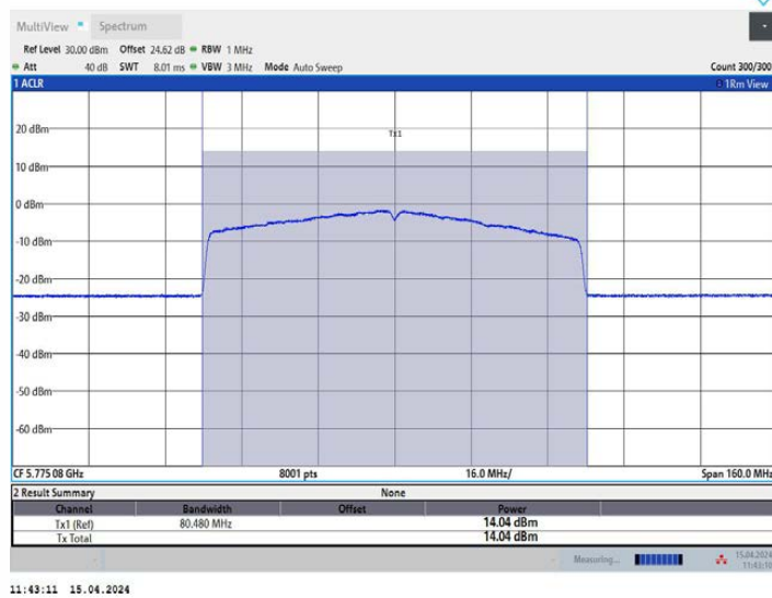
11AX80MIMO_Ant3_5775
