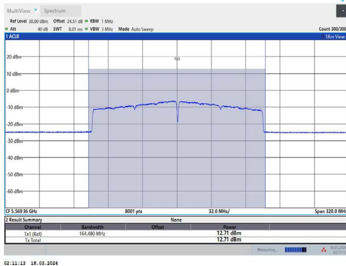
11AX160MIMO_Ant2_5570
