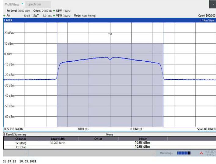
11AX40MIMO_Ant2_5510
