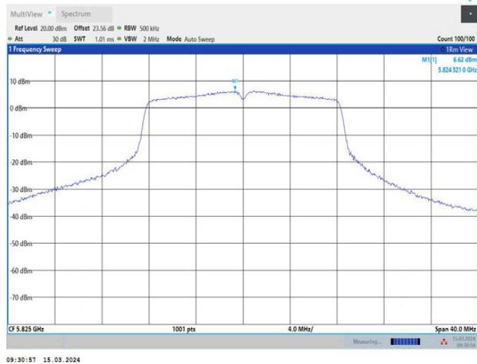
11A_Ant3_5825
