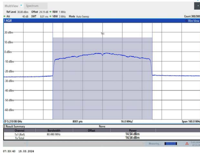
11AX80MIMO_Ant1_5210
