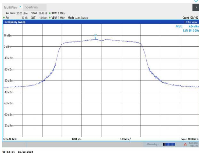
11A_Ant2_5280
