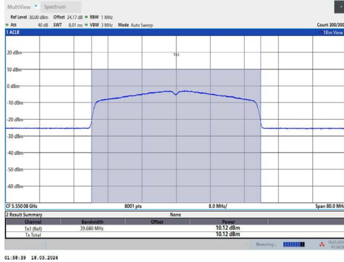
11AX40MIMO_Ant2_5550
