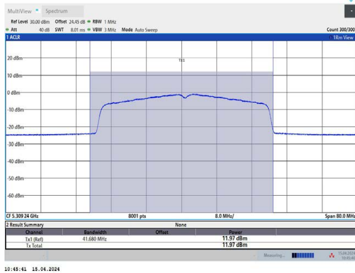
11AX40MIMO_Ant3_5310
