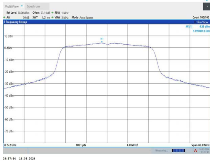
11N20MIMO_Ant3_5200
