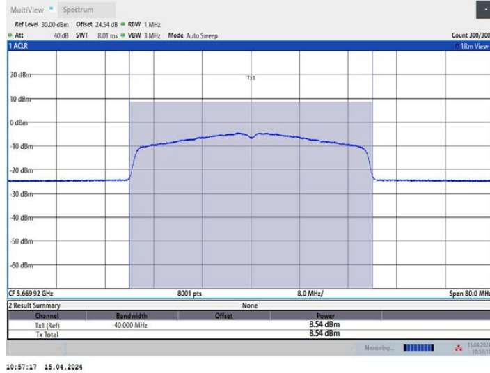
11AX40MIMO_Ant2_5670
