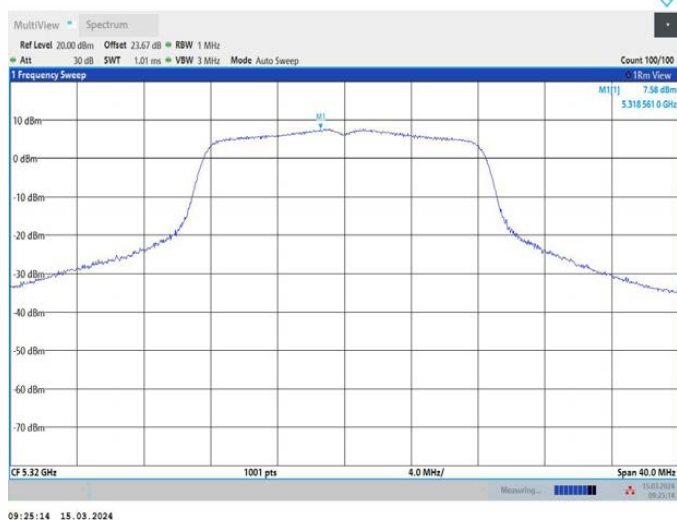
11A_Ant3_5320
