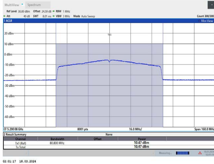
11AX80MIMO_Ant1_5290
