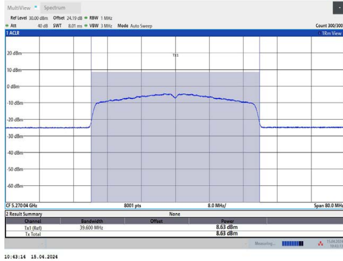
11AX40MIMO_Ant1_5270
