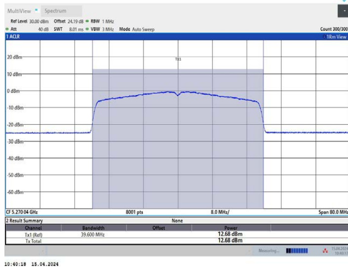
11AX40MIMO_Ant2_5270
