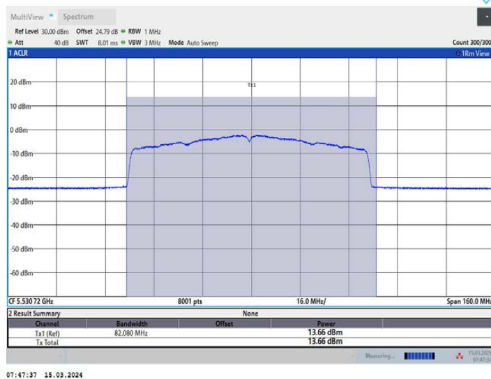
11AX80MIMO_Ant2_5530
