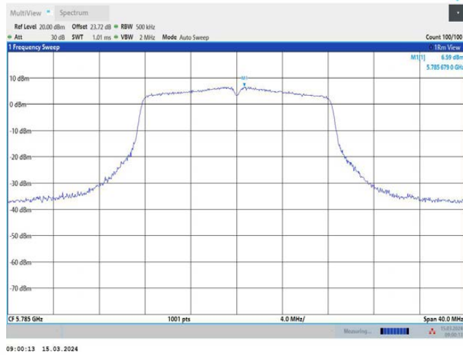
11A_Ant2_5785
