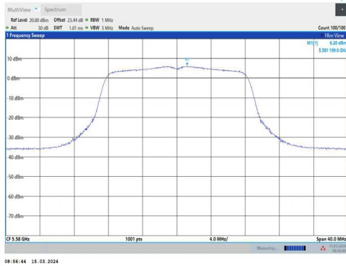
11A_Ant2_5580
