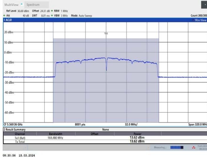
11AX160MIMO_Ant3_5570
