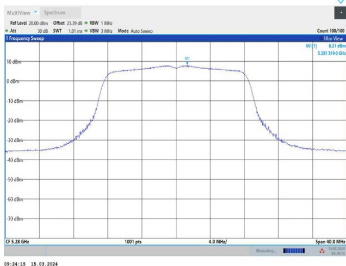
11A_Ant3_5280
