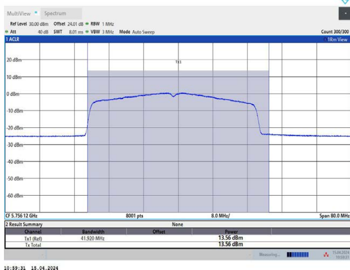
11AX40MIMO_Ant3_5755
