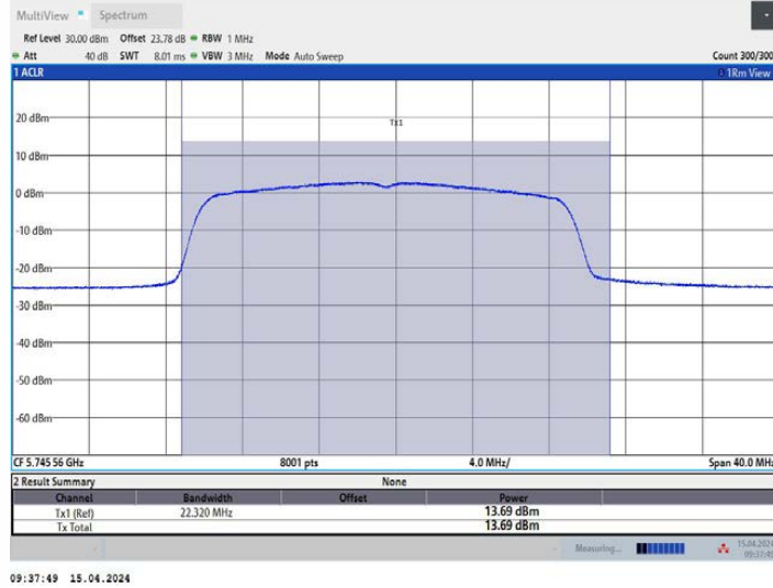
11AX20MIMO_Ant3_5745
