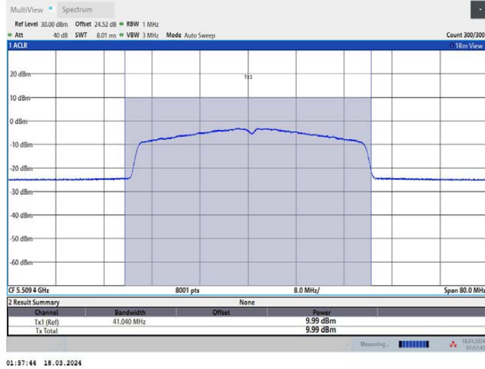
11AX40MIMO_Ant3_5510
