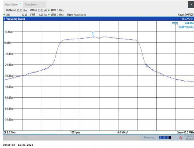
11A_Ant2_5700
