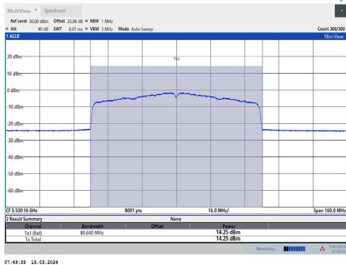
11AX80MIMO_Ant3_5530
