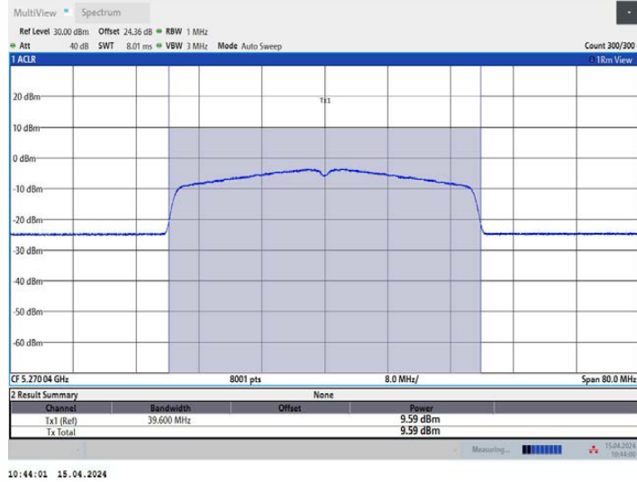
11AX40MIMO_Ant3_5270
