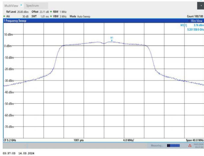
11N20MIMO_Ant2_5200
