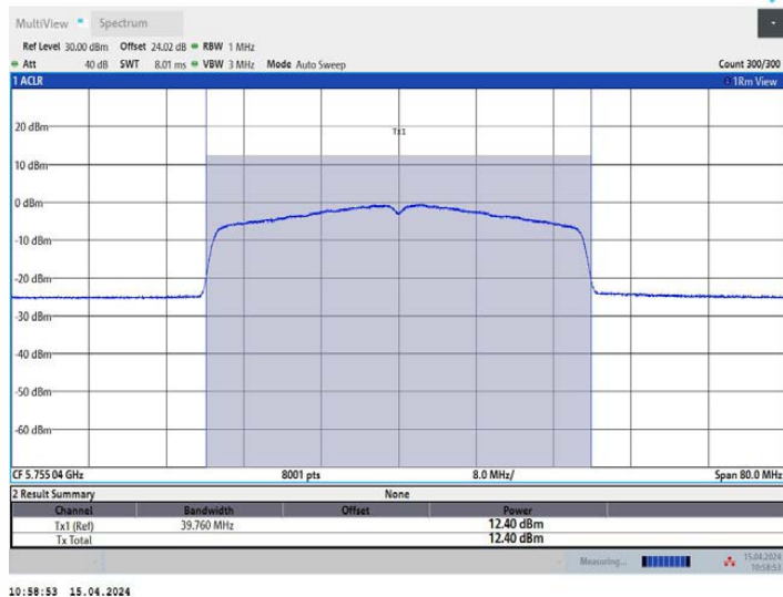
11AX40MIMO_Ant2_5755
