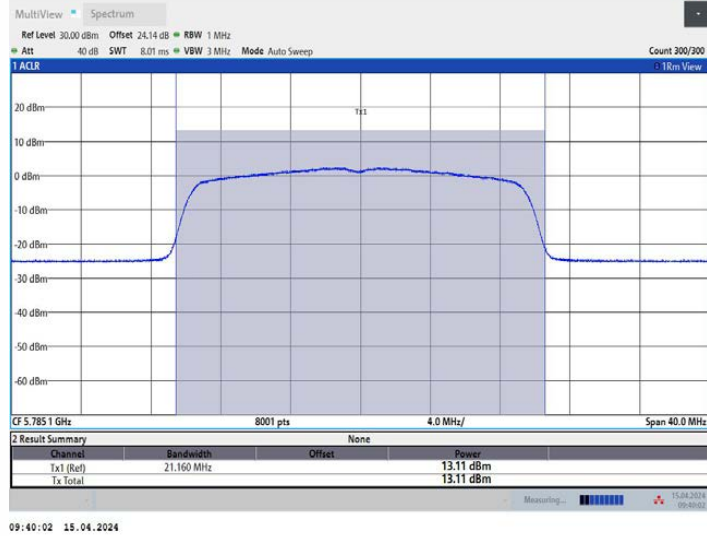
11AX20MIMO_Ant2_5785
