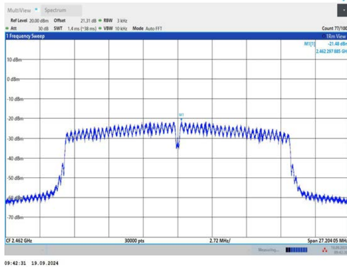
11N20MIMO_Ant2_2462
