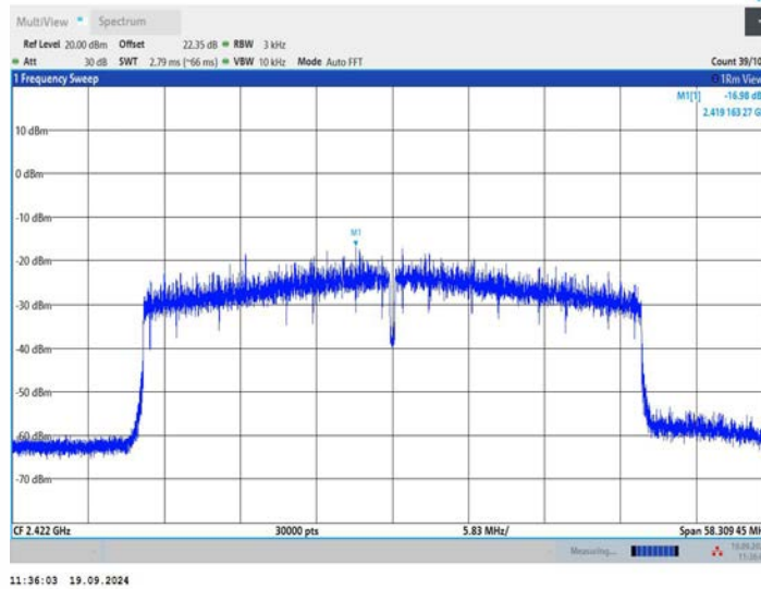
11BE40MIMO_Ant2_2422
