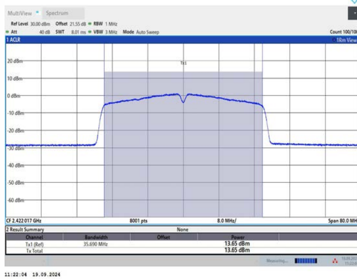
11N40MIMO_Ant2_2422
