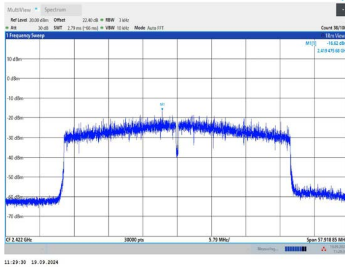
11AX40MIMO_Ant2_2422
