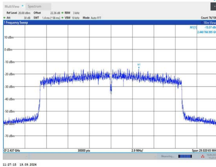
11AX20MIMO_Ant2_2437
