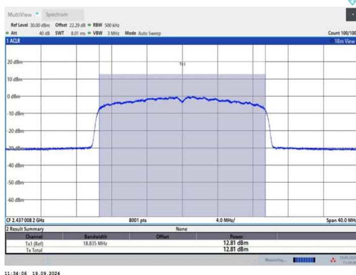
11BE20MIMO_Ant2_2437
