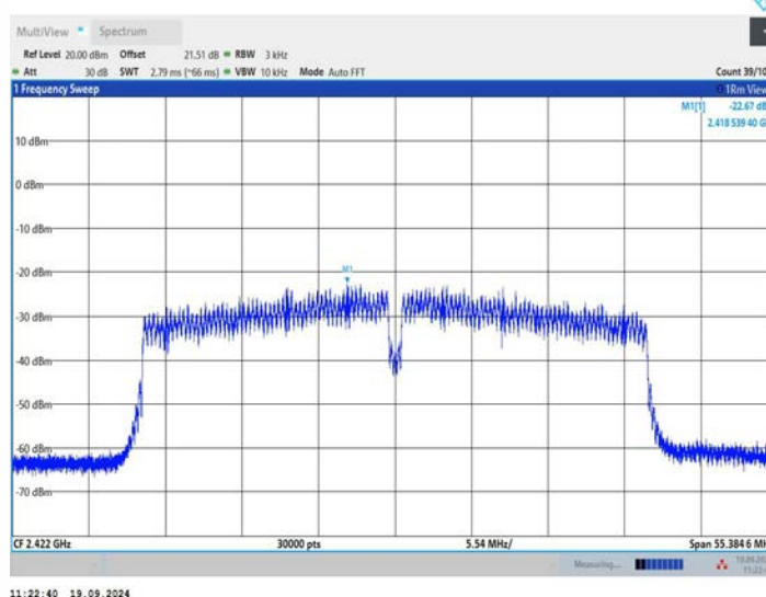
11N40MIMO_Ant2_2422
