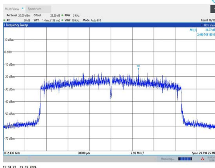
11BE20MIMO_Ant2_2437
