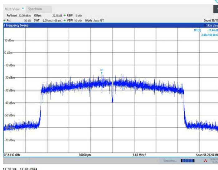
11BE40MIMO_Ant1_2437
