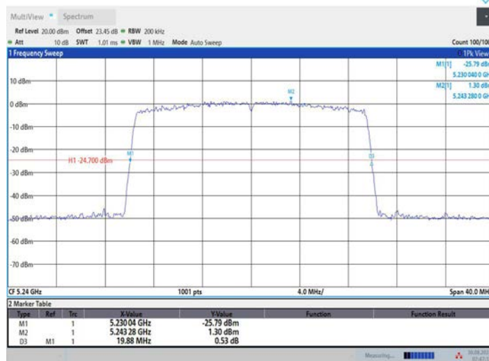
11BE20MIMO_Ant2_5240
