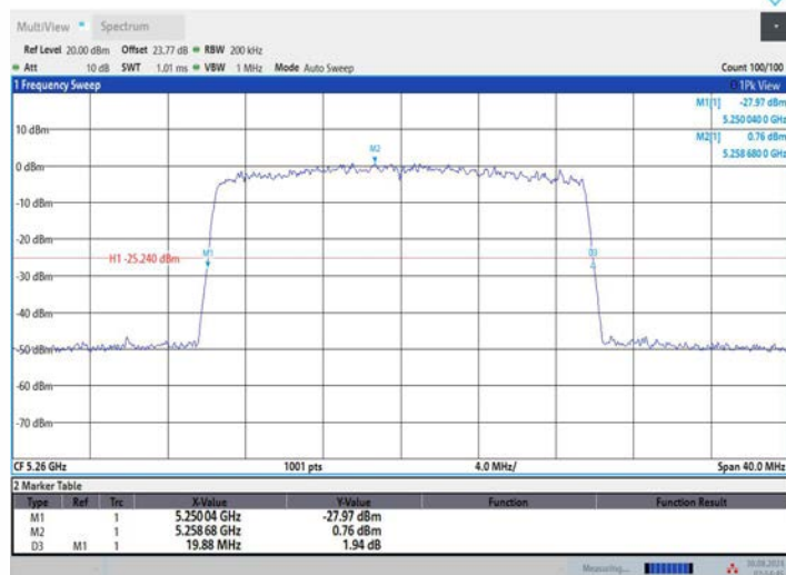
11BE20MIMO_Ant3_5260
