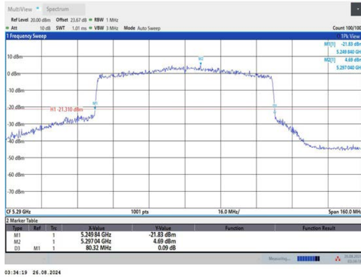
11AX80MIMO_Ant3_5290
