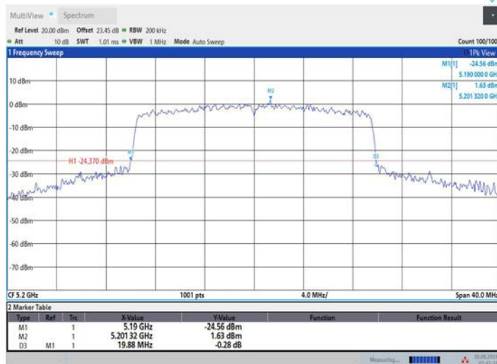
11BE20MIMO_Ant3_5200
