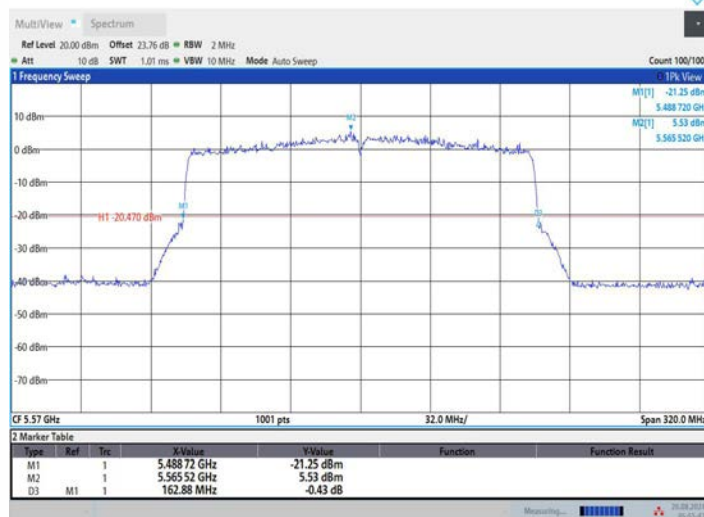
11AX160MIMO_Ant3_5570
