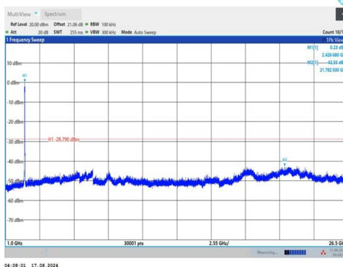
11N40MIMO_Ant2_2422_1000~26500
