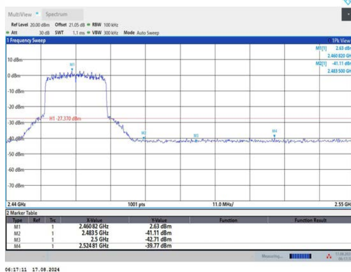
11AX20MIMO_Ant2_High_2462
