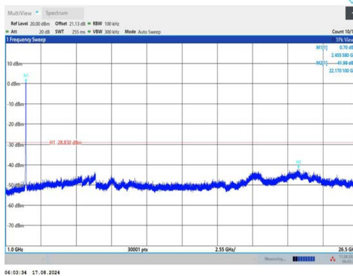
11N40MIMO_Ant2_2452_0~Reference
