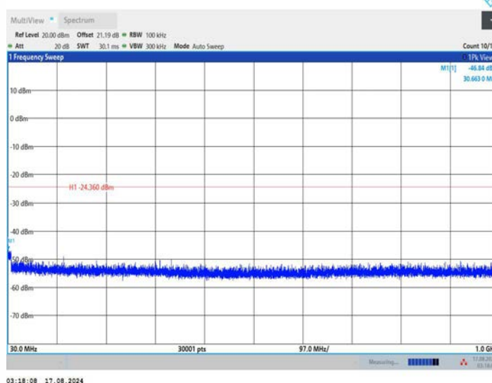
11B_Ant2_2412_30~1000
