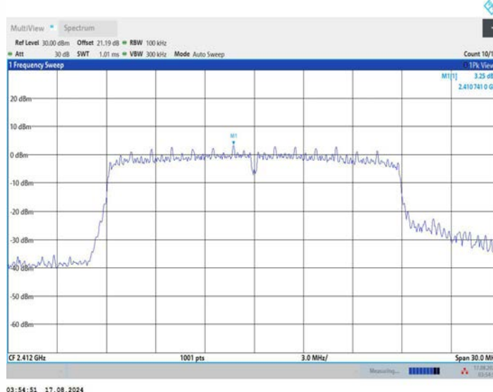
11N20MIMO_Ant2_2412_0~Reference
