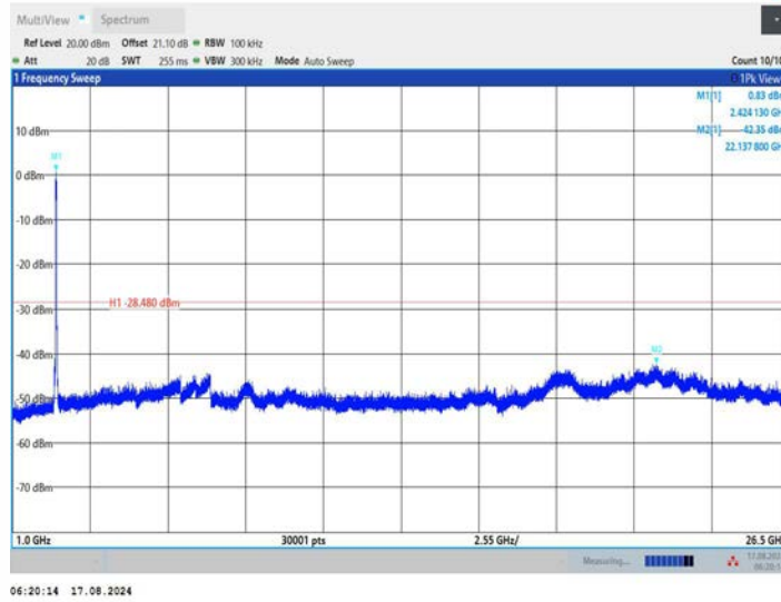
11AX40MIMO_Ant2_2422_0~Reference
