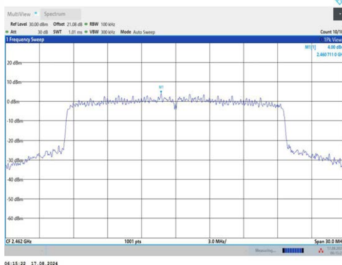
11AX20MIMO_Ant1_2462_0~Reference
