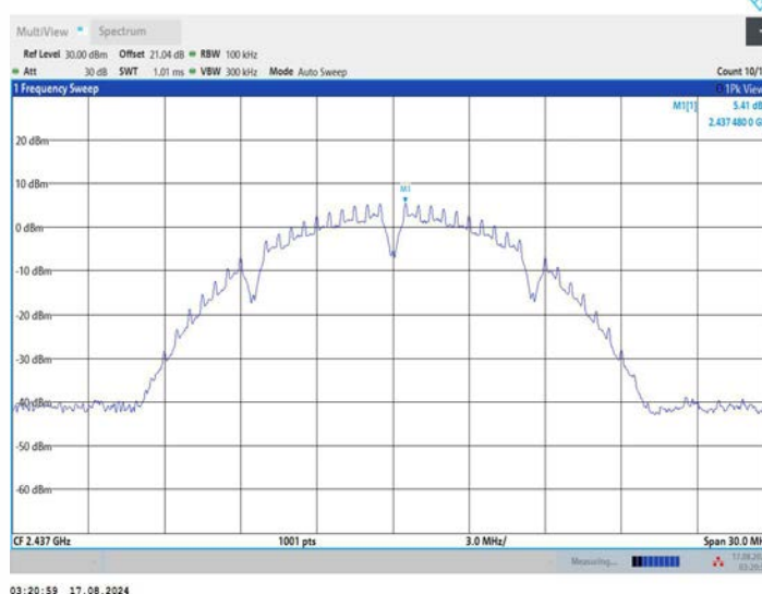
11B_Ant2_2437_0~Reference
