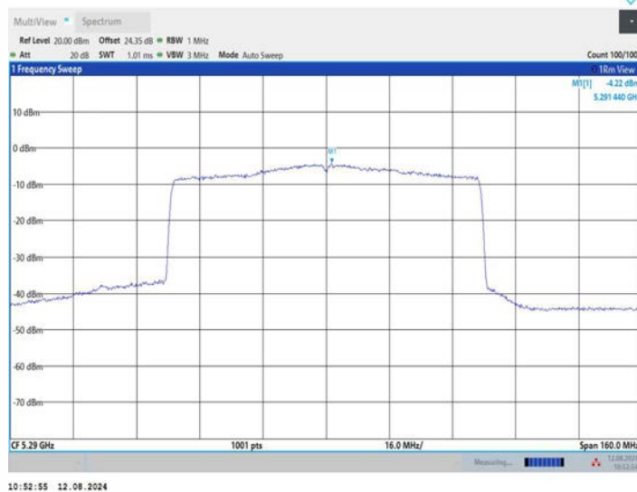
11AX80MIMO_Ant3_5290
