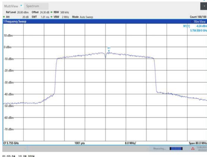
11AX40MIMO_Ant3_5755
