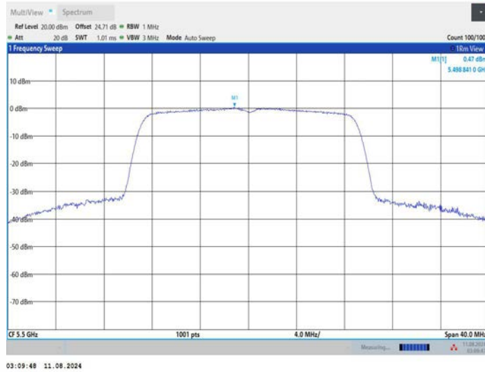
11AC20MIMO_Ant3_5500
