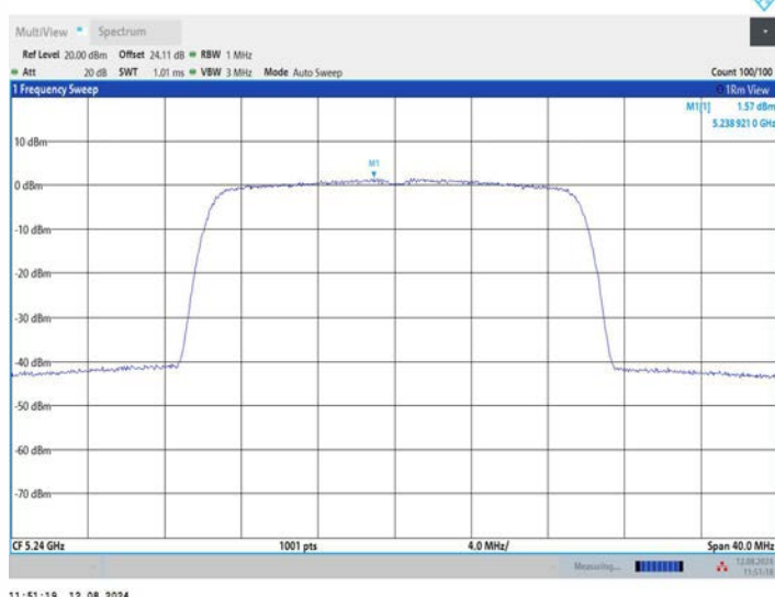
11BE20MIMO_Ant2_5240
