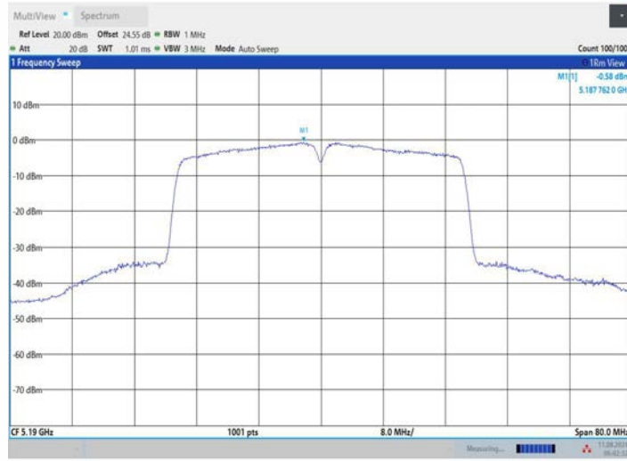
11AC40MIMO_Ant3_5190
