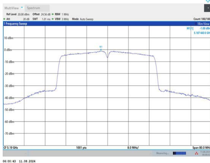
11AC40MIMO_Ant2_5190
