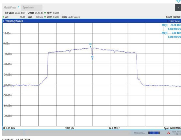
11AX160MIMO_Ant3_5250_UNII-1
