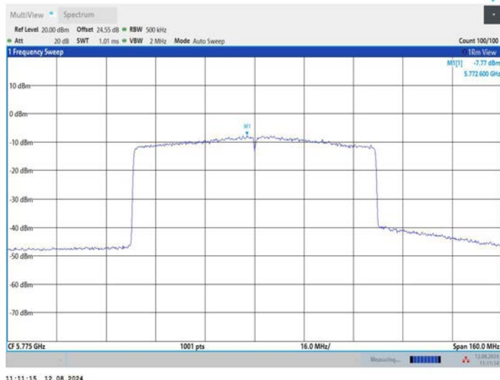
11AX80MIMO_Ant3_5775
