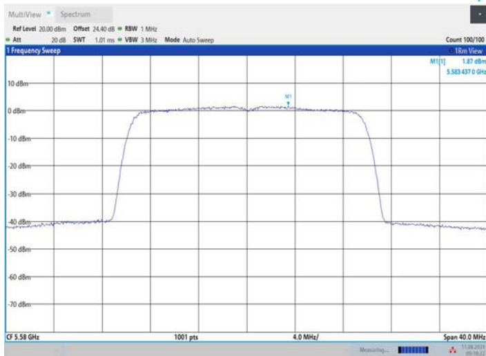
11AX20MIMO_Ant3_5580
