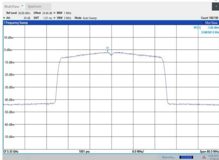
11AX40MIMO_Ant3_5550
