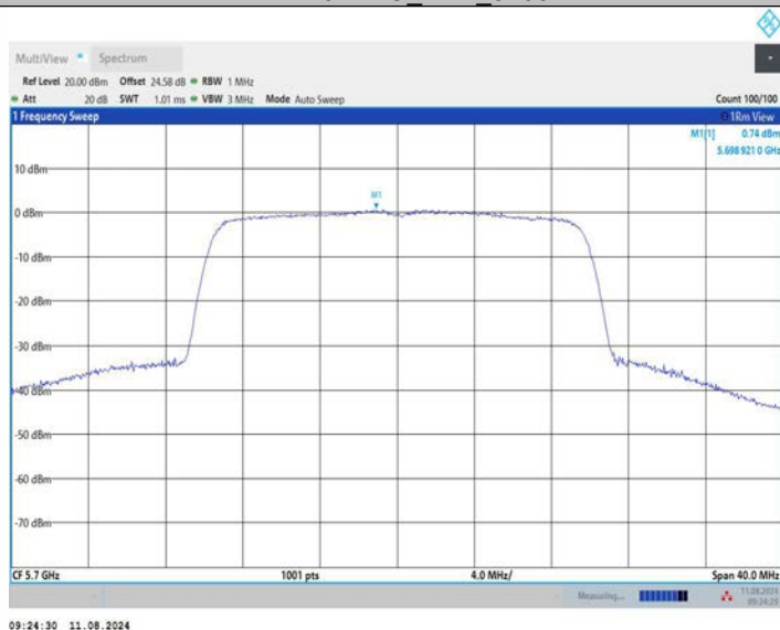
11AX20MIMO_Ant3_5700
