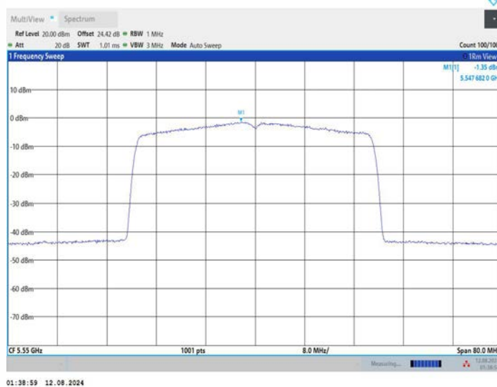
11AX40MIMO_Ant2_5550
