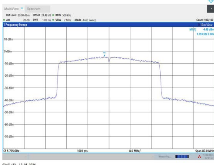
11AX40MIMO_Ant3_5795
