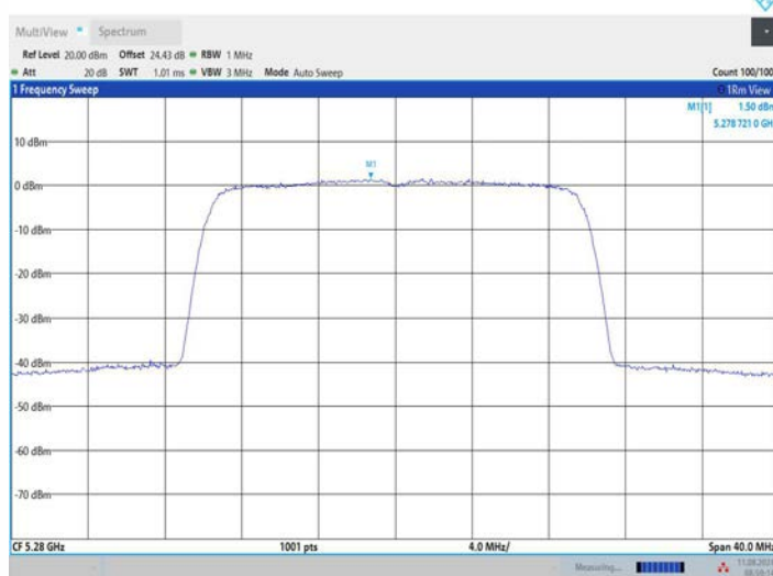
11AX20MIMO_Ant3_5280
