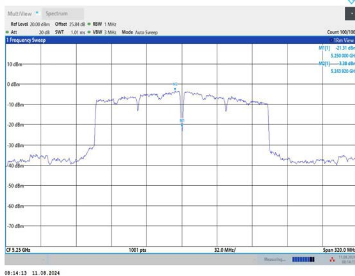
11AC160MIMO_Ant1_5250_UNII-2A
