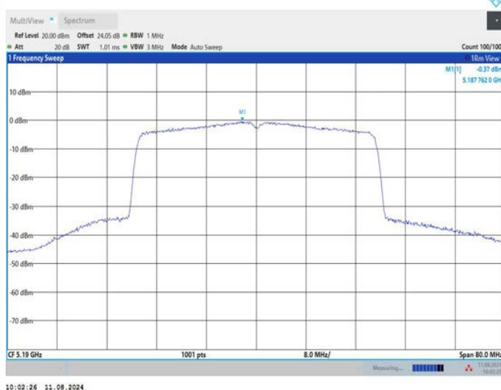
11AX40MIMO_Ant3_5190
