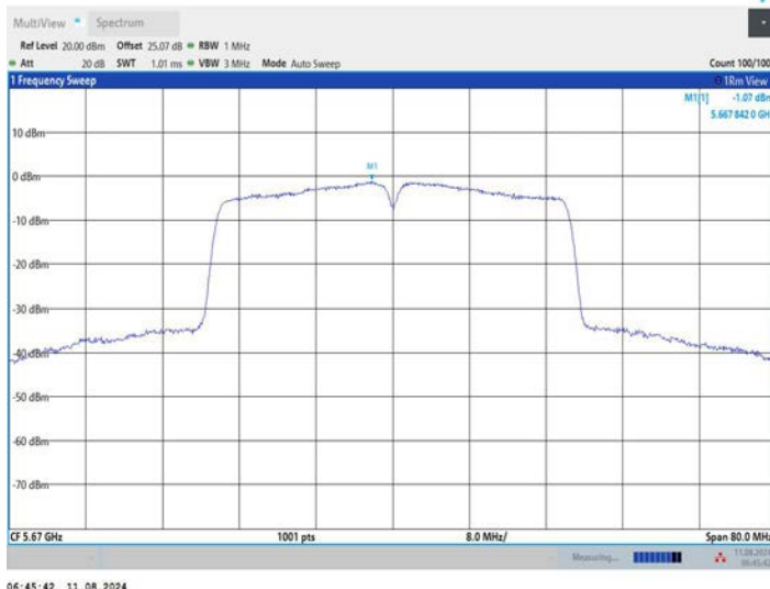
11AC40MIMO_Ant3_5670
