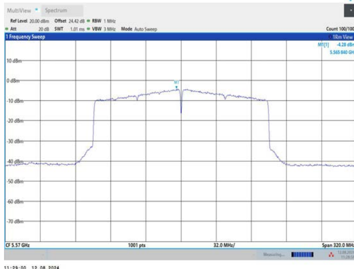
11AX160MIMO_Ant2_5570
