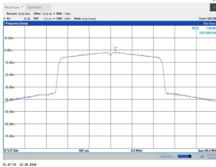
11AX40MIMO_Ant3_5670
