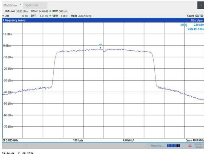
11AX20MIMO_Ant3_5825
