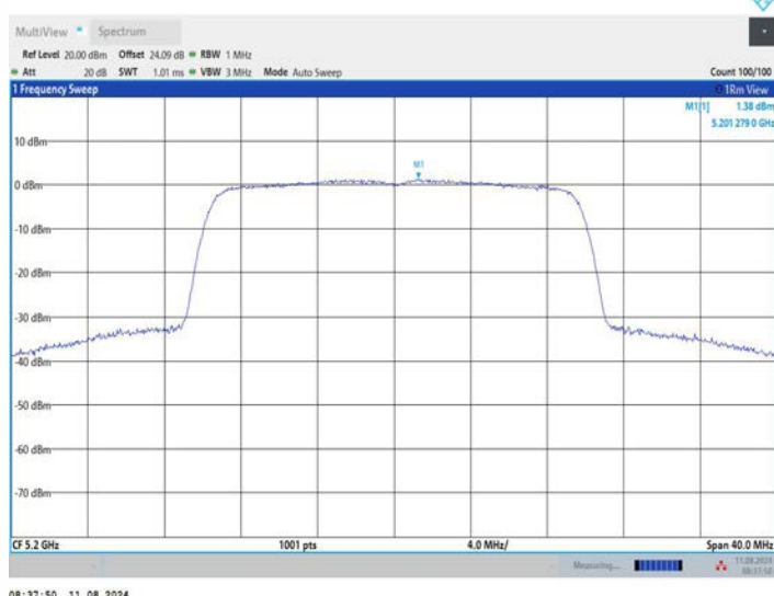
11AX20MIMO_Ant2_5200
