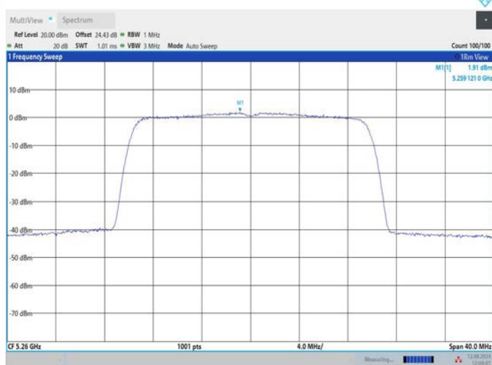
11BE20MIMO_Ant3_5260
