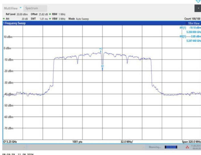
11AC160MIMO_Ant2_5250_UNII-1
