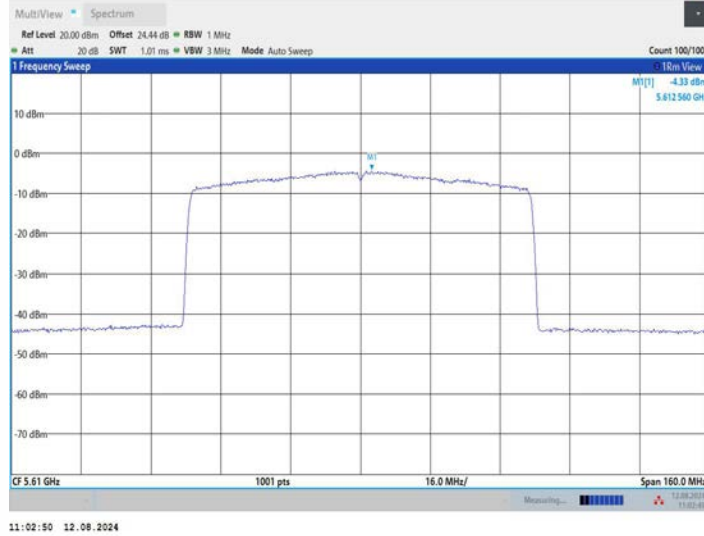
11AX80MIMO_Ant2_5610
