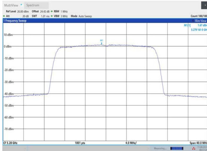
11AX20MIMO_Ant2_5280
