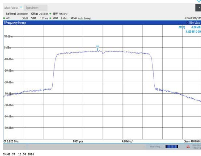
11AX20MIMO_Ant2_5825
