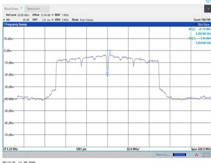
11AC160MIMO_Ant3_5250_UNII-2A
