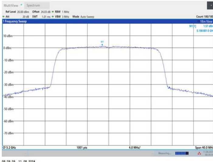
11AX20MIMO_Ant3_5200
