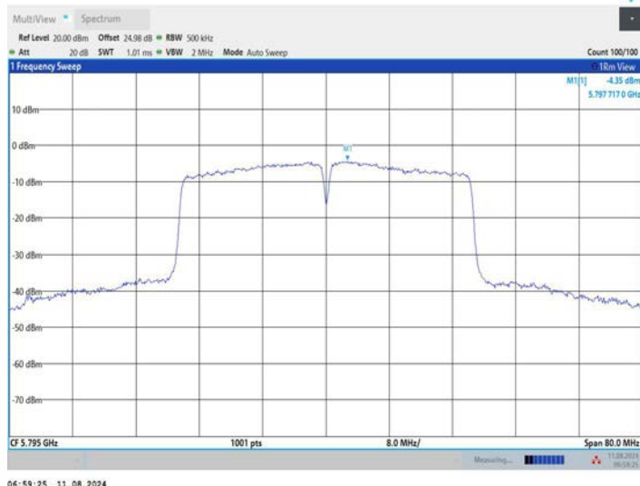
11AC40MIMO_Ant3_5795
