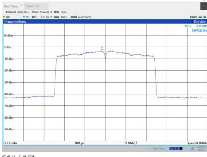
11AC80MIMO_Ant3_5610
