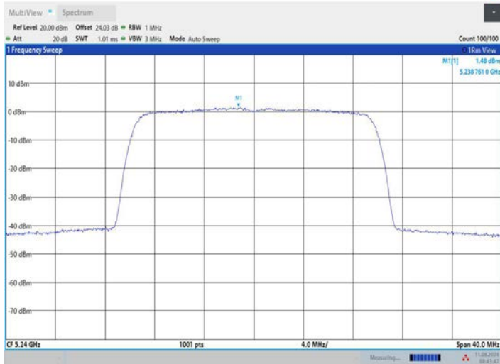
11AX20MIMO_Ant2_5240
