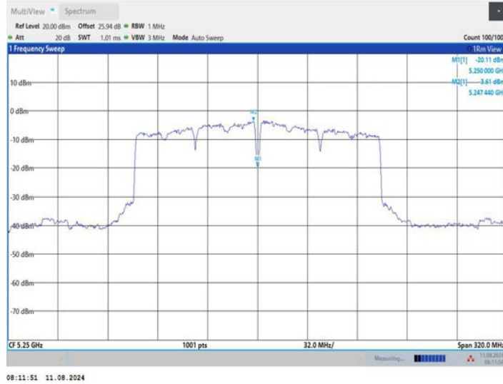
11AC160MIMO_Ant3_5250_UNII-1
