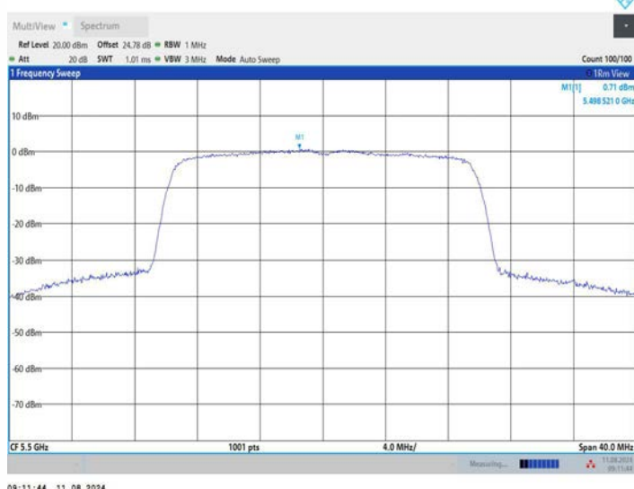
11AX20MIMO_Ant3_5500
