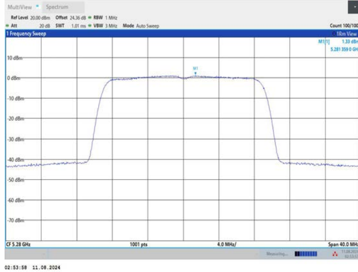
11AC20MIMO_Ant3_5280
