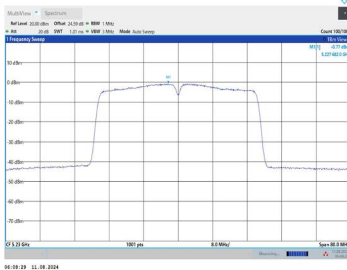
11AC40MIMO_Ant3_5230
