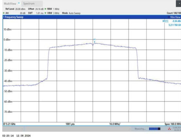
11AX80MIMO_Ant3_5210
