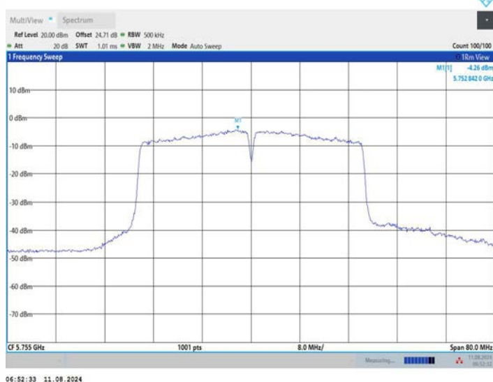
11AC40MIMO_Ant3_5755
