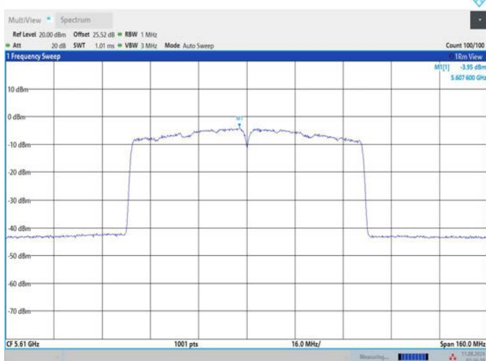
11AC80MIMO_Ant2_5610
