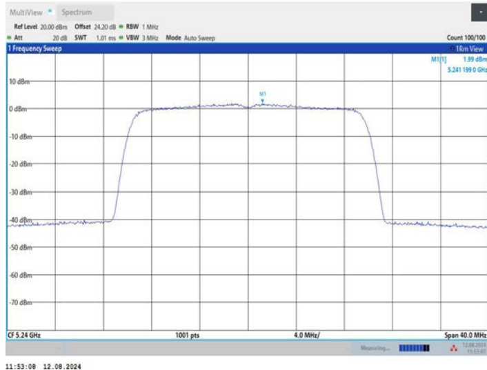
11BE20MIMO_Ant3_5240
