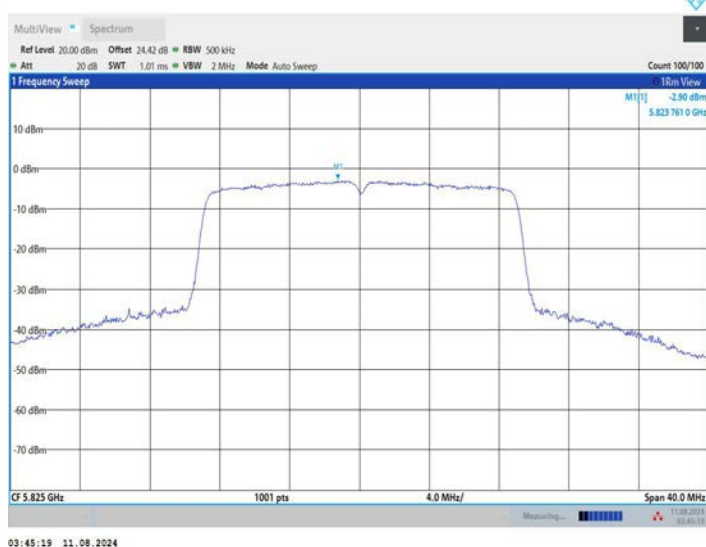
11AC20MIMO_Ant3_5825
