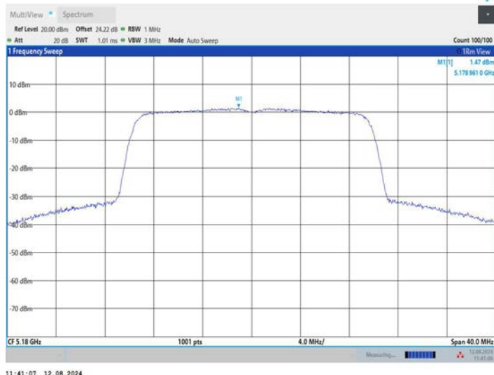
11BE20MIMO_Ant3_5180
