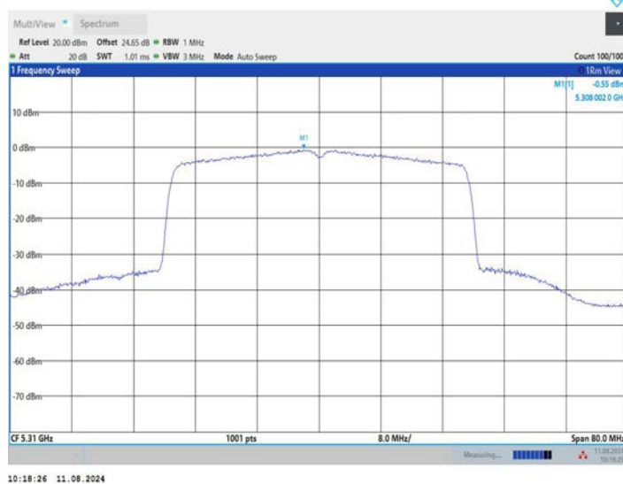
11AX40MIMO_Ant2_5310
