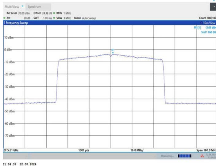
11AX80MIMO_Ant3_5610
