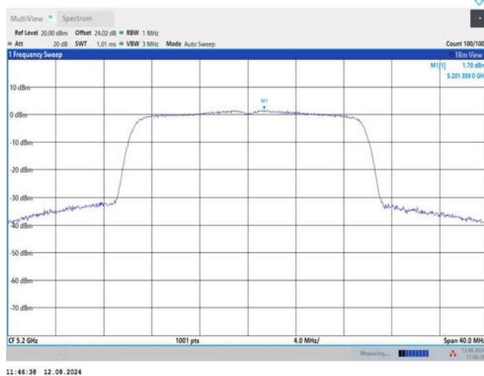
11BE20MIMO_Ant3_5200
