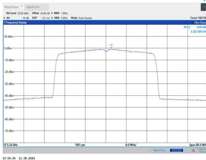
11AX40MIMO_Ant2_5230
