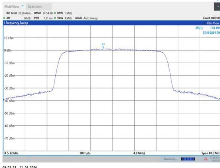
11AX20MIMO_Ant3_5320
