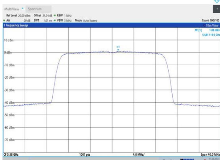
11AX20MIMO_Ant2_5580
