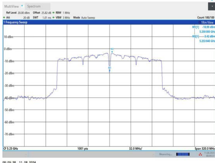
11AC160MIMO_Ant2_5250_UNII-2A
