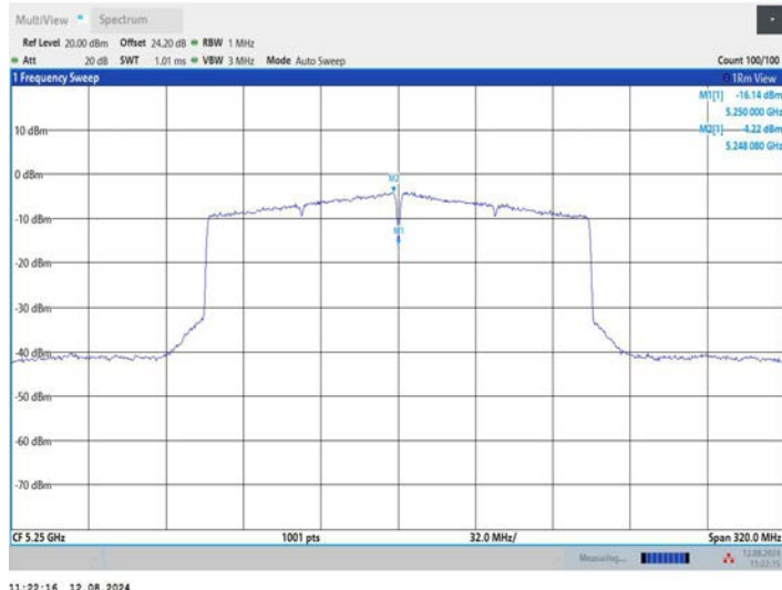
11AX160MIMO_Ant2_5250_UNII-1
