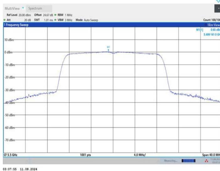
11AC20MIMO_Ant2_5500
