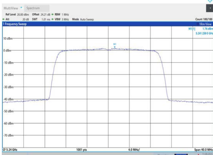
11AX20MIMO_Ant3_5240
