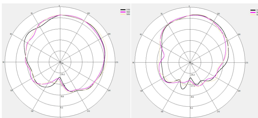
水平角度 2D 方向图
