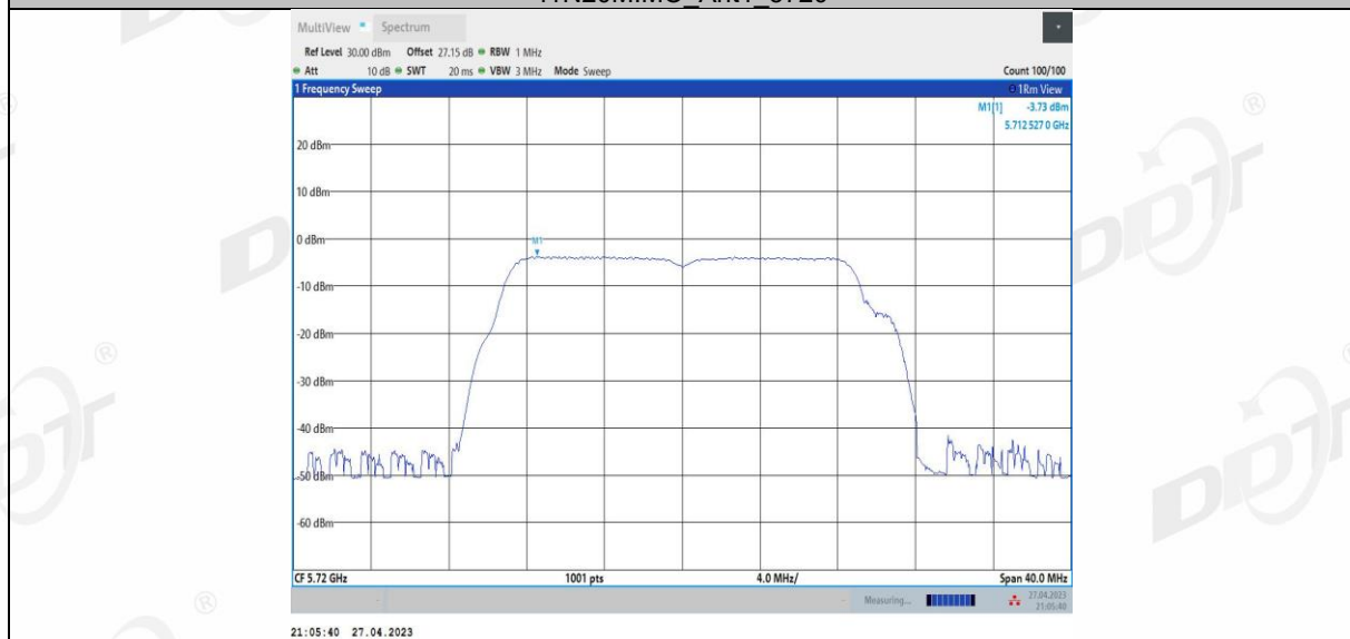
11N20MIMO Ant2 5720
