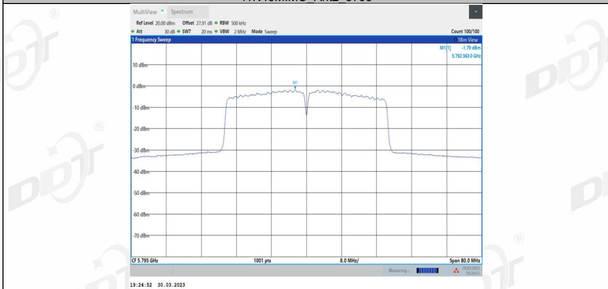
11N40MIMO Ant3 5795
