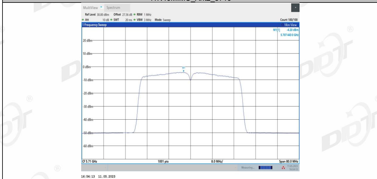
11N40MIMO_Ant3_5710
