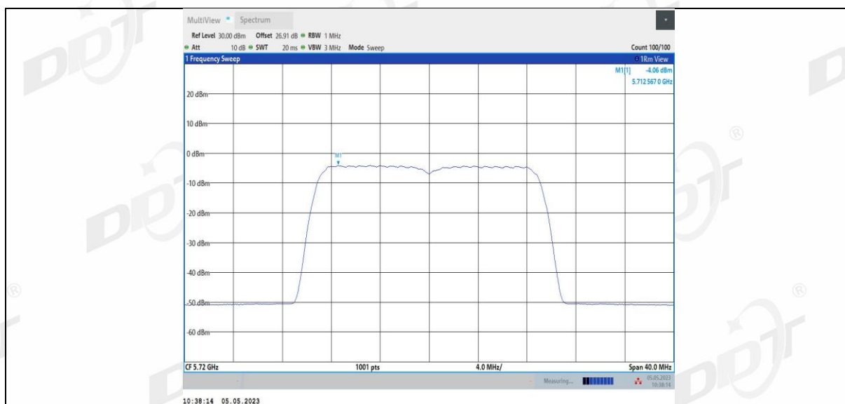
11AX20MIMO_Ant3_5720
