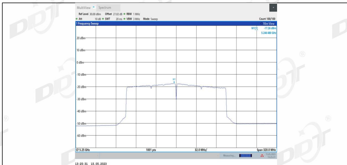
11AX160MIMO Ant4 5250
