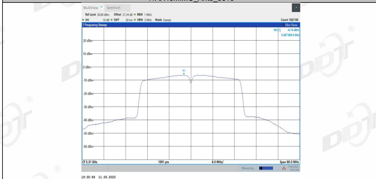
11AX40MIMO_Ant4_5310
