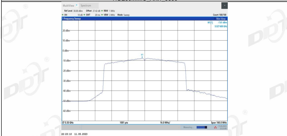
11BE80MIMO_Ant2_5530
