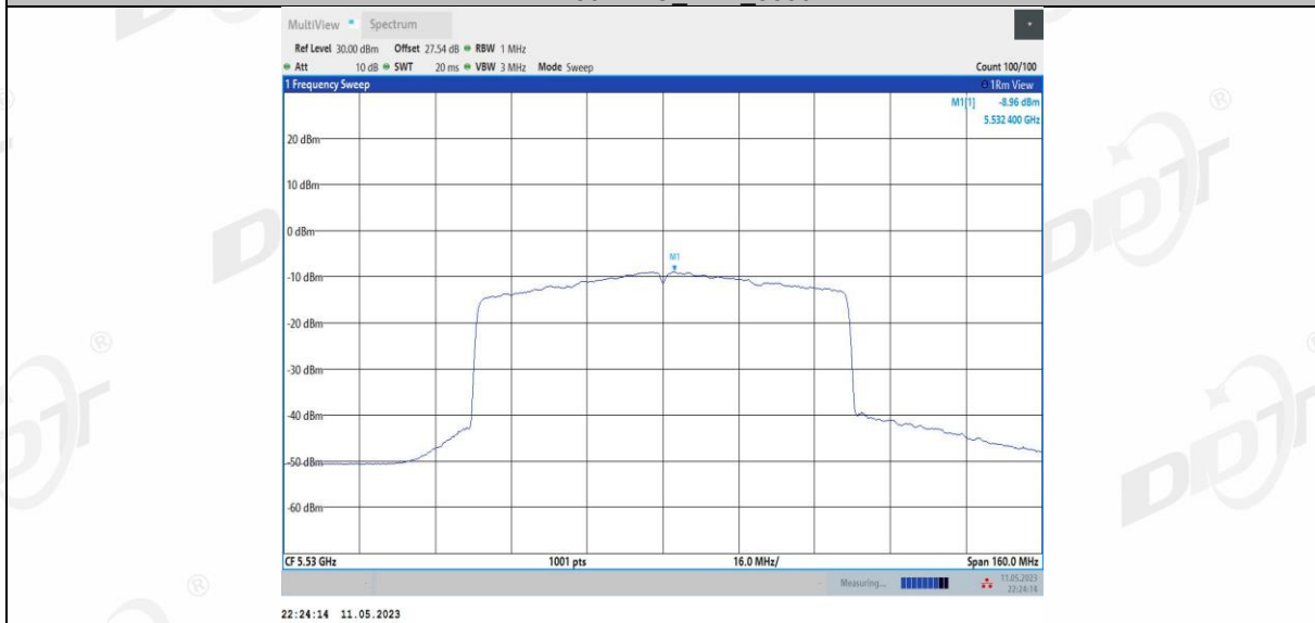
11BE80MIMO_Ant3_5530
