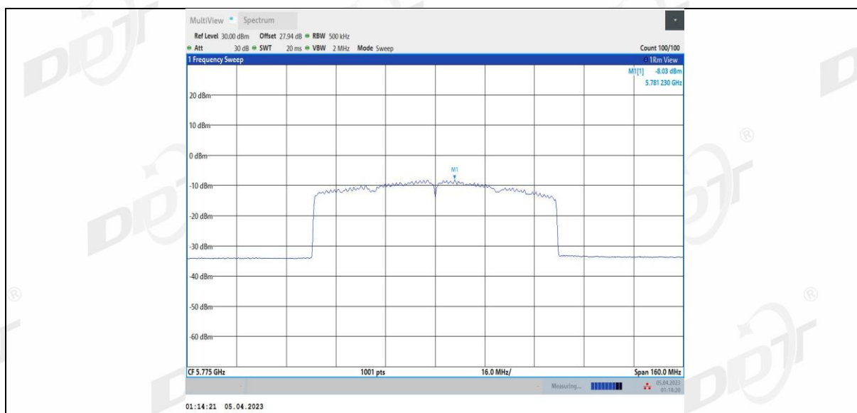
11BE80MIMO Ant4 5775
