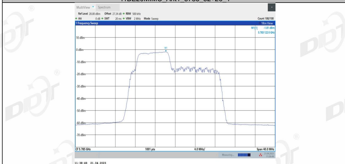
11BE20MIMO Ant1 5785 52+26 2
