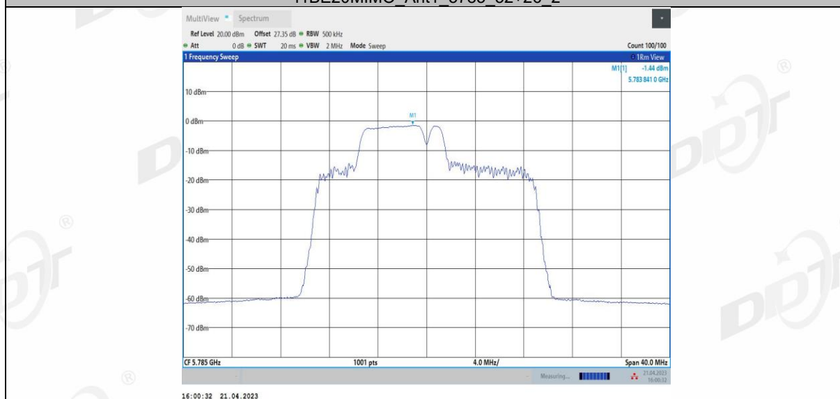
11BE20MIMO Ant1 5785 52+26 3
