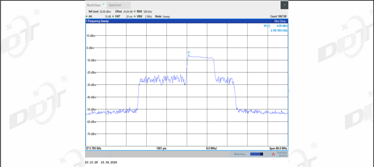
11BE40MIMO_Ant3_5795_106+26_4
