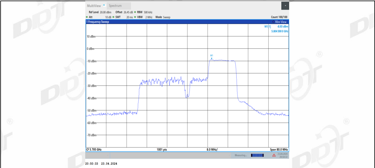
11BE40MIMO_Ant3_5795_106+26_3
