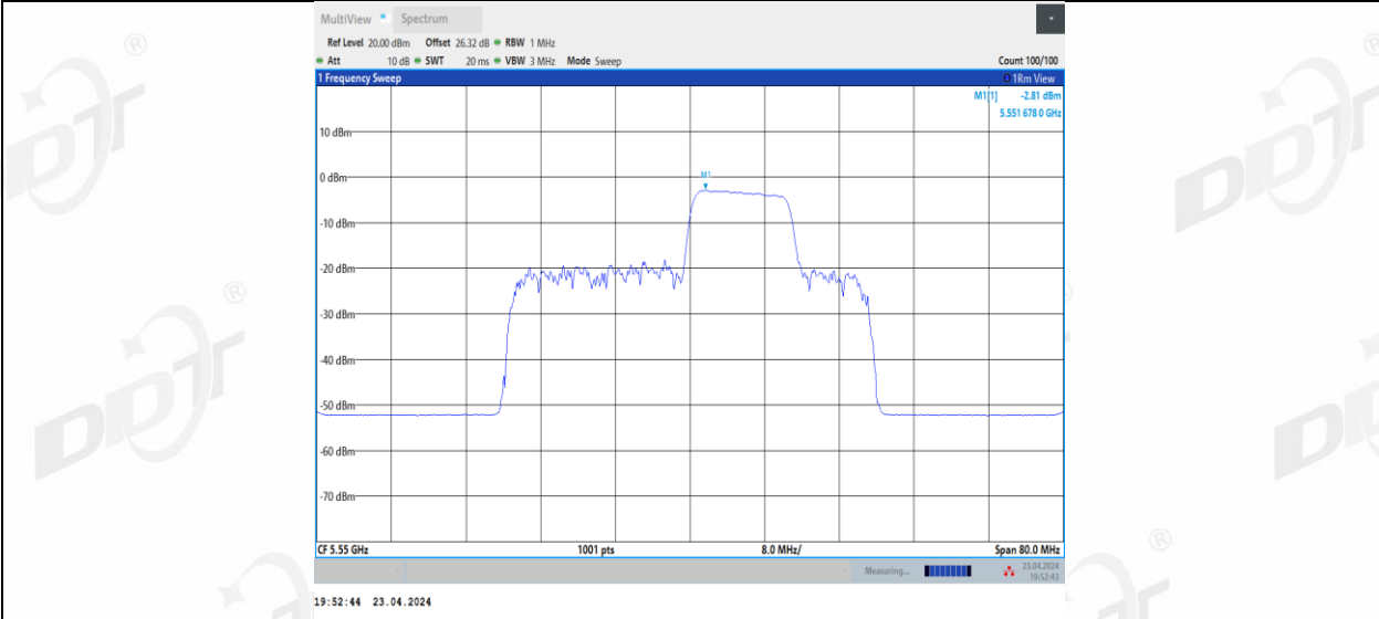
11BE40MIMO_Ant3_5550_106+26_4
