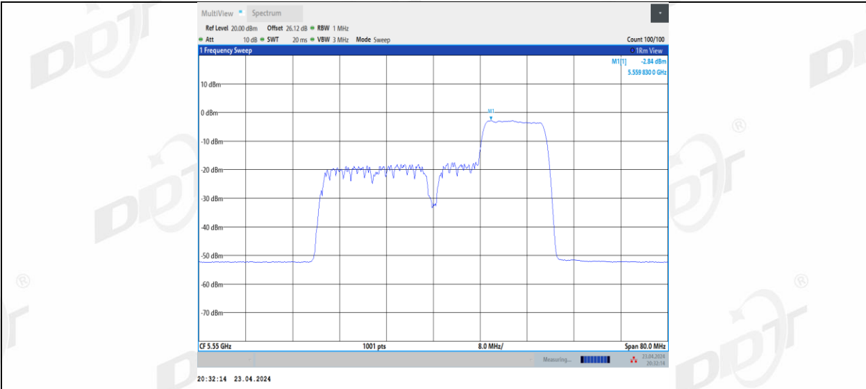
11BE40MIMO_Ant3_5550_106+26_3
