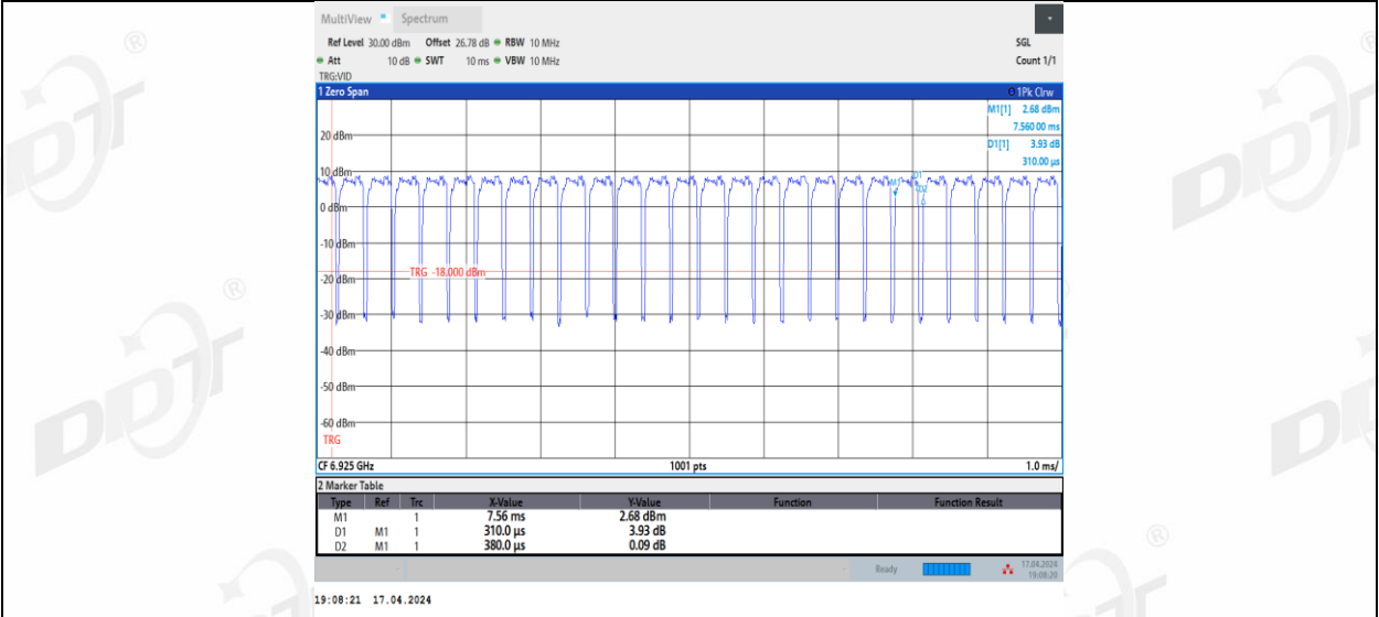
11BE40MIMO_Ant3_6925
