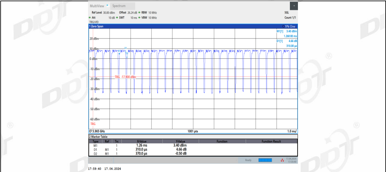
11BE40MIMO_Ant2_5965
