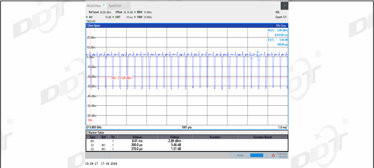
11BE80MIMO_Ant2_6865
