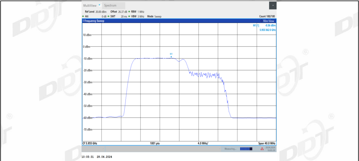
11BE20MIMO_Ant1_5955_106+26_2
