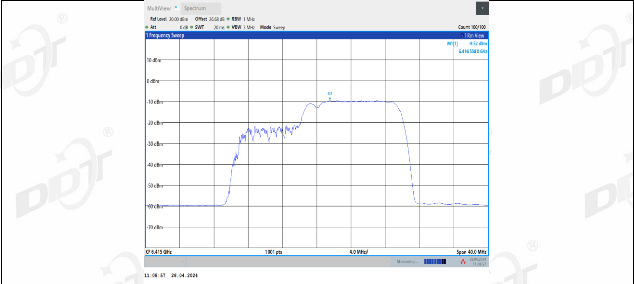
11BE20MIMO_Ant2_6415_52+26_1
