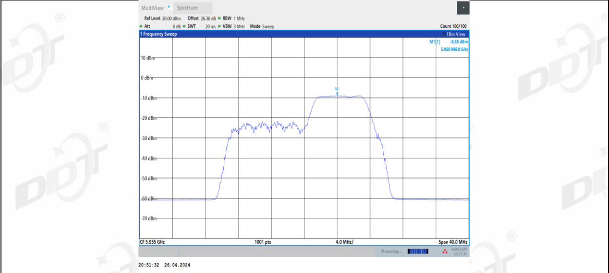
11BE20MIMO_Ant2_5955_106+26_1
