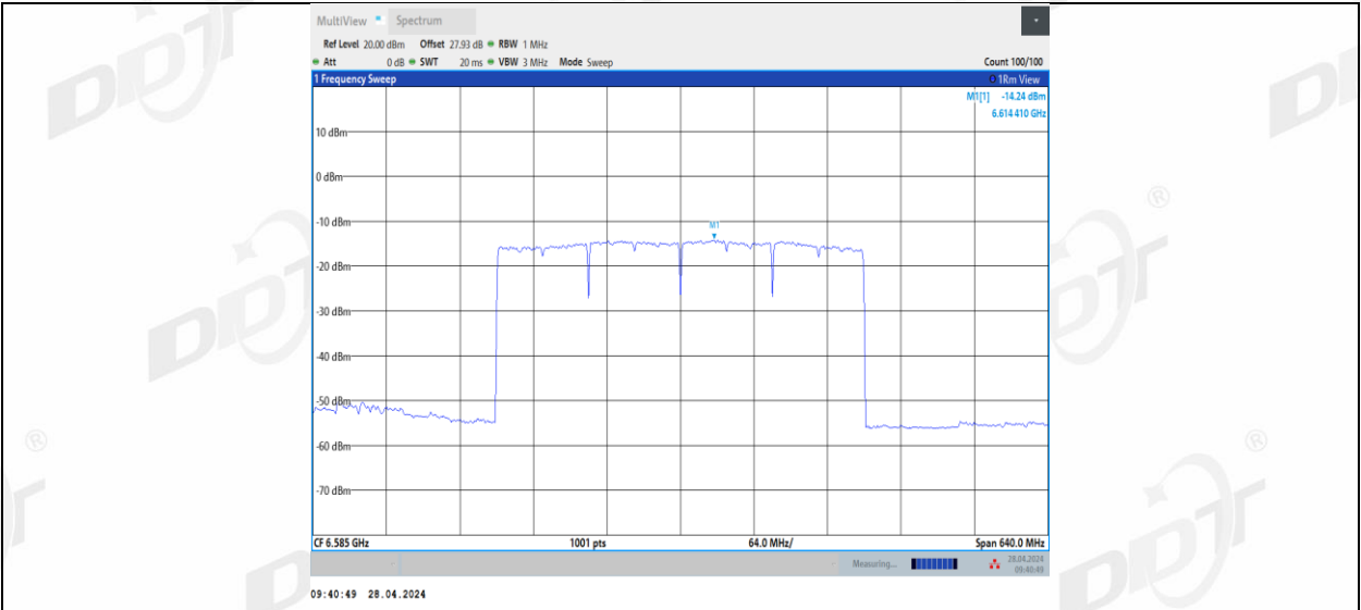
11BE320MIMO_Ant2_6585
