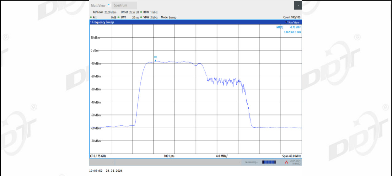
11BE20MIMO_Ant2_6175_106+26_2
