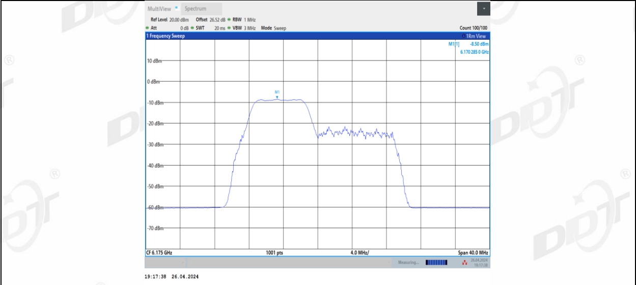
11BE20MIMO_Ant2_6175_52+26_2
