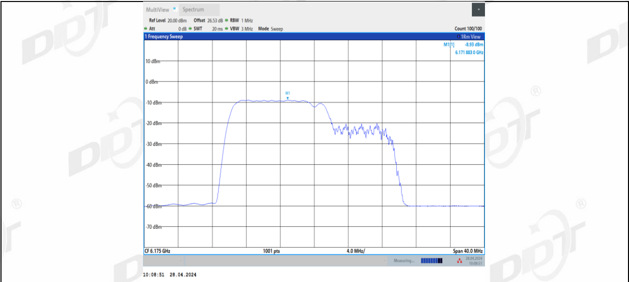
11BE20MIMO_Ant1_6175_106+26_2
