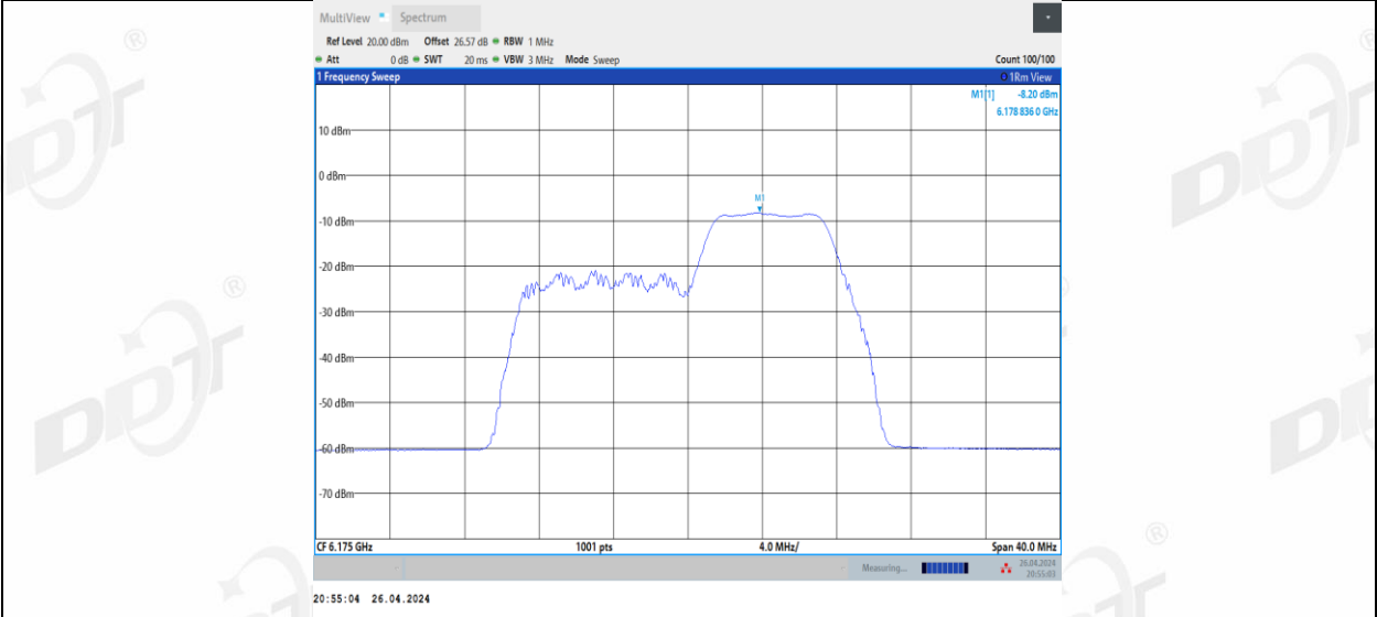
11BE20MIMO_Ant2_6175_106+26_1
