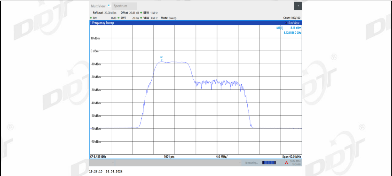
11BE20MIMO Ant1_6435_52+26_2
