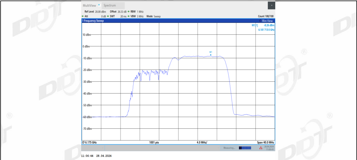
11BE20MIMO_Ant3_6175_52+26_1
