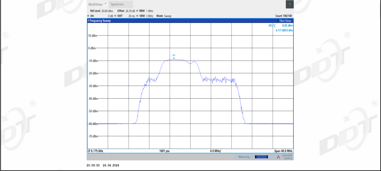
11BE20MIMO_Ant3_6175_52+26_3
