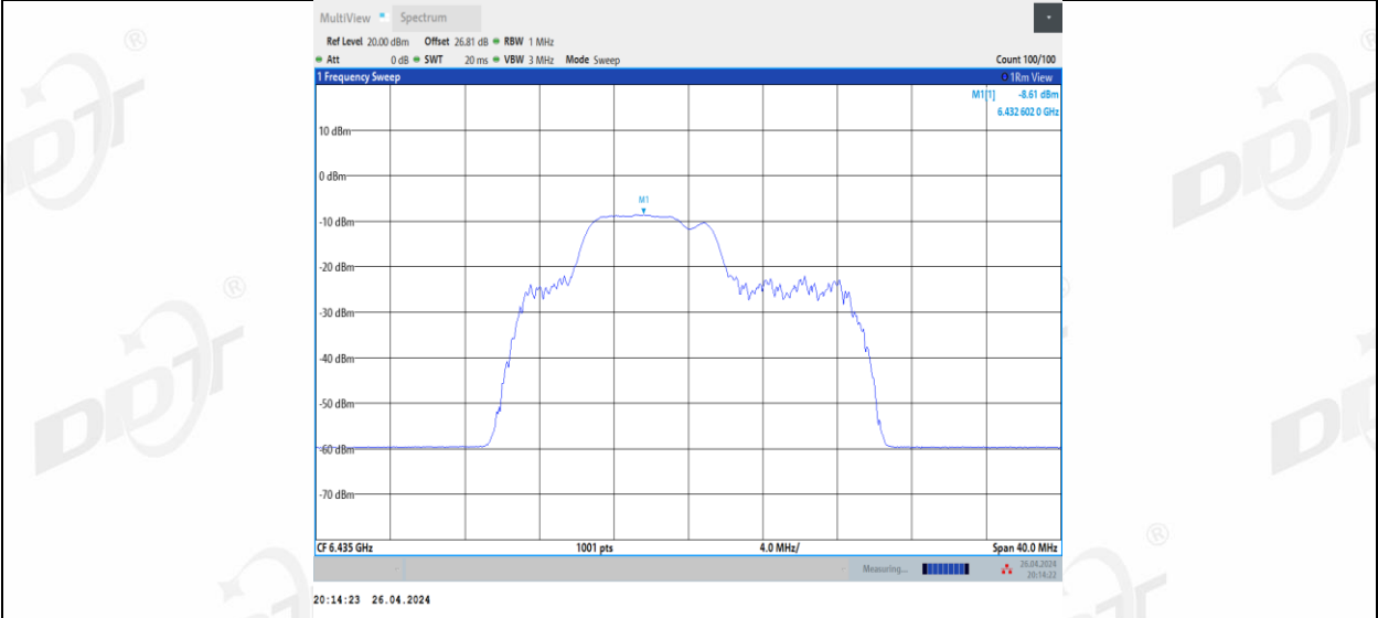
11BE20MIMO Ant1_6435_52+26_3
