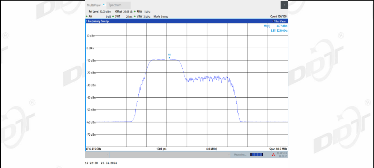
11BE20MIMO_Ant2_6415_52+26_2
