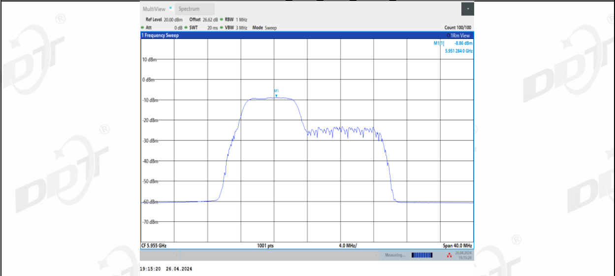
11BE20MIMO_Ant3_5955_52+26_2
