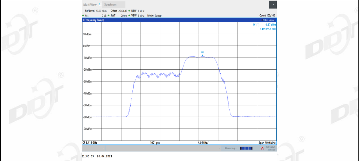
11BE20MIMO_Ant2_6415_106+26_1
