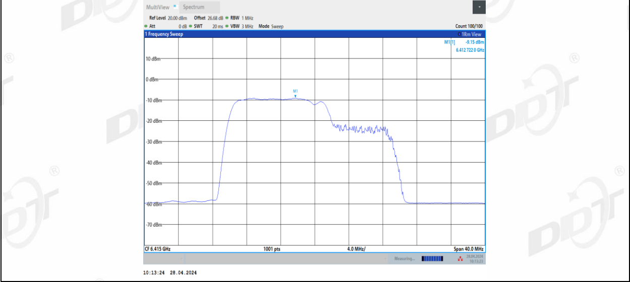
11BE20MIMO_Ant2_6415_106+26_2
