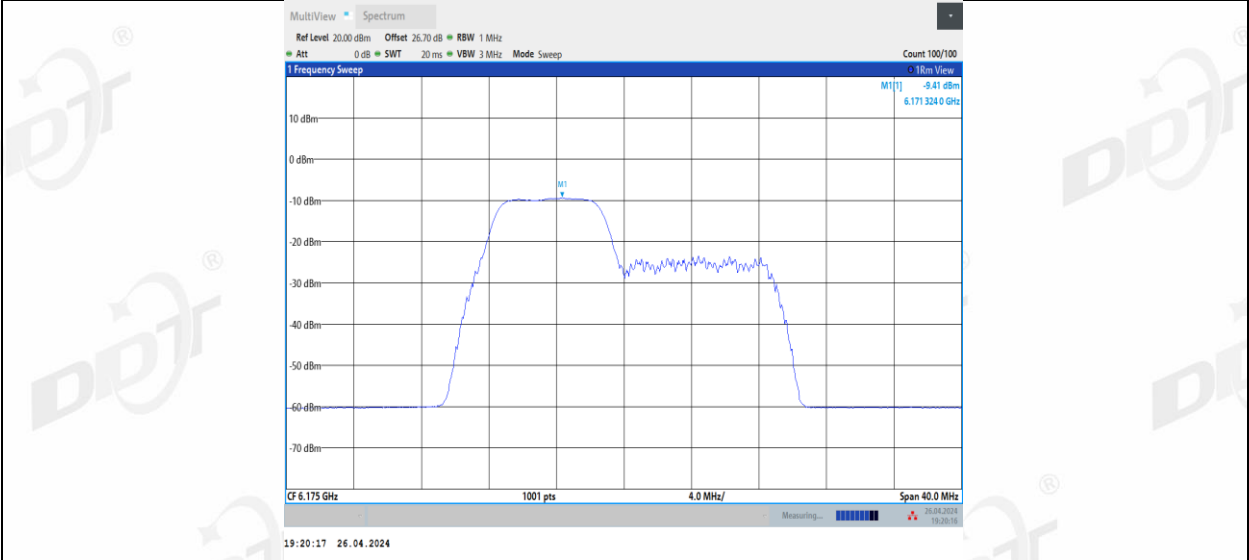
11BE20MIMO_Ant3_6175_52+26_2
