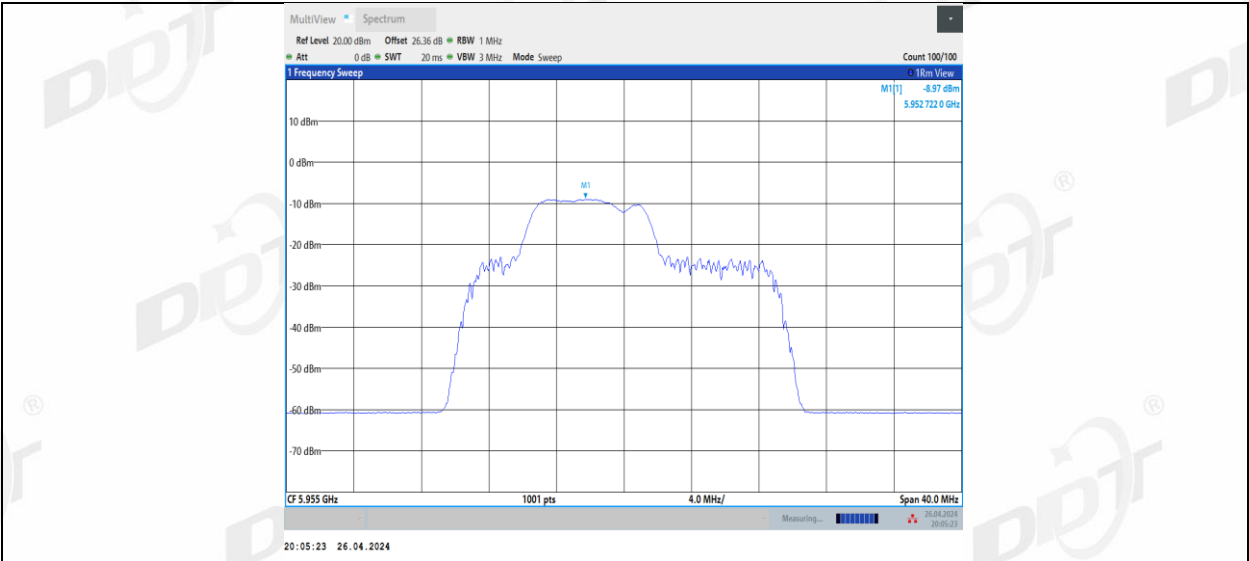
11BE20MIMO_Ant2_5955_52+26_3
