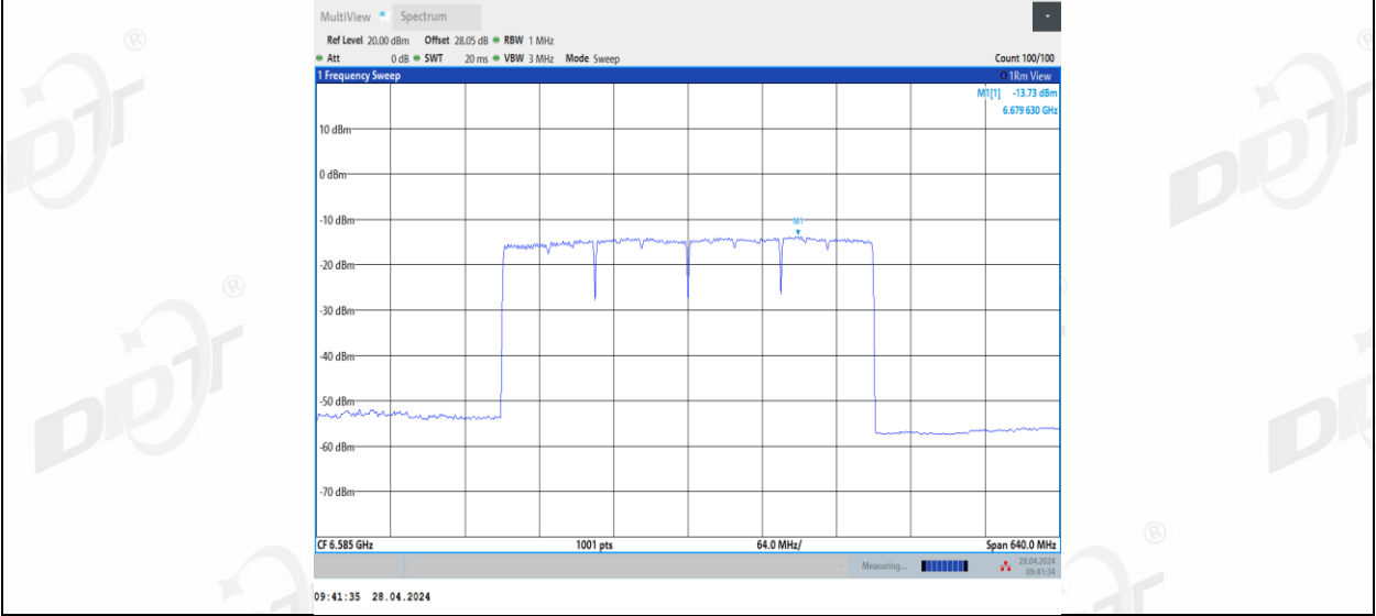
11BE320MIMO_Ant3_6585
