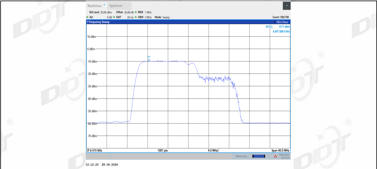
11BE20MIMO_Ant1_6415_106+26_2
