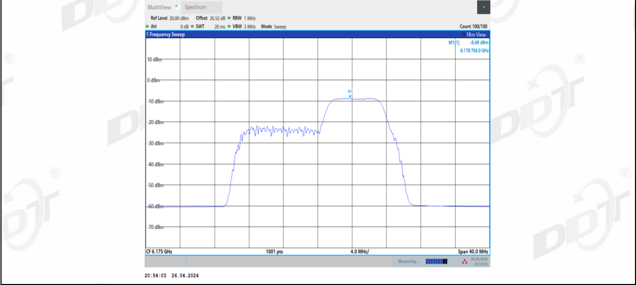
11BE20MIMO Ant1_6175_106+26_1
