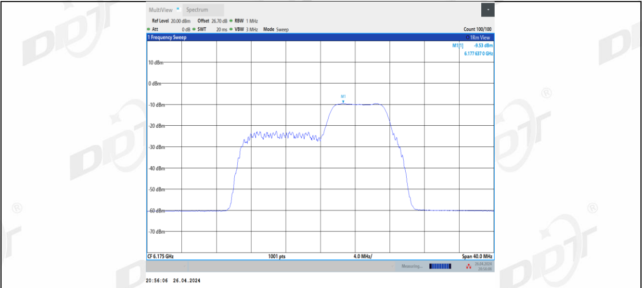
11BE20MIMO_Ant3_6175_106+26_1
