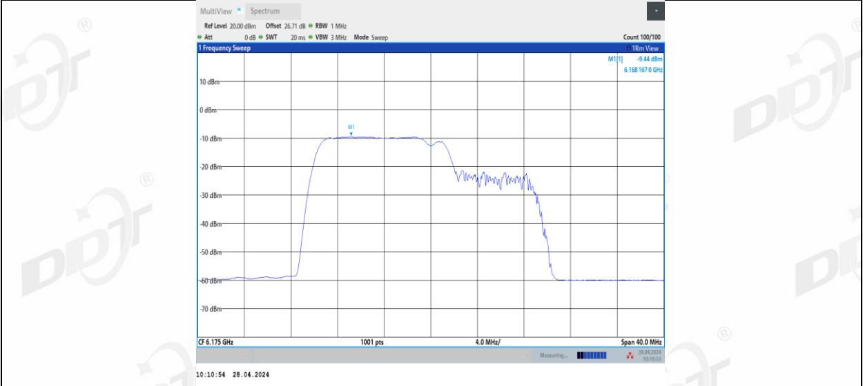
11BE20MIMO_Ant3_6175_106+26_2
