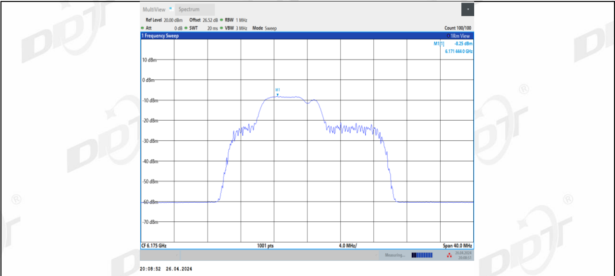
11BE20MIMO_Ant2_6175_52+26_3
