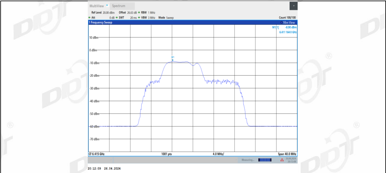
11BE20MIMO_Ant2_6415_52+26_3
