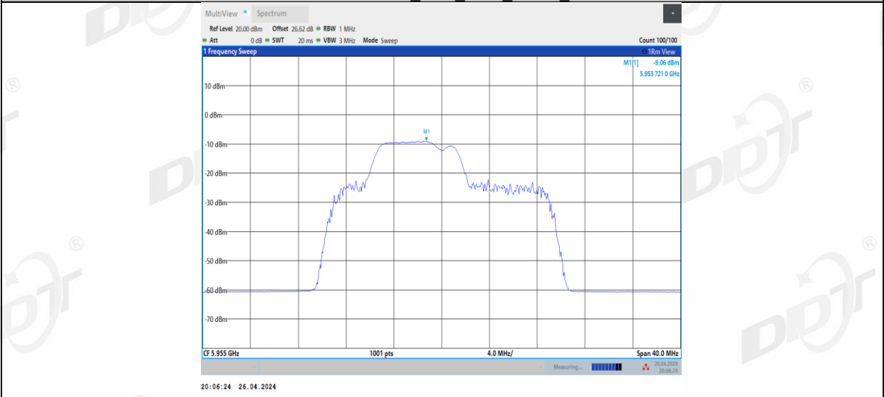
11BE20MIMO_Ant3_5955_52+26_3
