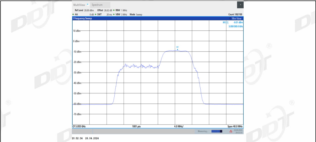
11BE20MIMO_Ant3_5955_106+26_1
