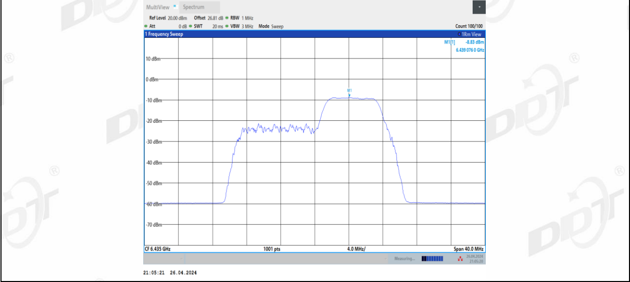
11BE20MIMO Ant1_6435_106+26_1
