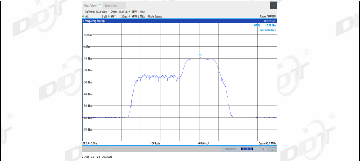
11BE20MIMO_Ant3_6415_106+26_1
