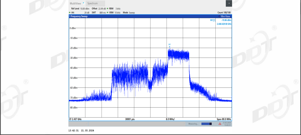
11BE40MIMO_Ant2_2437_106+26_OFDMA_3
