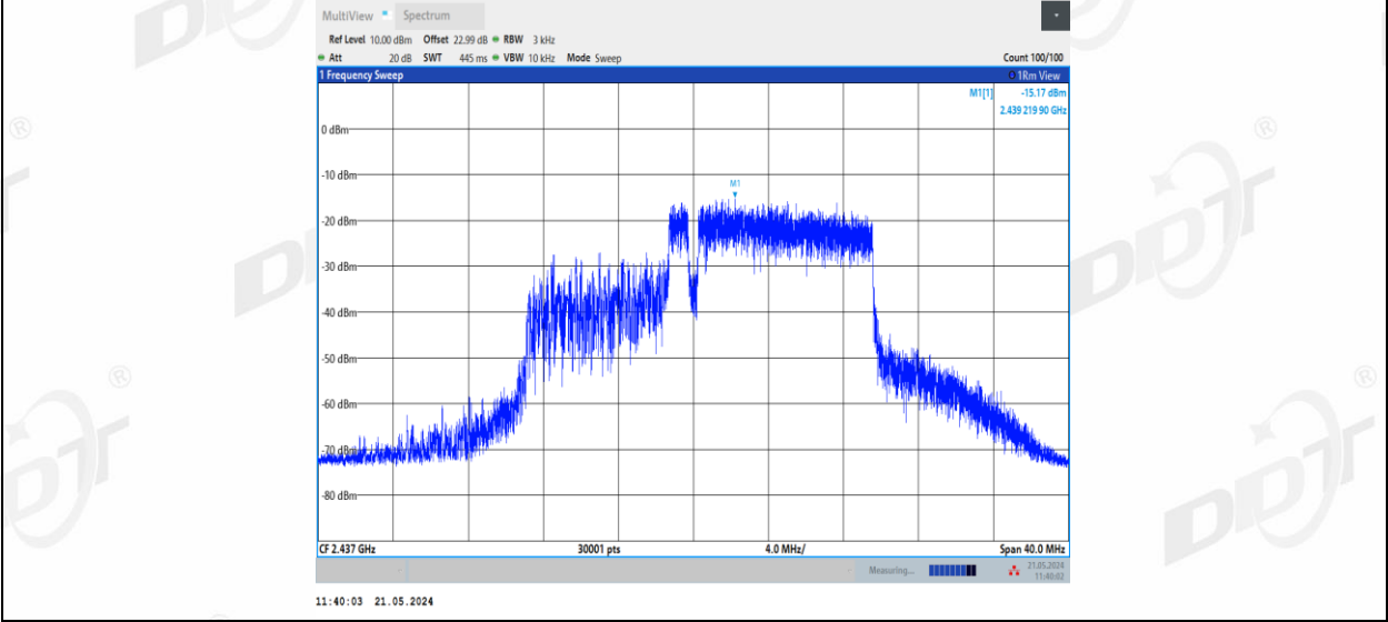
11BE20MIMO_Ant2_2437_52+26_OFDMA_1
