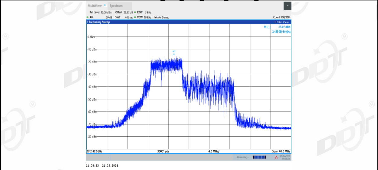
11BE20MIMO_Ant1_2462_52+26_OFDMA_2
