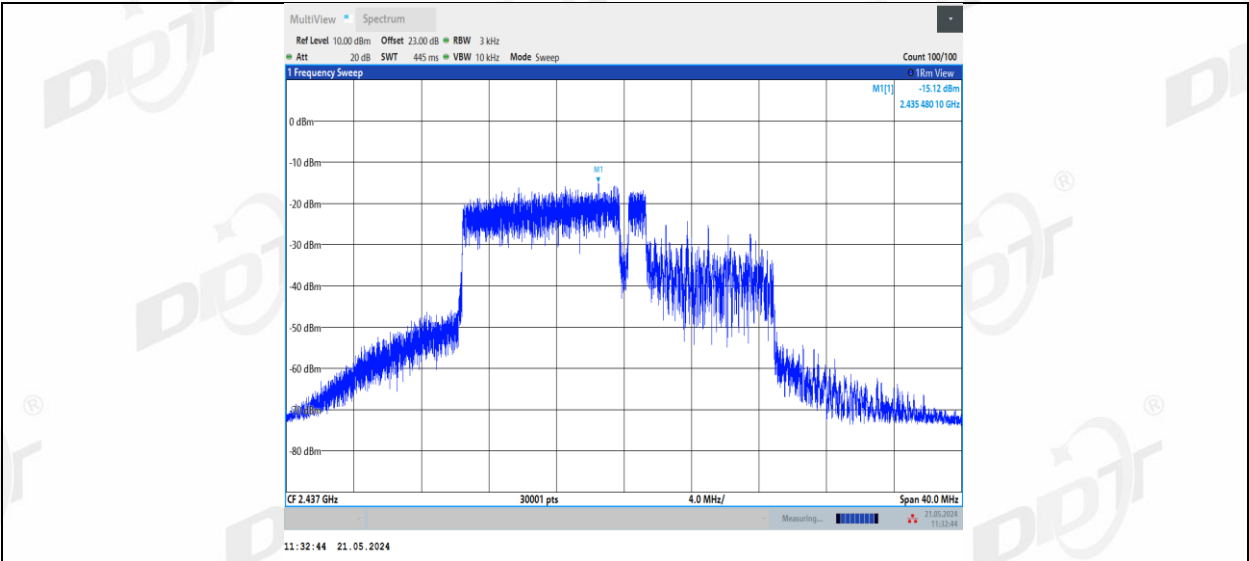
11BE20MIMO_Ant2_2437_106+26_OFDMA_2
