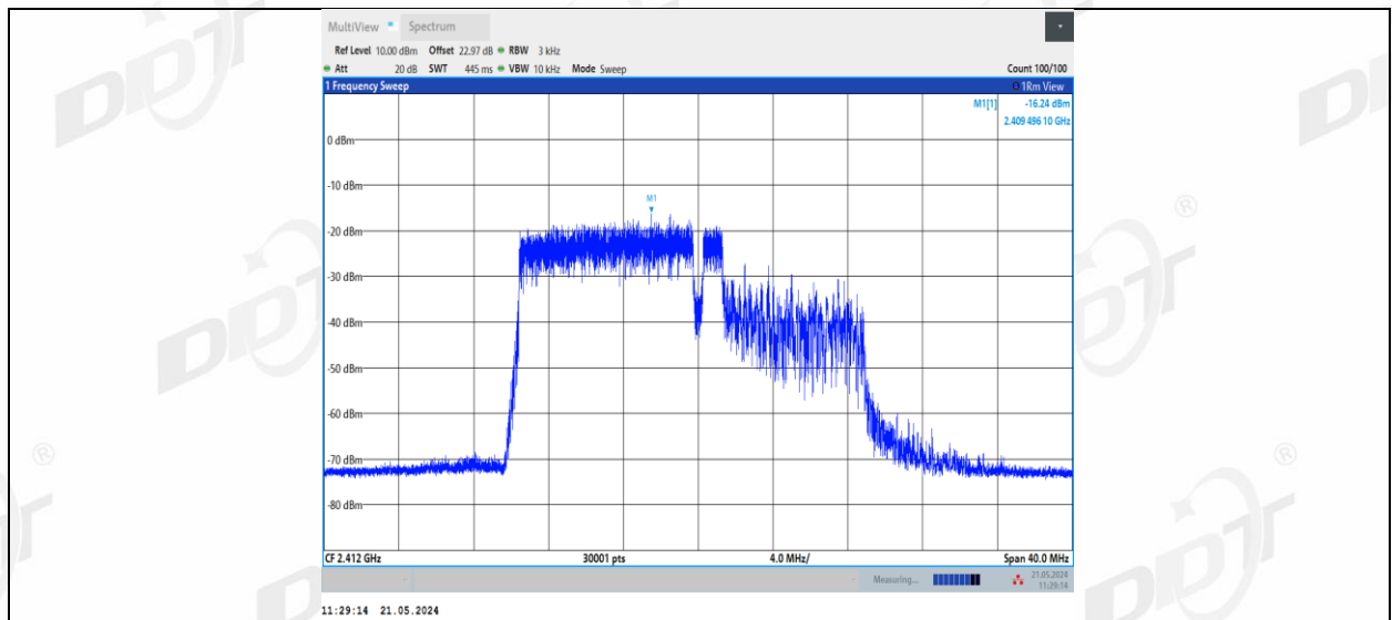
11BE20MIMO_Ant1_2412_106+26_OFDMA_2
