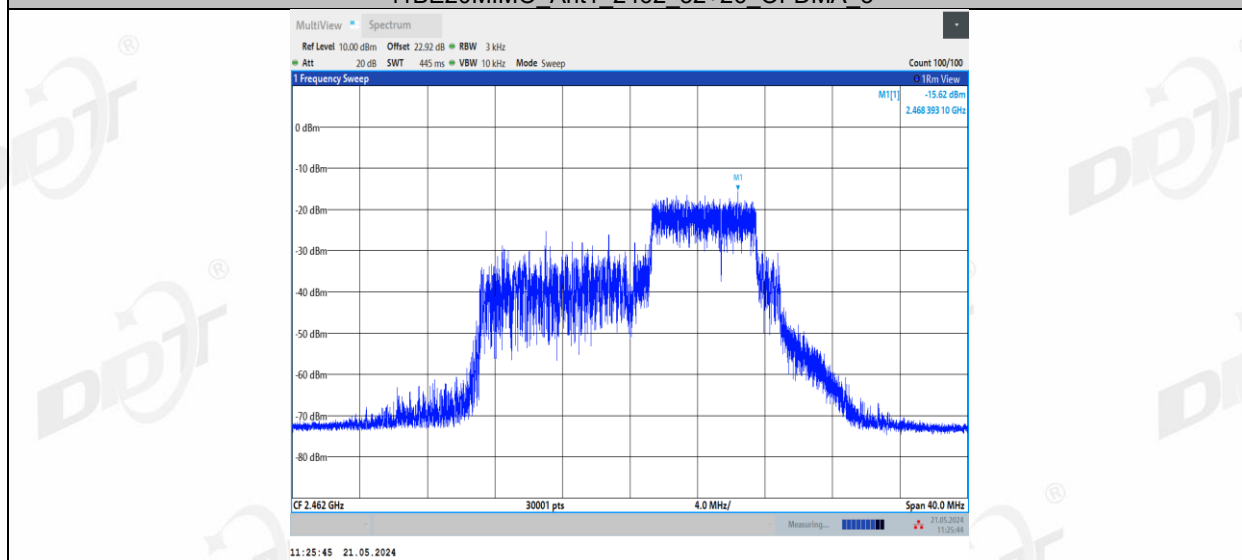
11BE20MIMO_Ant1_2462_106+26_OFDMA_1
