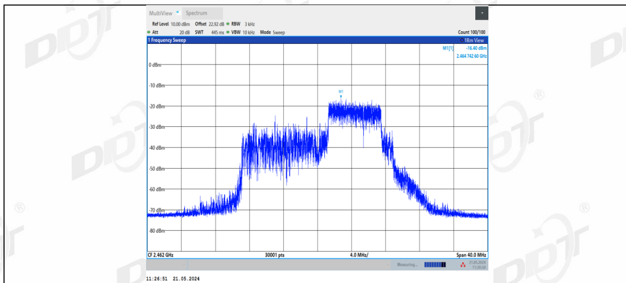
11BE20MIMO_Ant2_2462_106+26_OFDMA_1
