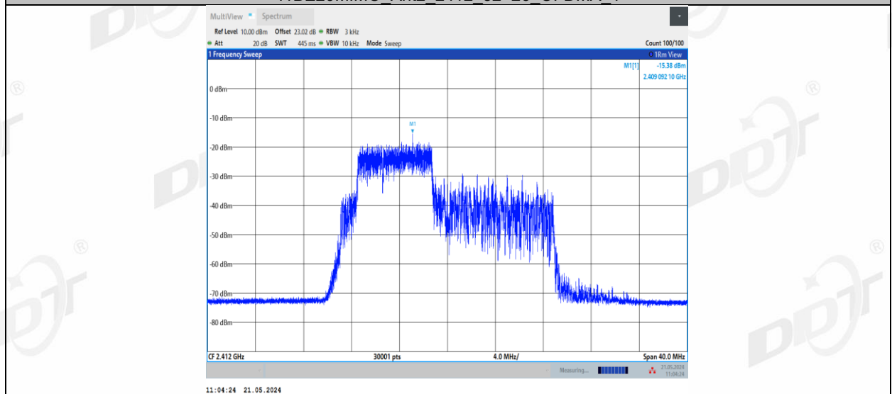
11BE20MIMO_Ant2_2412_52+26_OFDMA_2
