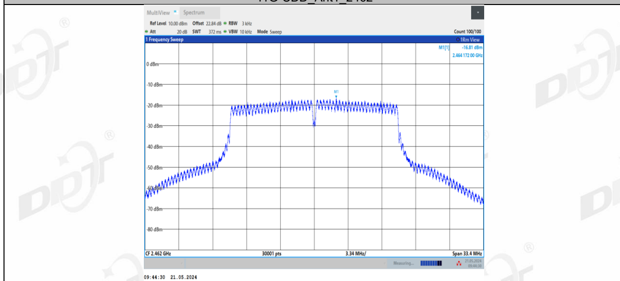
11G-CDD_Ant2_2462
