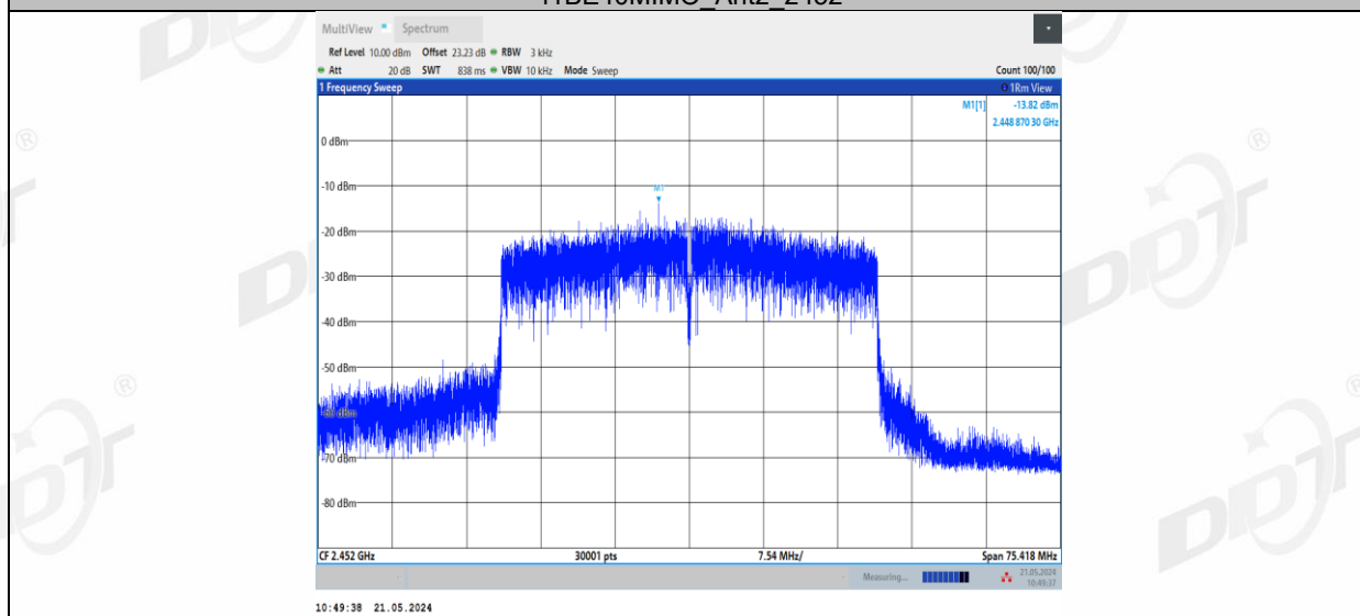
11BE40MIMO_Ant2_2452
