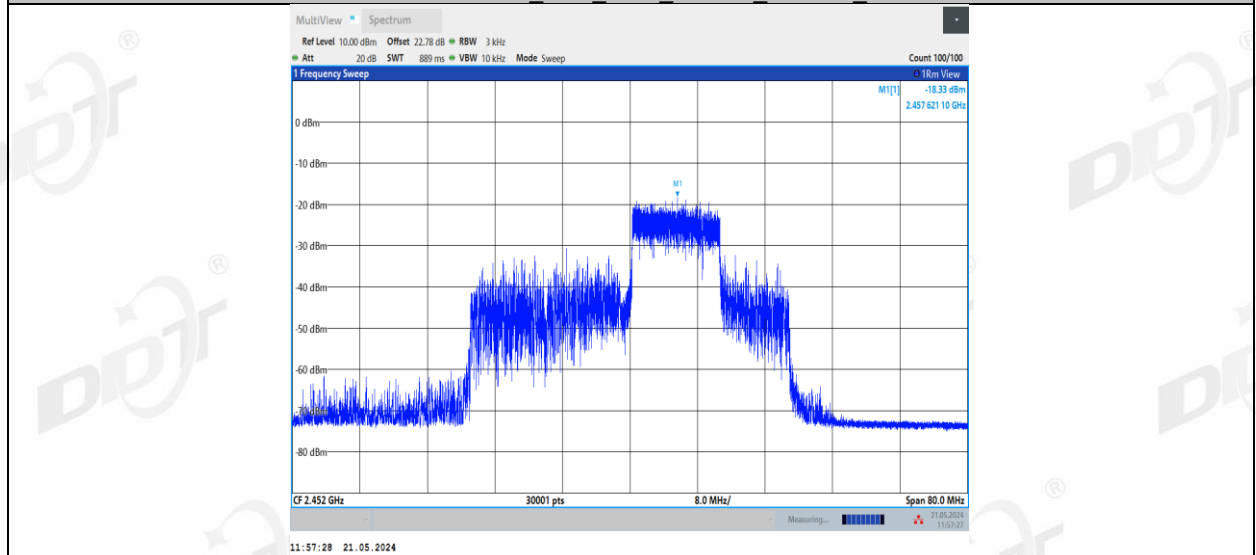
11BE40MIMO_Ant2_2452_106+26_OFDMA_4
