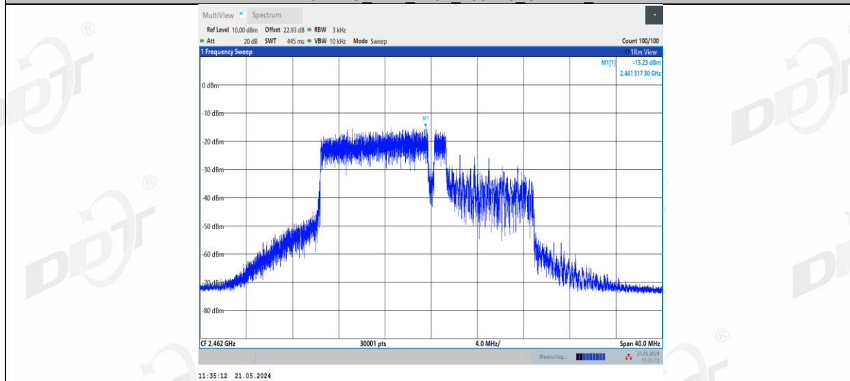
11BE20MIMO_Ant2_2462_106+26_OFDMA_2
