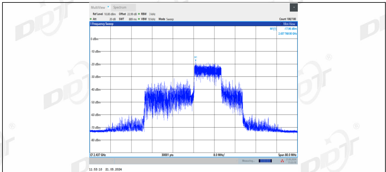
11BE40MIMO_Ant2_2437_106+26_OFDMA_4
