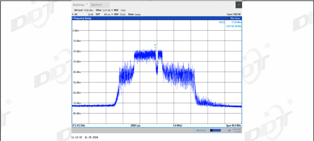
11BE20MIMO_Ant2_2412_52+26_OFDMA_3
