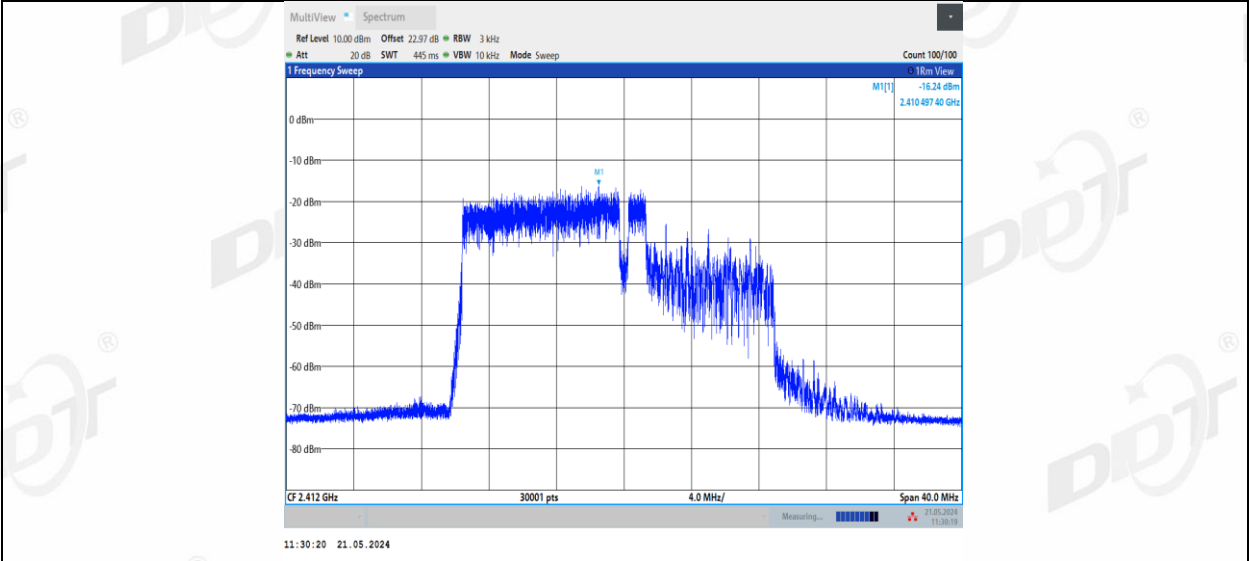
11BE20MIMO_Ant2_2412_106+26_OFDMA_2
