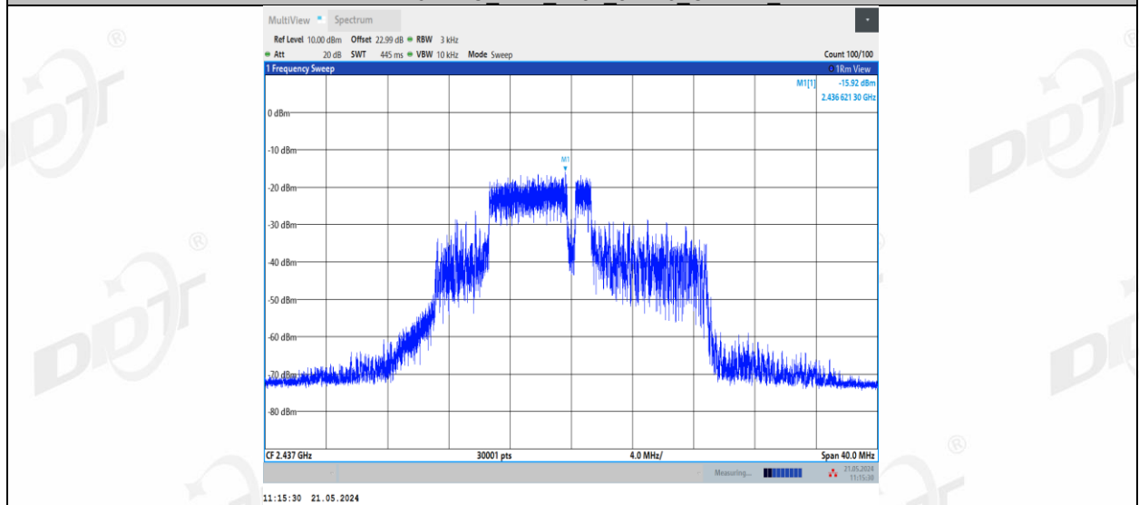
11BE20MIMO_Ant2_2437_52+26_OFDMA_3
