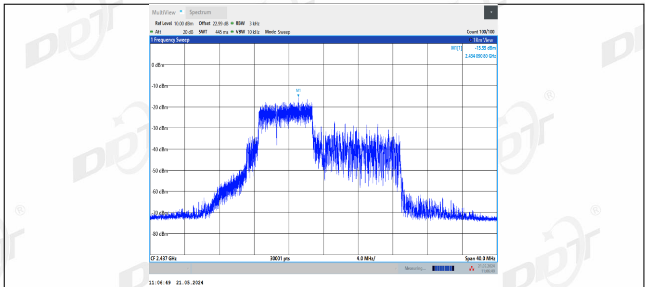
11BE20MIMO_Ant2_2437_52+26_OFDMA_2
