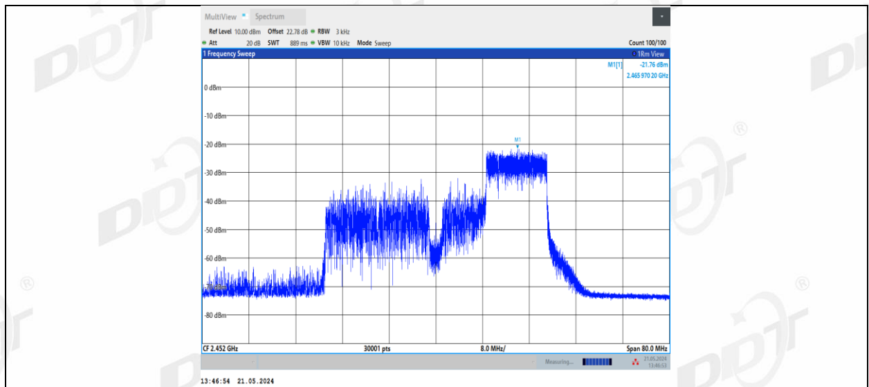
11BE40MIMO_Ant2_2452_106+26_OFDMA_3
