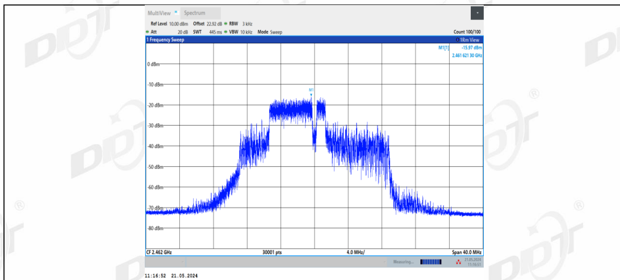
11BE20MIMO_Ant1_2462_52+26_OFDMA_3
