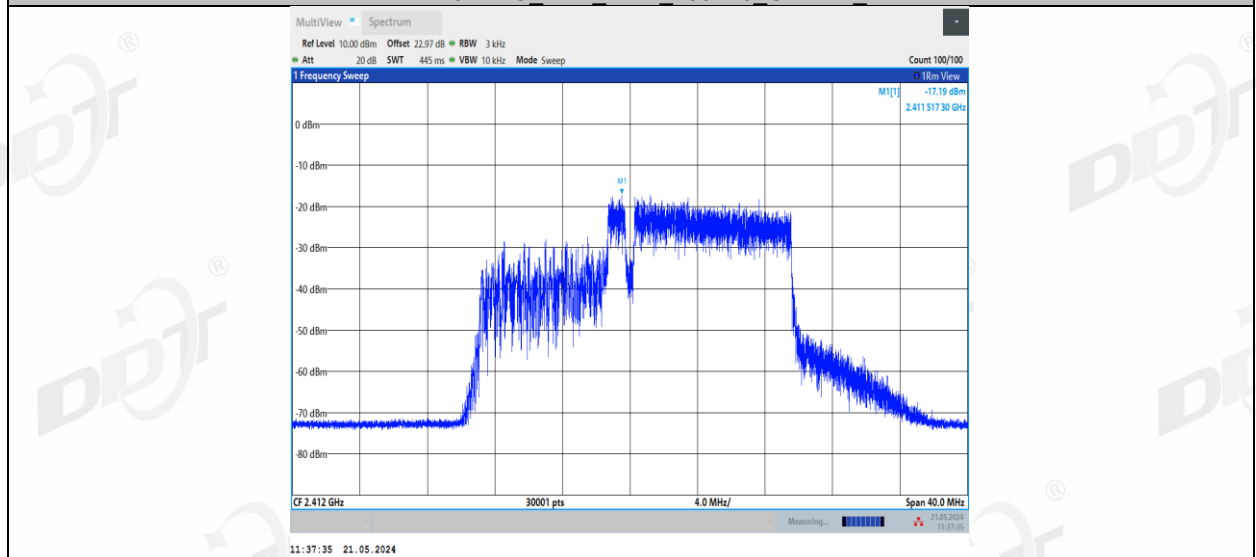
11BE20MIMO_Ant2_2412_52+26_OFDMA_1
