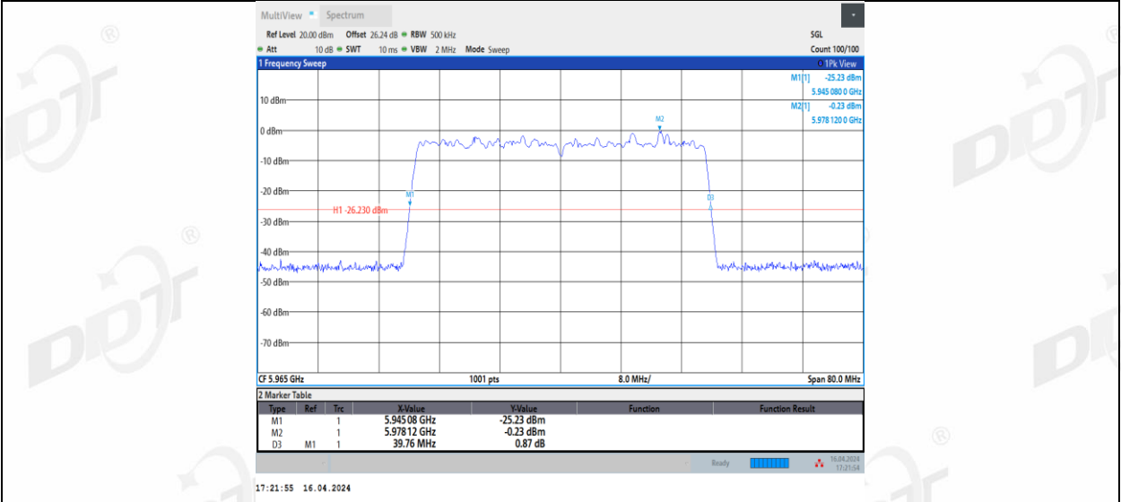
11BE40MIMO_Ant3_5965
