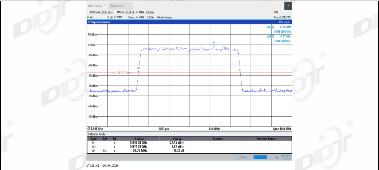
11BE40MIMO_Ant2_5965
