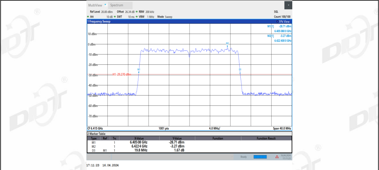
11BE20MIMO_Ant3_6415
