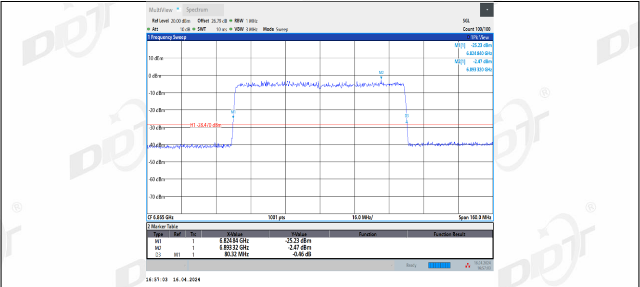
11AX80MIMO_Ant2_6865
