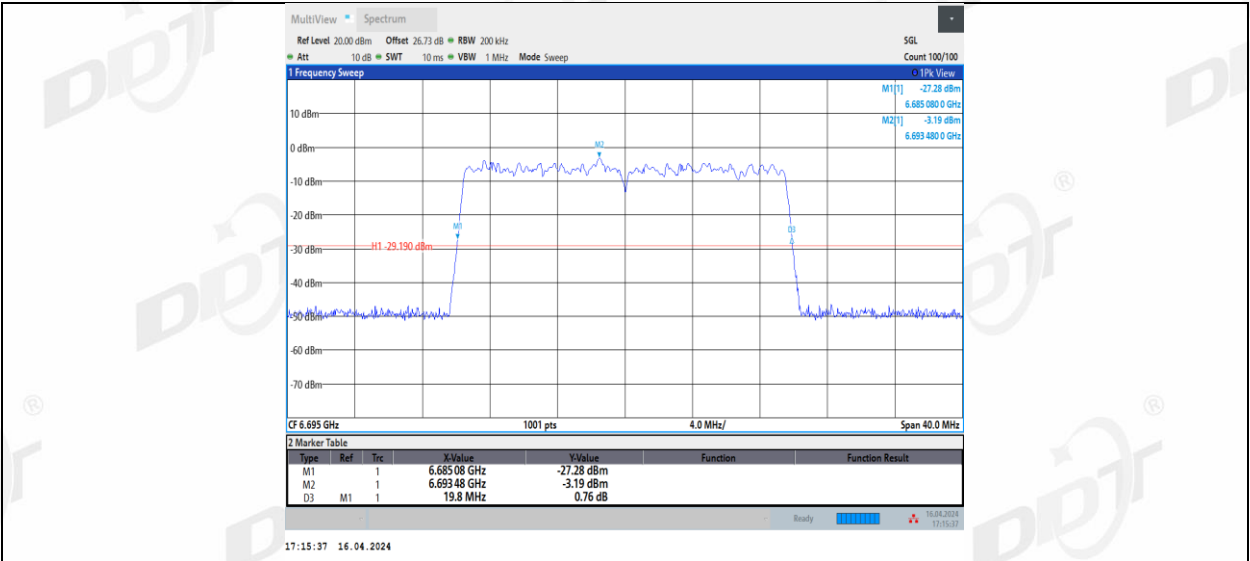
11BE20MIMO_Ant2_6695
