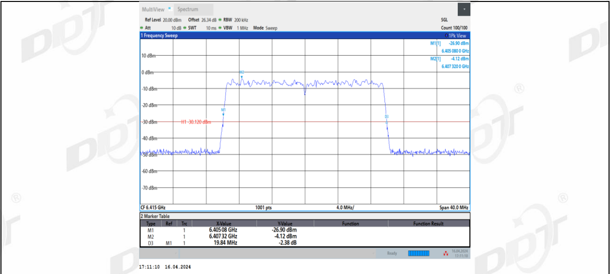
11BE20MIMO_Ant2_6415
