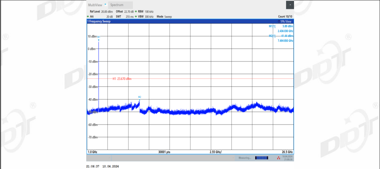
11BE20MIMO_Ant1_2462_0~Reference
