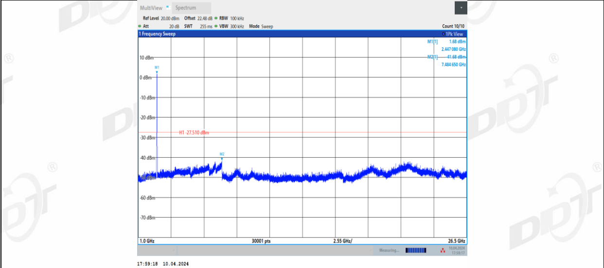
11AX20MIMO_Ant1_2412_0~Reference
