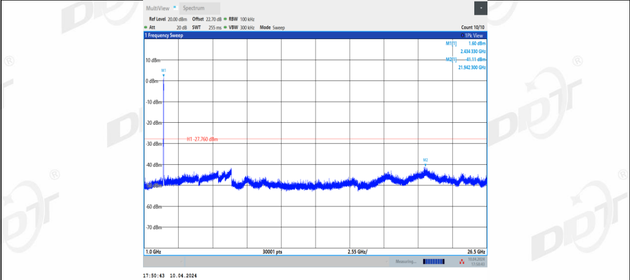
11N40MIMO_Ant1_2452_0~Reference
