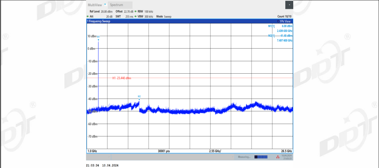
11BE20MIMO_Ant2_2437_0~Reference
