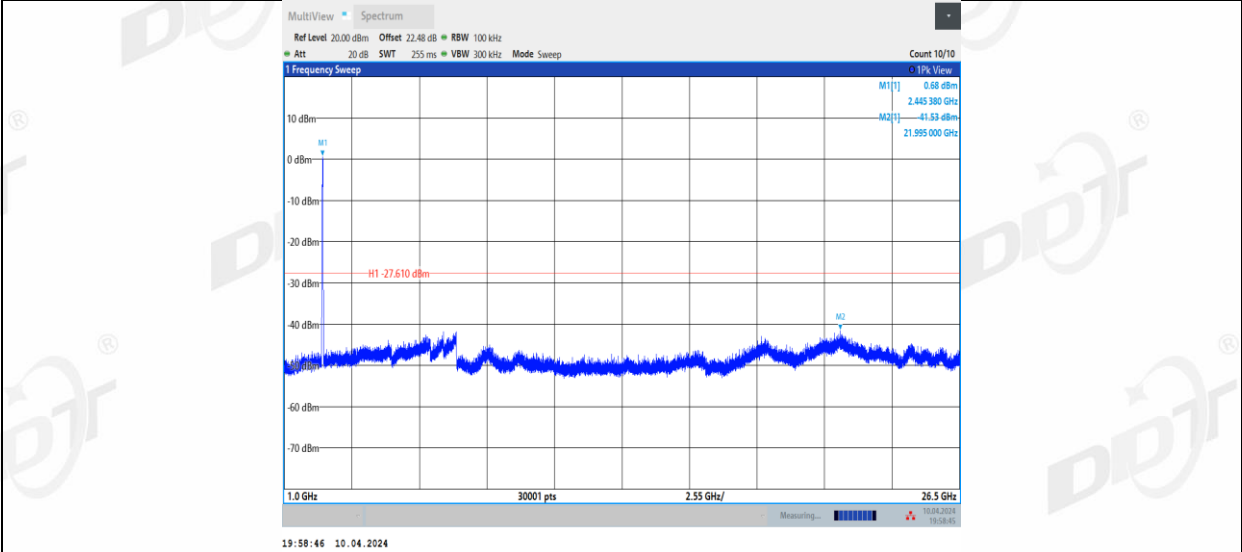
11BE20MIMO_Ant1_2412_0~Reference
