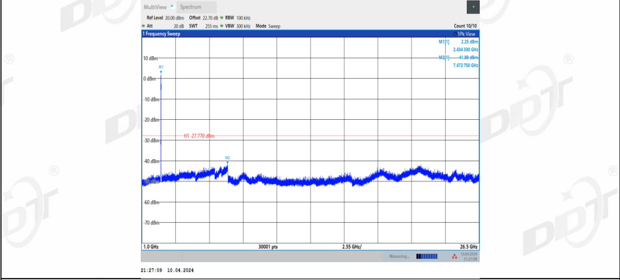
11BE40MIMO_Ant2_2437_0~Reference
