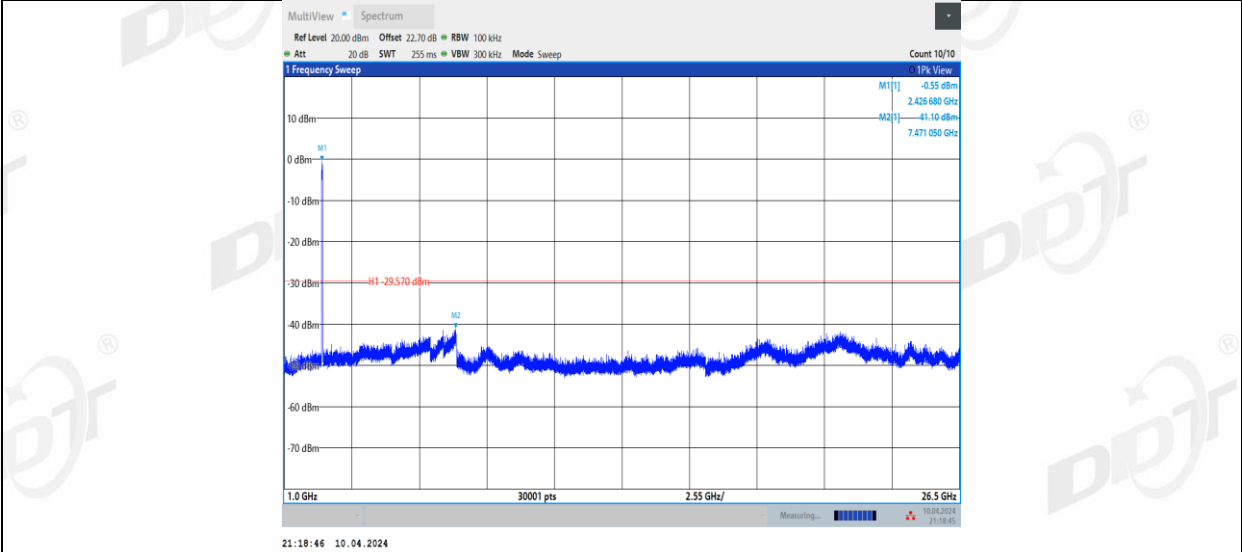
11BE40MIMO_Ant2_2422_0~Reference
