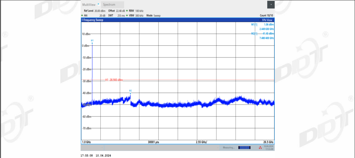
11N40MIMO_Ant2_2452_0~Reference
