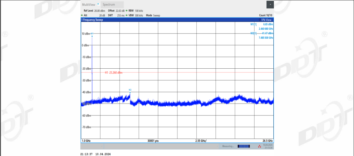
11BE40MIMO_Ant1_2422_0~Reference
