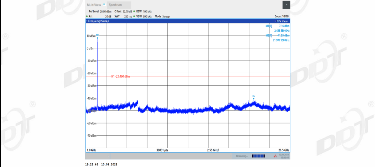
11AX20MIMO_Ant2_2437_0~Reference
