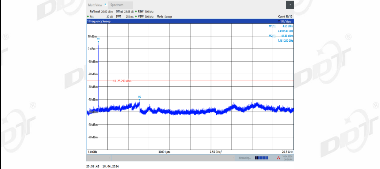
11BE20MIMO_Ant2_2412_0~Reference
