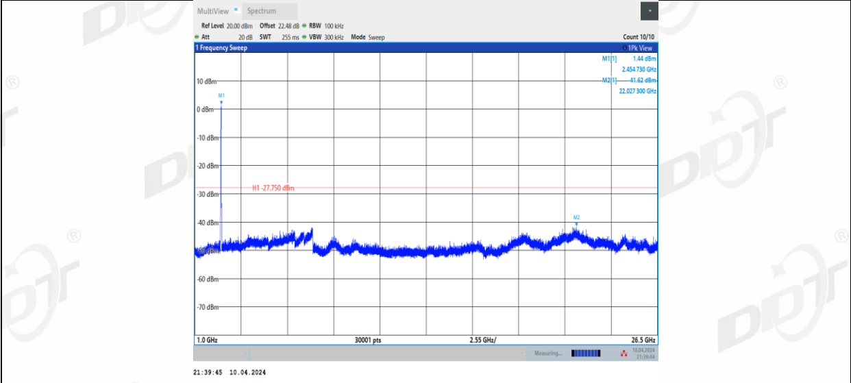
11BE40MIMO_Ant2_2452_1000~26500
