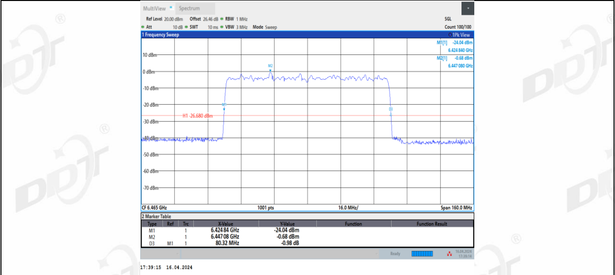
11BE80MIMO_Ant3_6465
