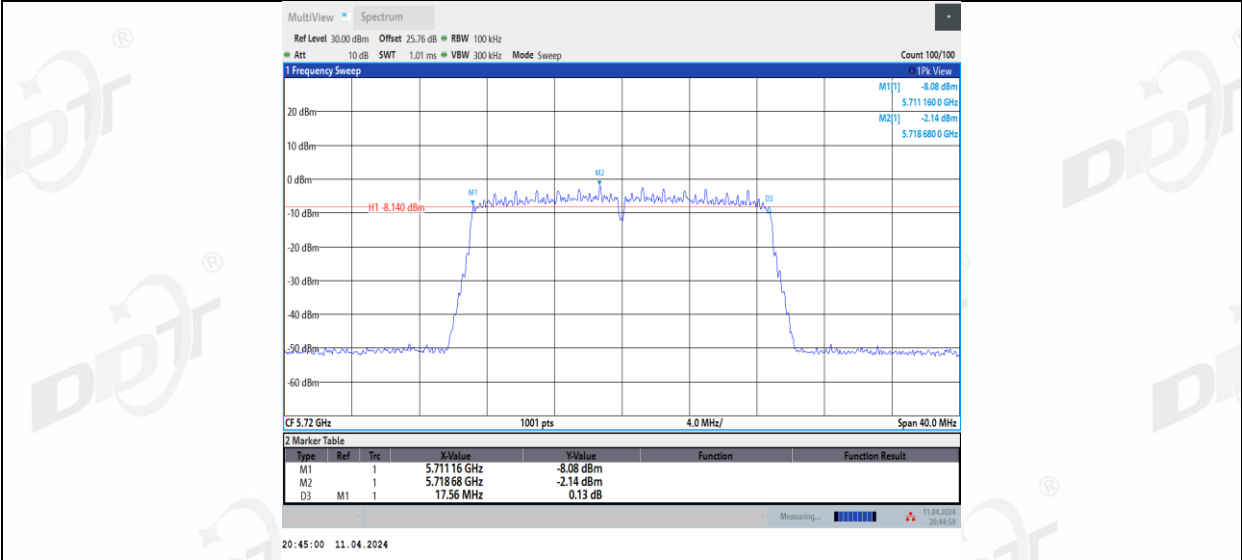
11N20MIMO_Ant3_5720
