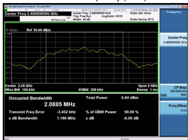
BLE 2M Carrier frequency (MHz): 2480
