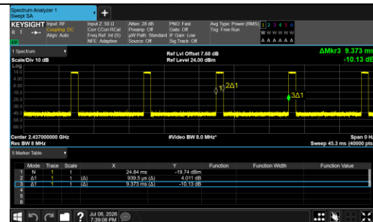
IEEE 802.11b 20MHz Channel 6
