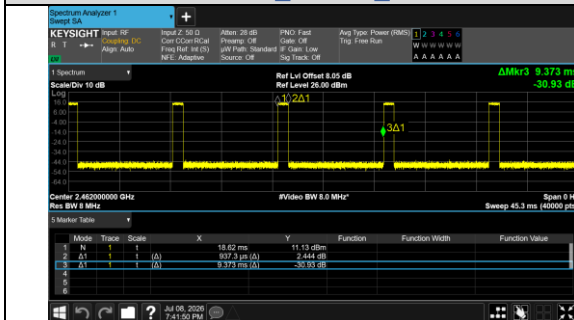
IEEE 802.11b 20MHz Channel 11
