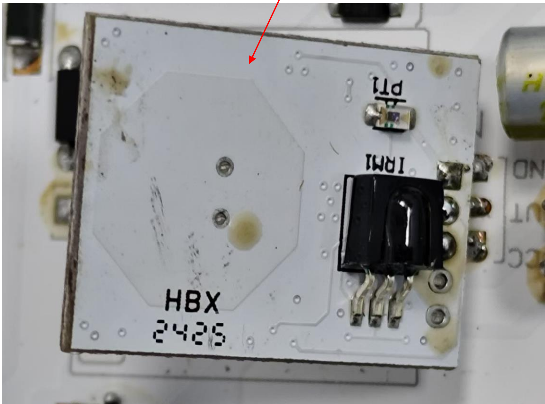
Antenna
