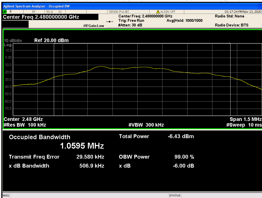
-6dB Bandwidth NVNT BLE 1M PHY 2480MHz Ant1
