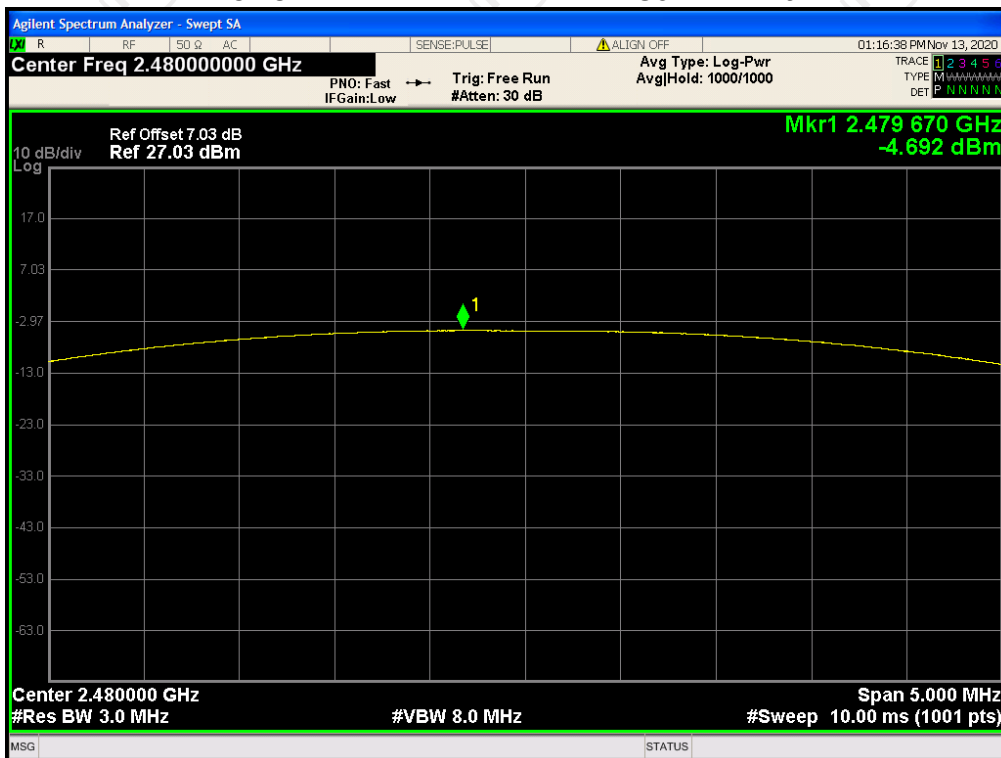
Power NVNT BLE 1M PHY 2480MHz Ant1
